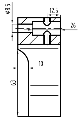
A-A metszet
