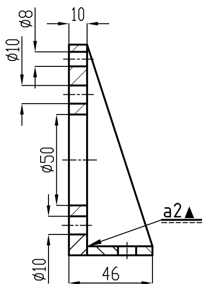
A-A metszet
