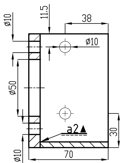
A-A metszet
