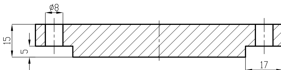
A-A metszet
