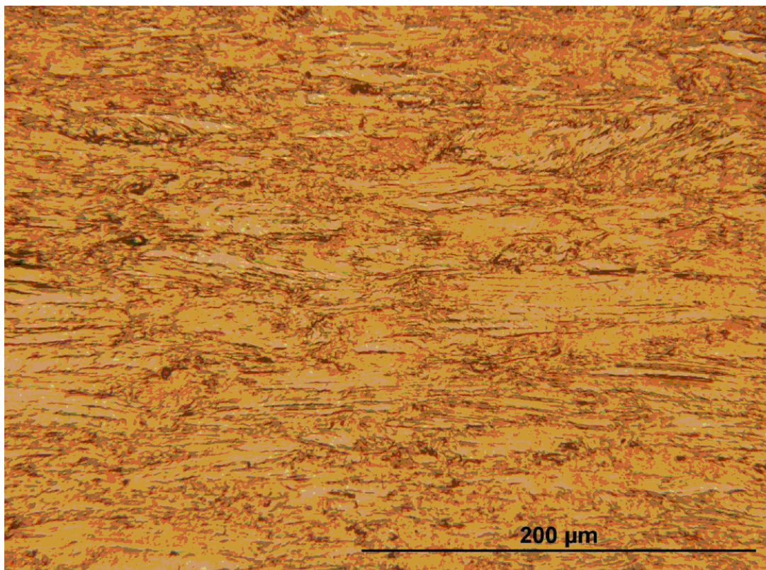
M7.ábra. A hidegen hengerelt, 90°C-on megszakított felhevítésű réz próbatest metallográfiai csiszolata
