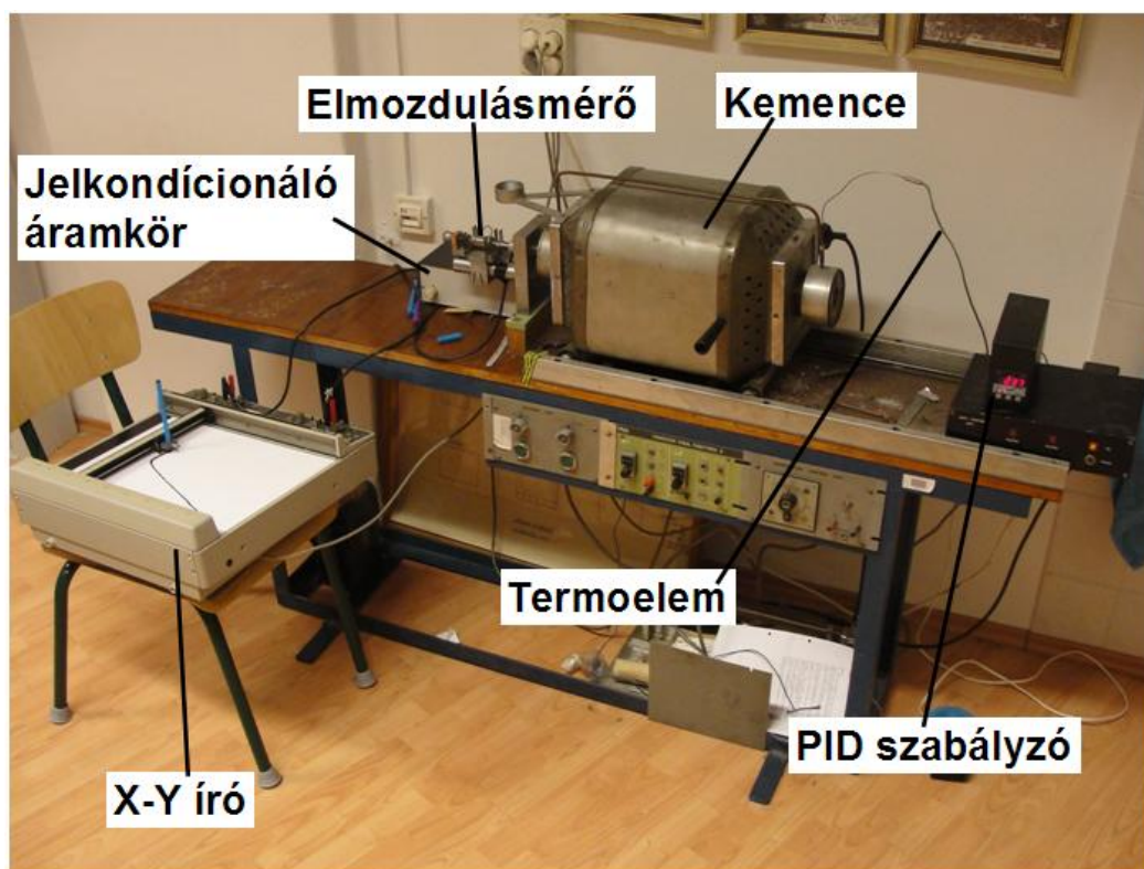
M1. ábra. A folyamatos keménységmérő berendezés fotója
