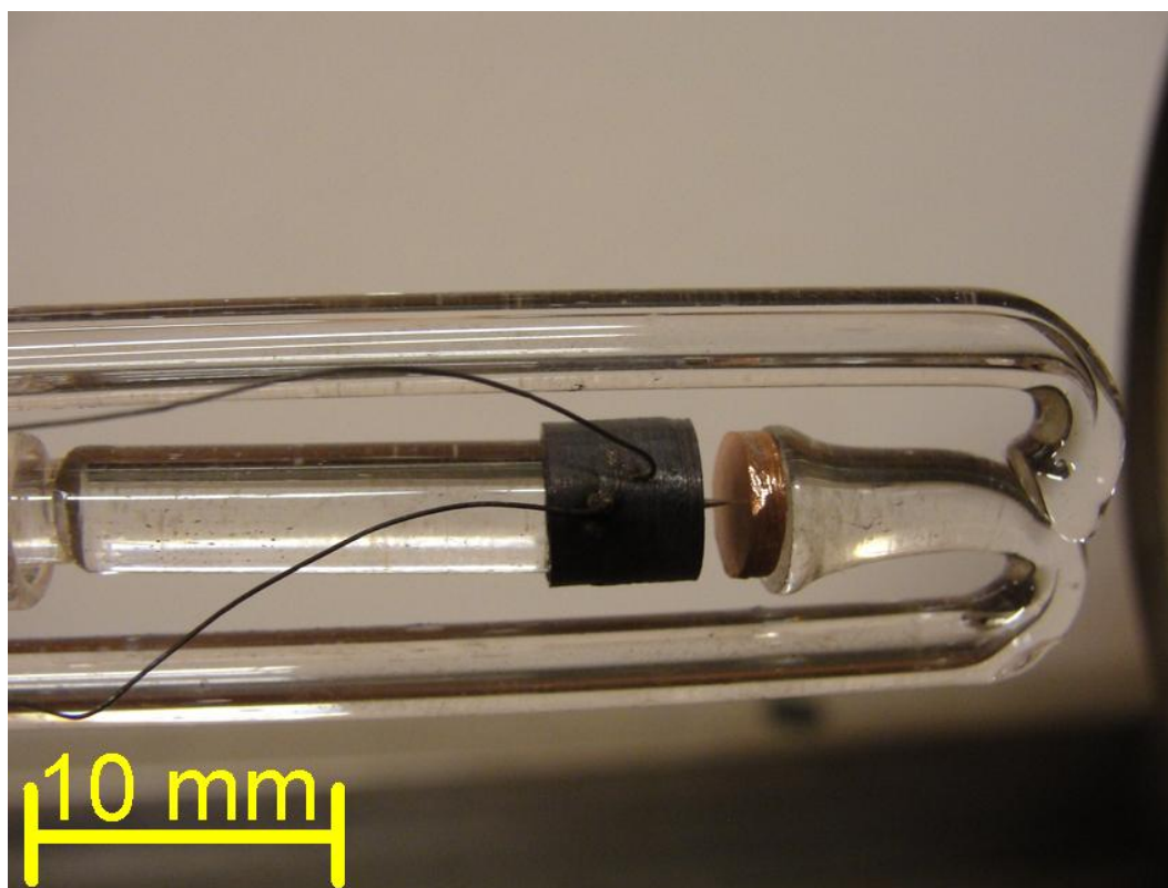
M2. ábra. Az acél tű és a réz próbatest az átalakított dilatometerben.
