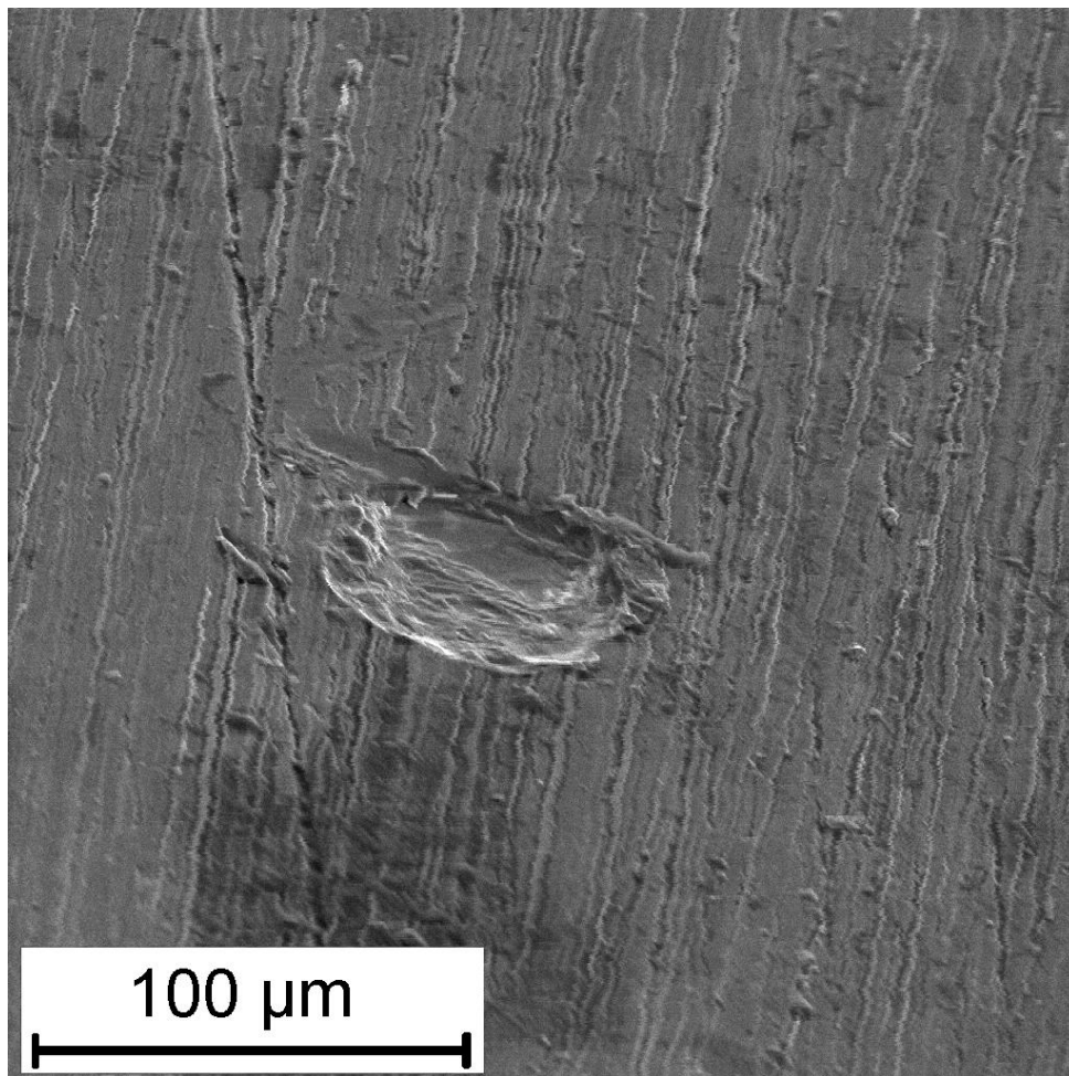
M3.ábra Az acél tű lenyomatának elektronmikroszkópos képe
