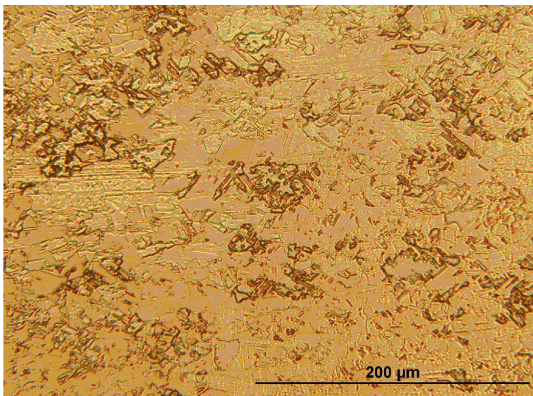
M8.ábra. A hidegen hengerelt, 180 °C-on megszakított felhevítésű réz próbatest metallográfiai csiszolata.
