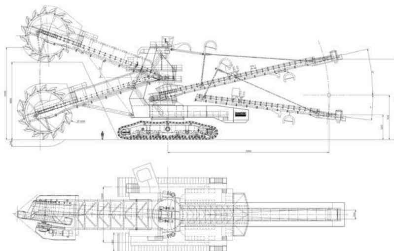
21. ábra Sandvik PE 100-as műszaki rajza (2013.10.19.), Forrás: www.mert.hu [36]
