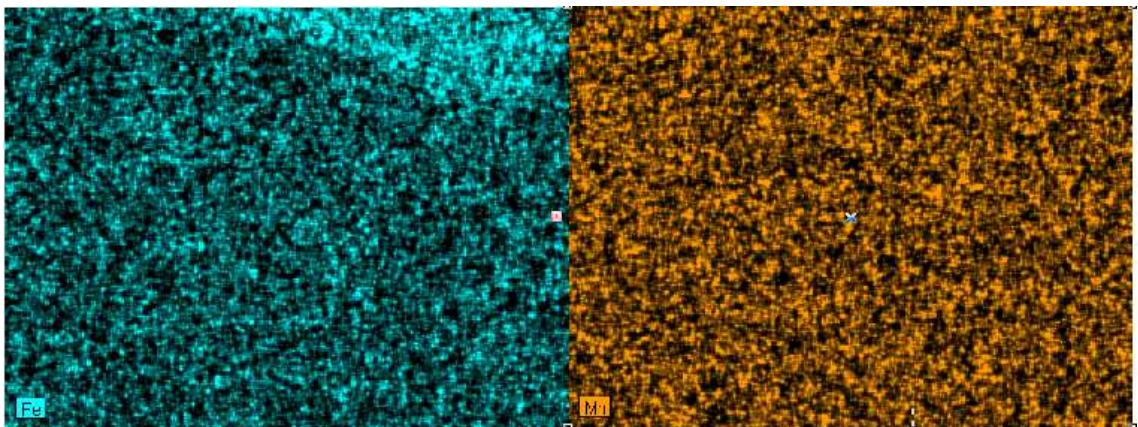
9.kép A vas (bal oldal) és a mangán (jobb oldal) eloszlásáról készült elemtérképek.
