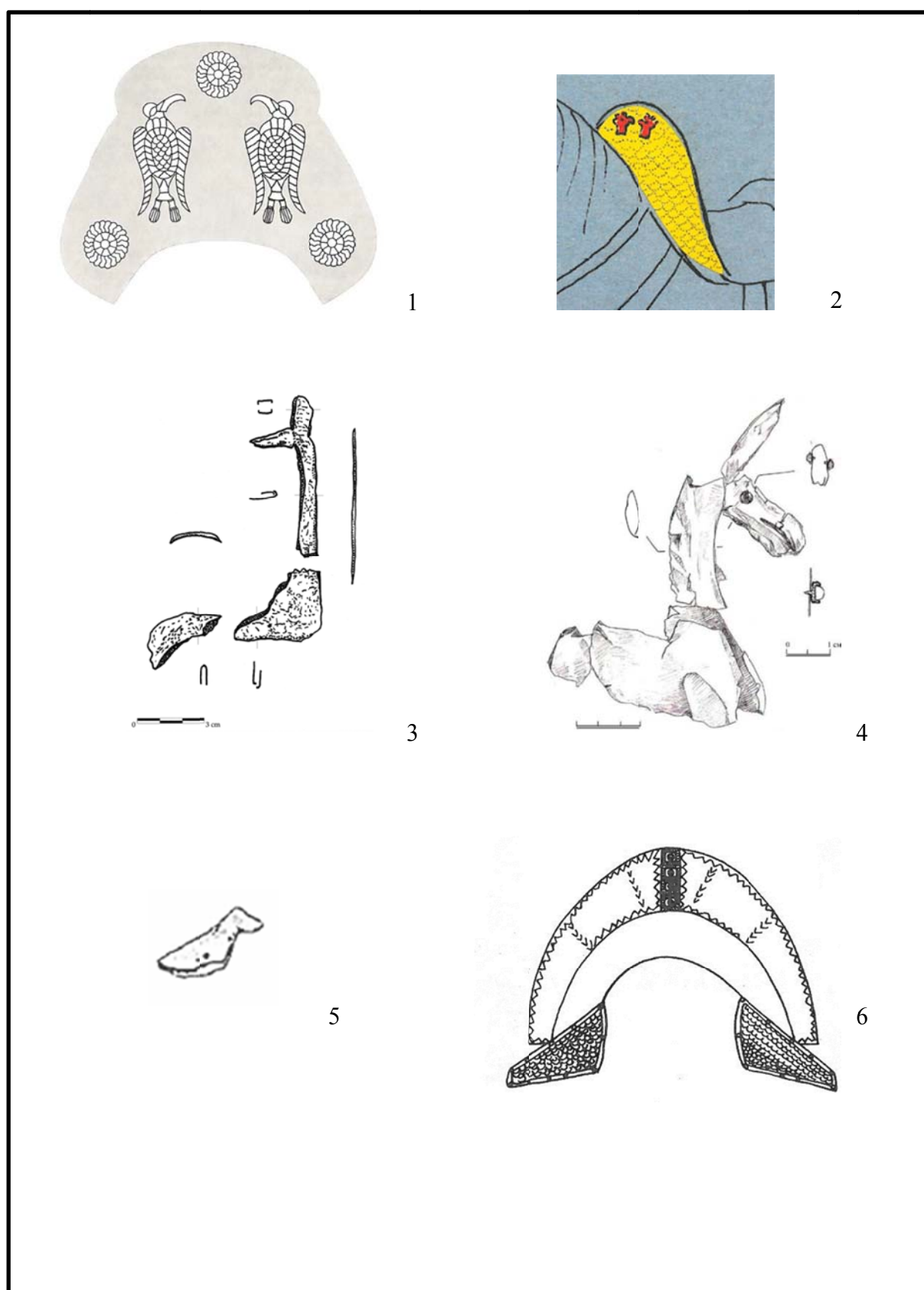
II. Tábla. 1–2, 6 Nyeregrekonstrukció (Apahida, Nagyszéksós, Melitopol), 3–5 Aranyfóliás szobor (Árpás, Ust'-Al'ma 957. sír, Kzyl-Kajnar-Tobe).
