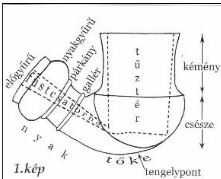
22. kép: a pipa fő részei Kondorosy Szabolcs ábráján (KONDOROSY 2008, 357).
