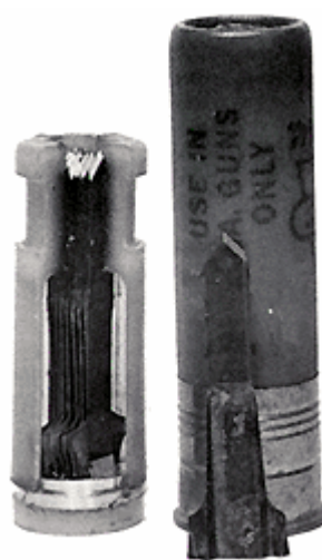
16. ábra Sörétes lőszer nyíllövedékekkel
