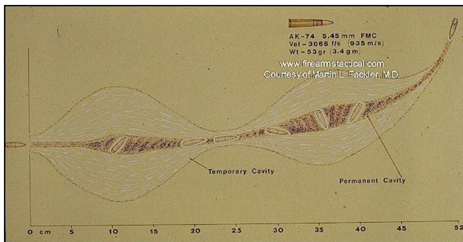
9. ábra 5,45×39 mm-es PS ballisztikai zselés tesztje
