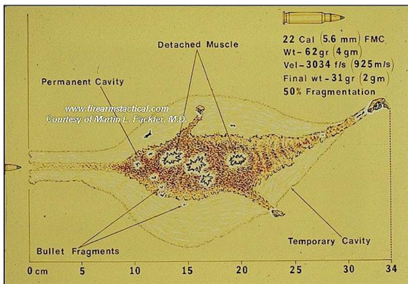
11. ábra 5,56×45 mm-es M855 ballisztikai zselés tesztje
