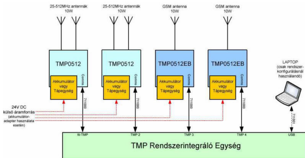
9. kép: TMP rendszer felépítése
