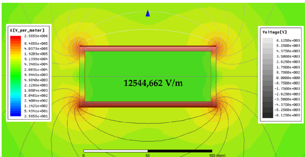
7. ábra. A térerő eloszlása a penészes tápoldattal töltött reaktorban ( \sigma=4,75\text{mS/cm} , \varepsilon=750 , U_{\text{eff}}=7000\text{V} , f=50\text{Hz} )
