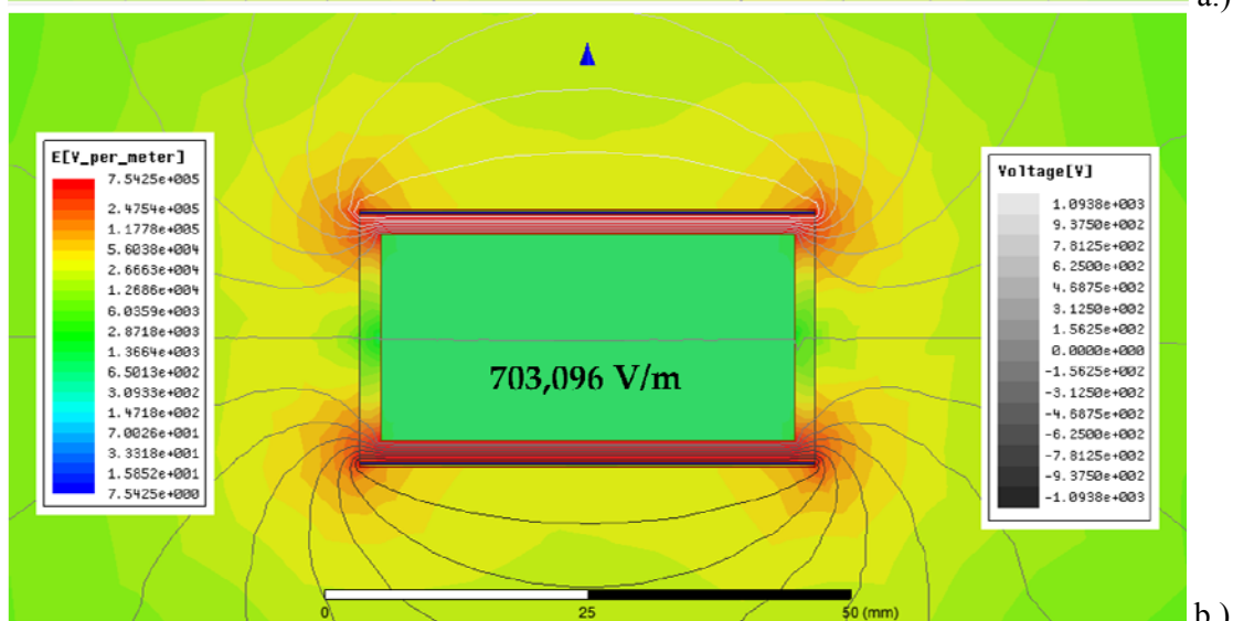
6. ábra. A térerő eloszlása a szuszpenzióval töltött reaktorban a szuszpenzió permittivitásának függvényében ( \sigma=175\mu\text{S/cm} , \varepsilon=500 (a.) és 3000 (b.), U=1250\text{V} )
