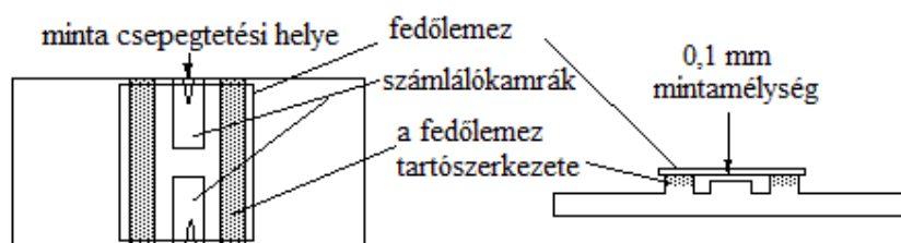
10. ábra. Számlálókamra felül- és oldalnézete [15]
