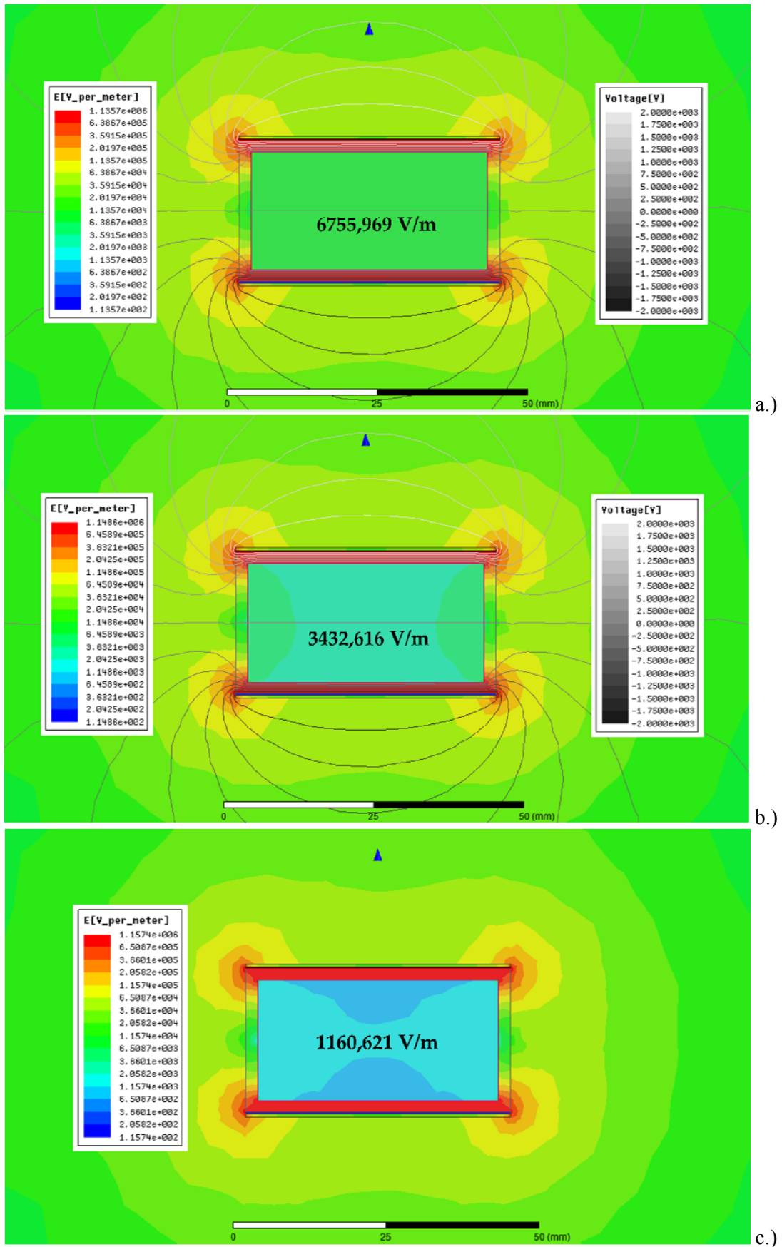
5. ábra. A térerő eloszlása a szuszpenzióval töltött reaktorban a szuszpenzió permittivitásának függvényében ( \sigma=175\mu\text{S/cm} , \varepsilon=500 (a.), 1000 (b.) és 3000 (c.), U_{\text{eff}}=2000\text{V} , f=50\text{Hz} )
