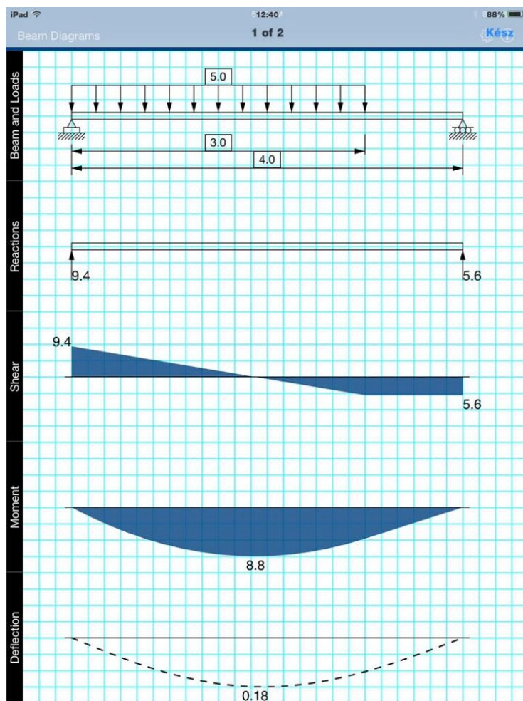
11. ábra: Tartó egy szakaszán megoszló erővel terhelt kéttámaszú tartó igénybevételi ábrái (bal oldalon) illetve egy koncentrált erővel terhelt konzolos tartó igénybevételi ábrái - iBeams nevű Apple Alkalmazás -[forrás: Apple iPad]
