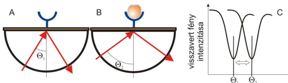
10. ábra – Az arany felületre immobilizált felismerő molekula \Theta_1 szög alatt idéző teljes visszaverődést a szenzor felületén (A). Az analát molekula bekötődése során a rezonanciaszög \Theta_2 -re változik (B), így a rezonancia szög eltolódásán keresztül (C) a bekötődés érzékenyen nyomon követhető [67].
