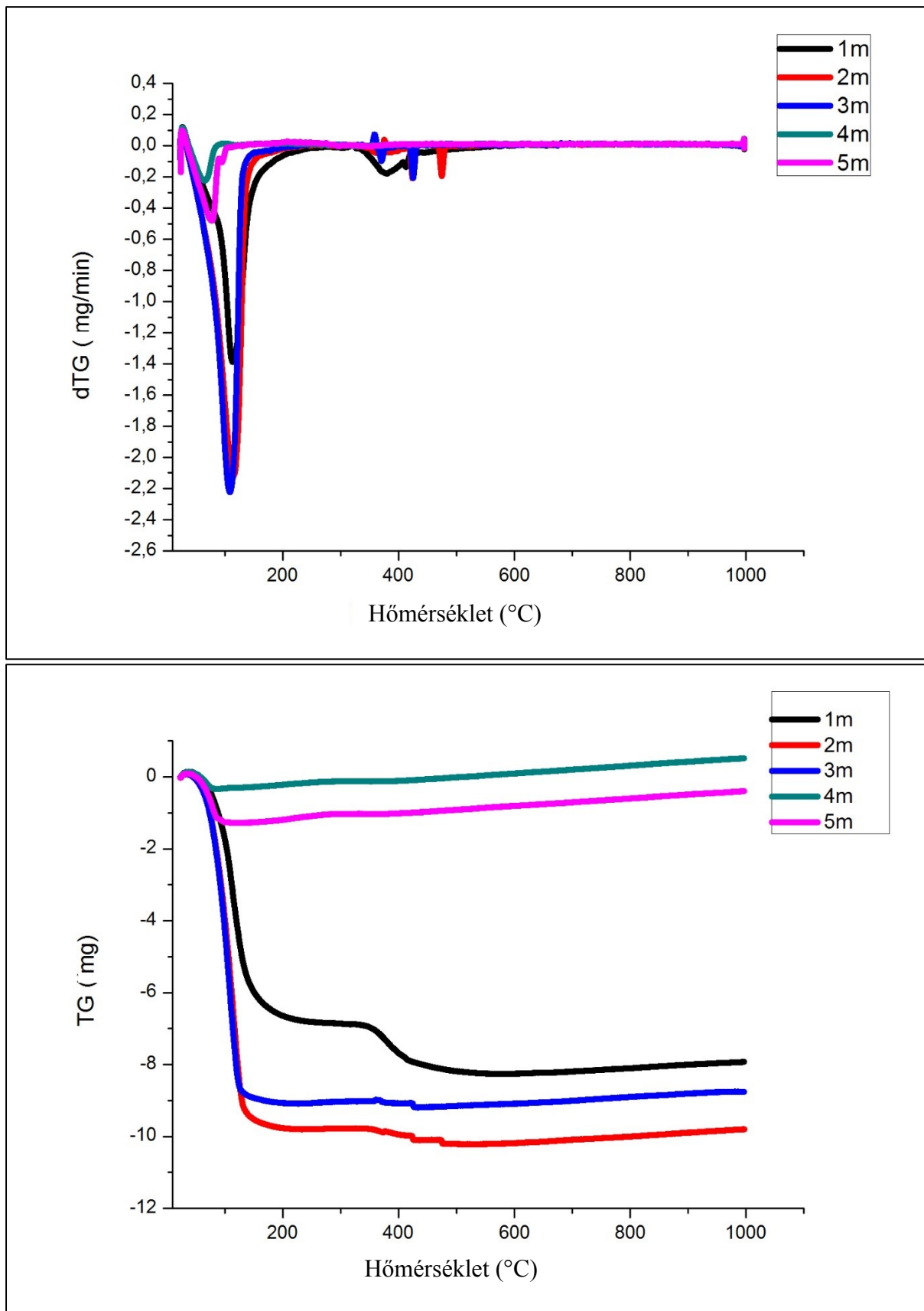
10. ábra A vízbázisú fekecs dTG (fent) és TG (lent) vizsgálatának eredménye, a két ábrán használt színkódolás megegyezik
