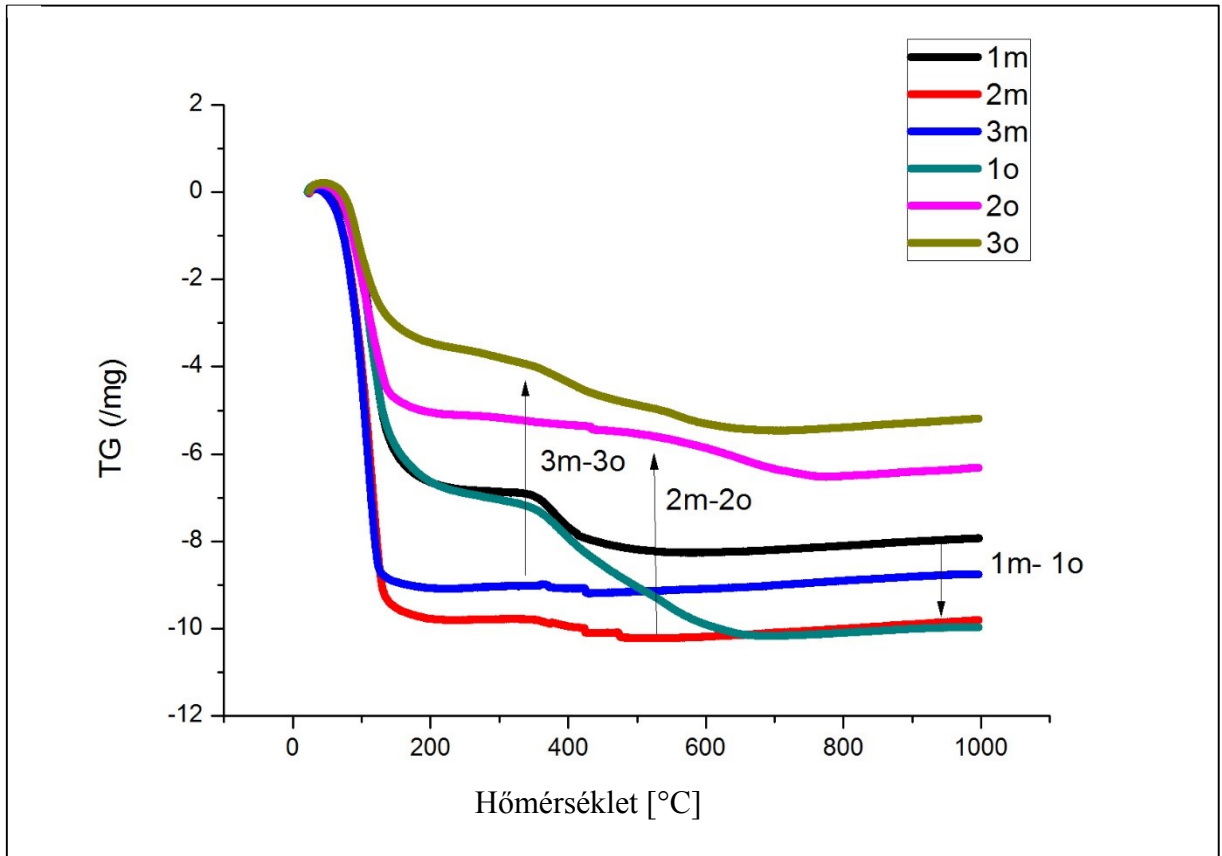
12. ábra Az m- és o-jelű minták termogravimetriai görbéjének összehasonlítása. A nyilak a nátrium-szilikát tartalmú minták felé mutatnak.
