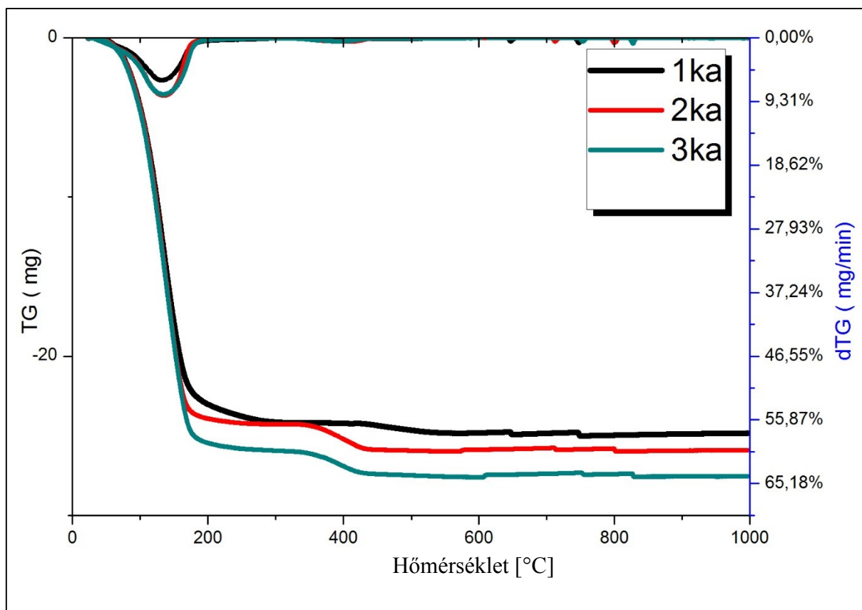
9. ábra A vízbázisú mintasorozathoz használt magnézia-cement kötőanyag termogravimetriai vizsgálata, ahol az azonos színű vonalak azonos anyagot jelölnek.
