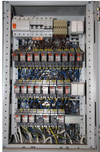
2. ábra – nagybátyám összetett relés vezérlése
