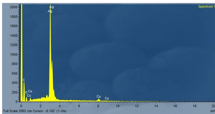
6. kép: A Letkés A fibula ezüsttartalmára vonatkozó scanning elektronkép és spektrum
