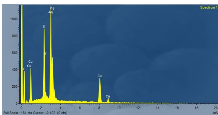
8. kép: A Letkés A fibula nielló berakására vonatkozó scanning elektronkép és spektrum
