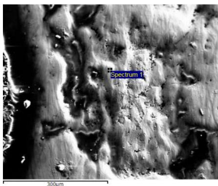
6. kép: A Letkés A fibula ezüsttartalmára vonatkozó scanning elektronkép és spektrum
