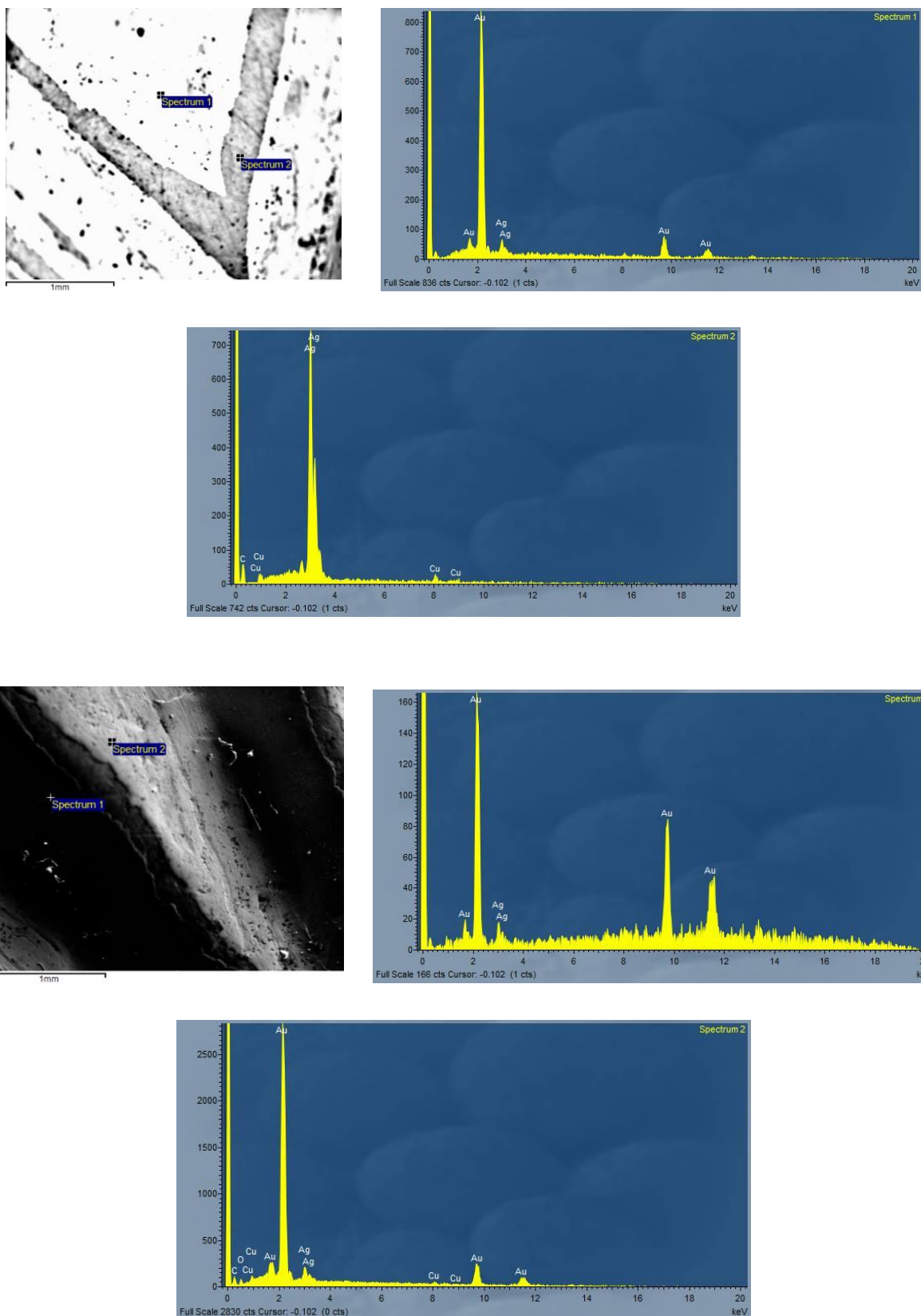
5. kép: A Bakodpuszta B fibula aranyozására vonatkozó scanning elektronképei és spektrumai
