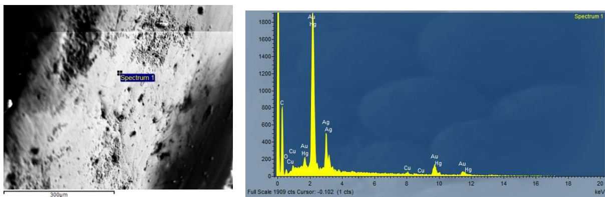
10. kép: A Letkés B fibula aranyozására vonatkozó scanning elektronkép és spektrum
