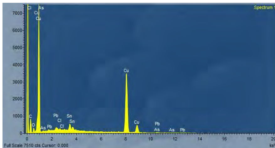
8a. kép – A „C” jelű félgomb tiszta fém részeire jellemző energiadiszperzív spektrum (Cu >> Sn, Pb >> As, Cl, S)
