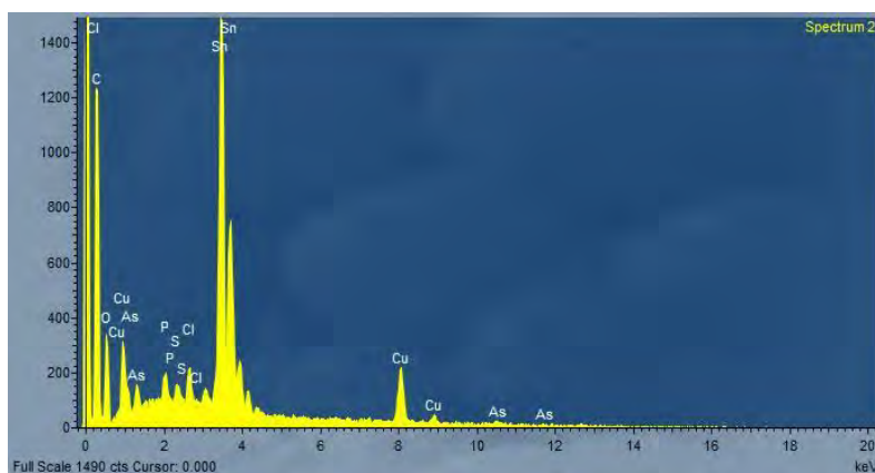
3. kép – Az összeillesztésben lévő anyag jellemző energiadisperzív spektruma (Sn >>> Cu, As, S, Cl, P)
