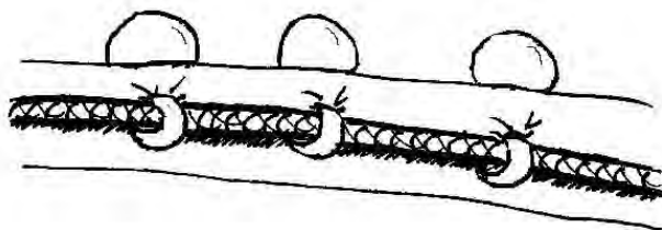
33b. kép – A fülesgombok felerősítési módja (rekonstrukciós rajz)
