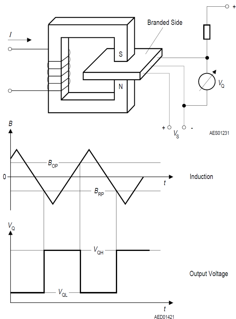
6.1. ábra. A felhasznált bipoláris Hall-szenzor működésének vázlata [13]
