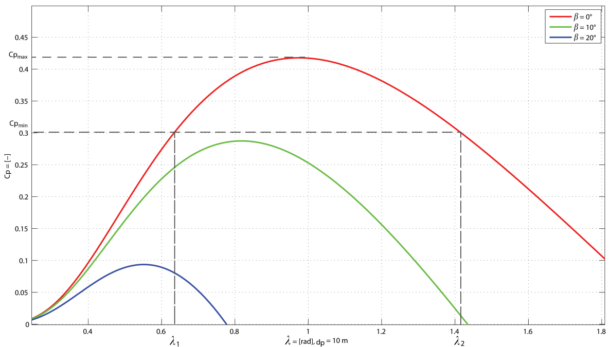
2.4. ábra. Formátényező a lapátvég-sebesség áttétel függvényében, d_p = 10 m
