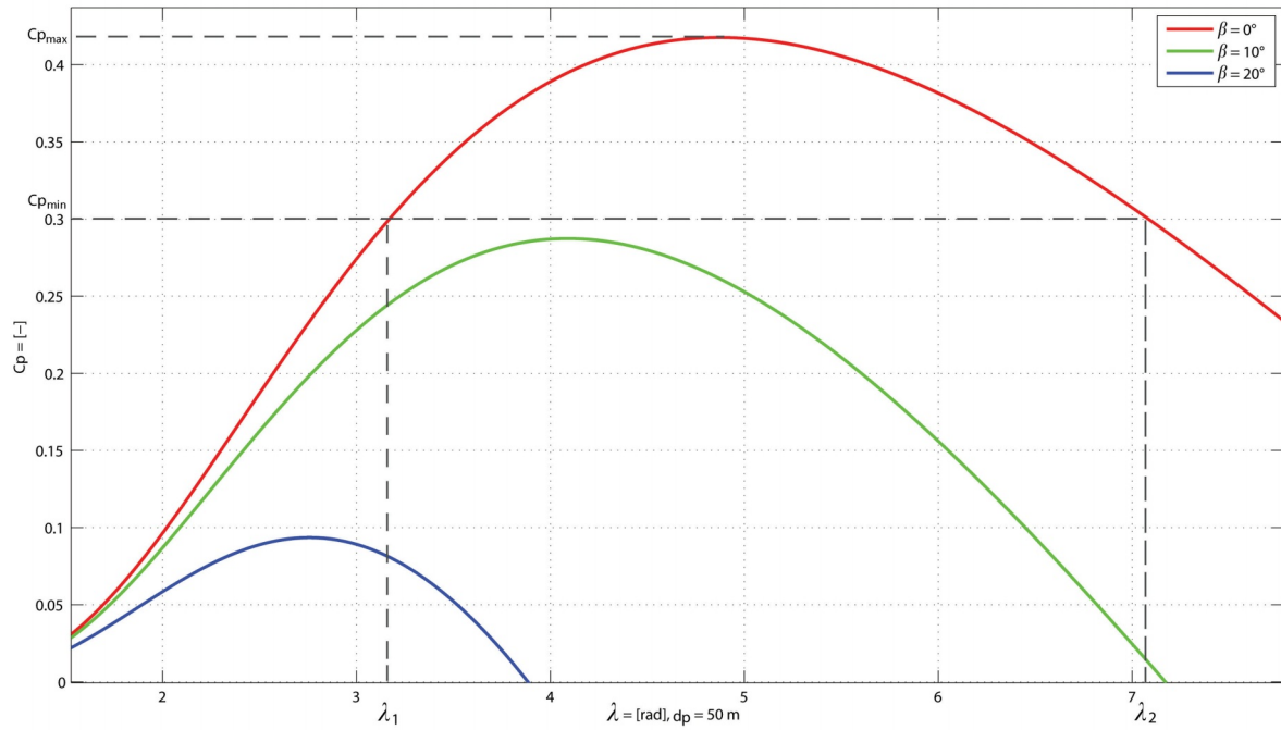
2.3. ábra. Formátényező a lapátvég-sebesség áttétel függvényében, d_p = 50 m
