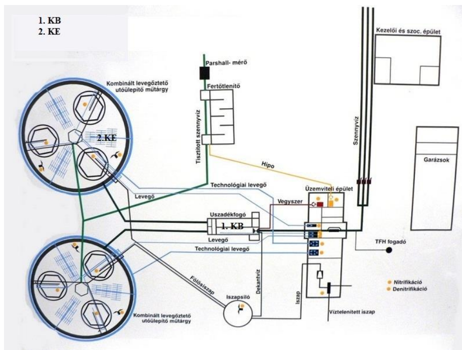
5. ábra Az Alsó-szigetközi Szennyvíztisztító telep OMS típusú szennyvízkezelő rendszer kapcsolási sémája [5]
