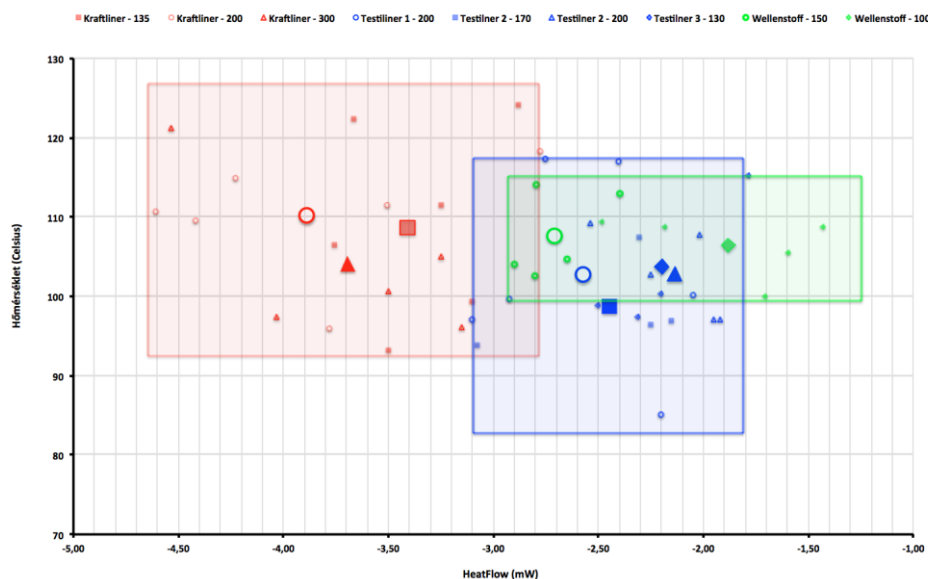
17. ábra: Az egyes alappapír típusok vizsgálati eredményeinek és szélsőértékük ábrázolása a csúcshőmérséklet és a hőáramlás függvényében
