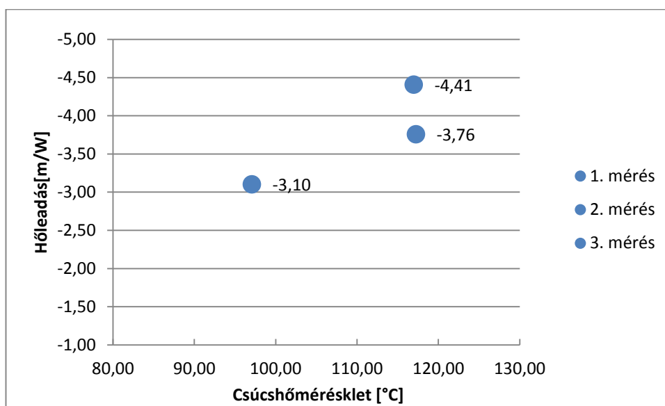
7. ábra: A Testliner I. típusú alappapír mérési eredményei
