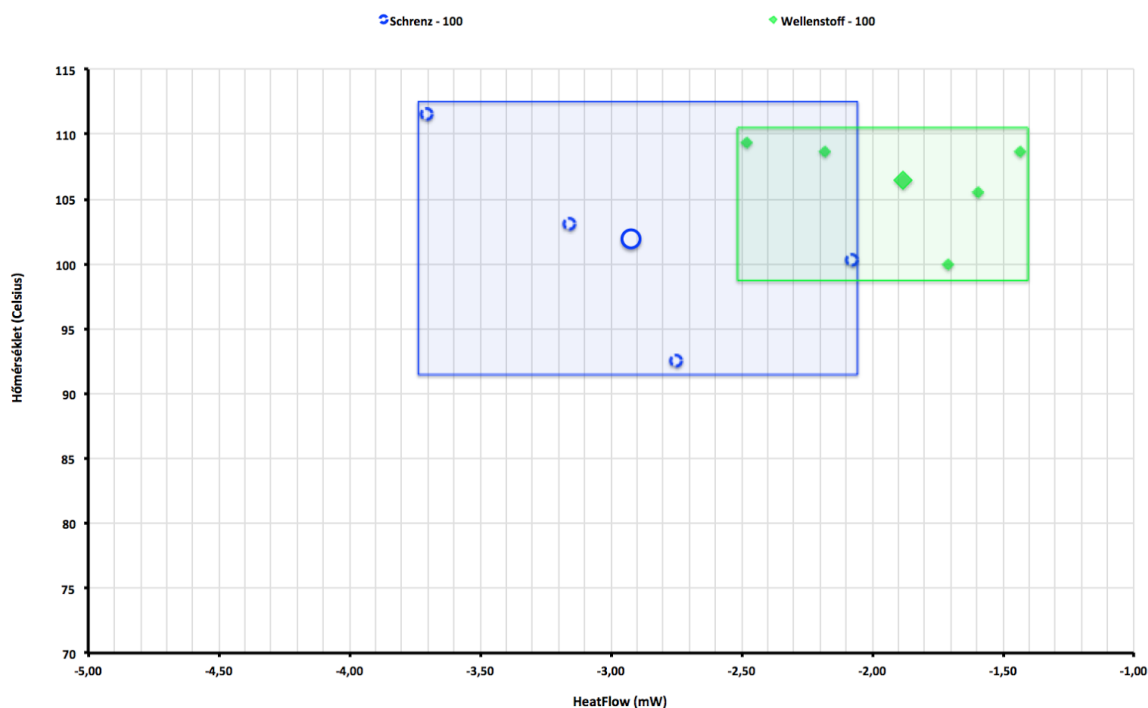
18. ábra: A Schrenz 100 és Wellenstoff 100 típusú alappapírok összehasonlító vizsgálati eredményeinek és szélsőértékük ábrázolása a csúcs hőmérséklet és a hőáramlás függvényében
