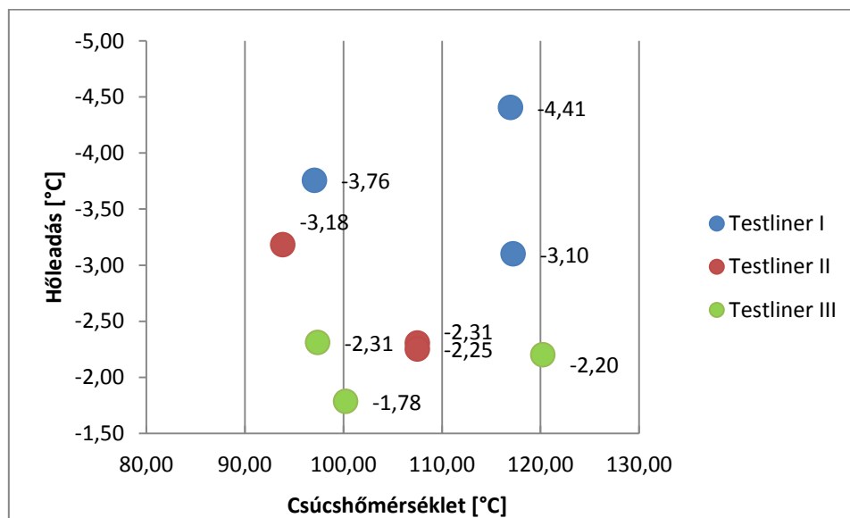
10. ábra: A Testliner típusú alappapírok összesített mérési eredményei
