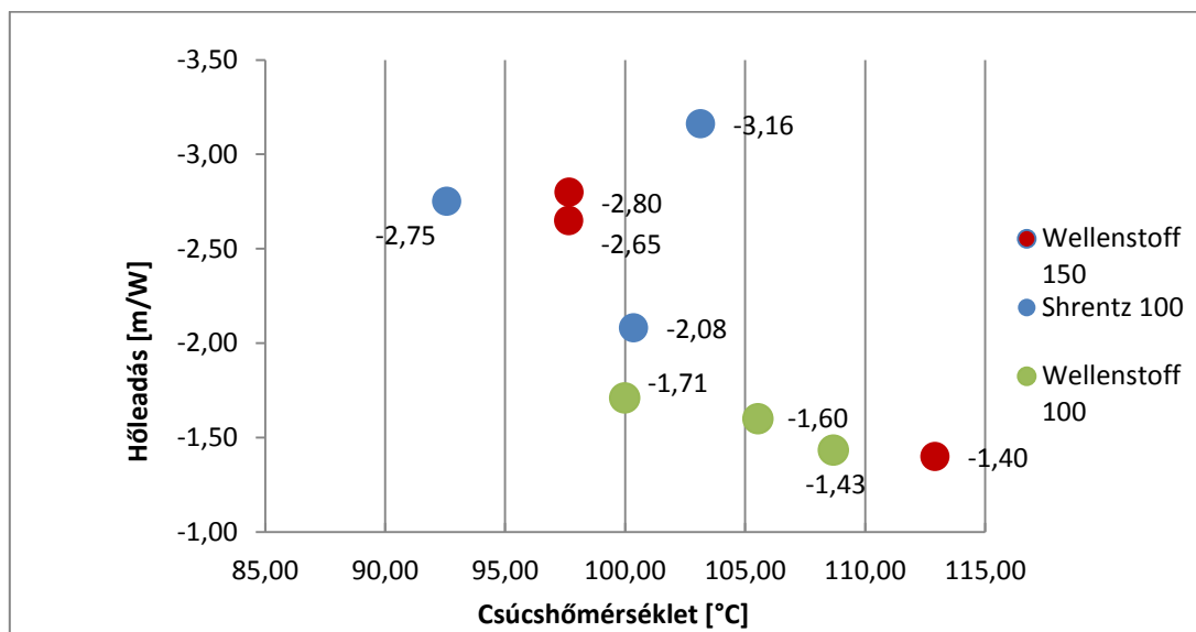
14. ábra: A Schrentz és Wellenstoff típusú alappapírok összesített mérési eredményei
