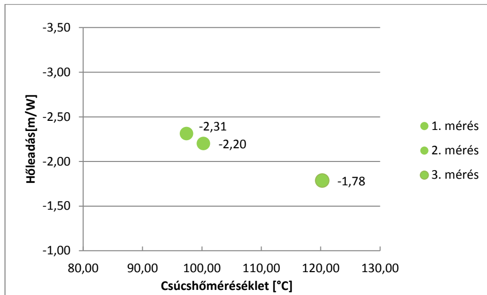
9.ábra: A Testliner III. típusú alappapír mérési eredményei
