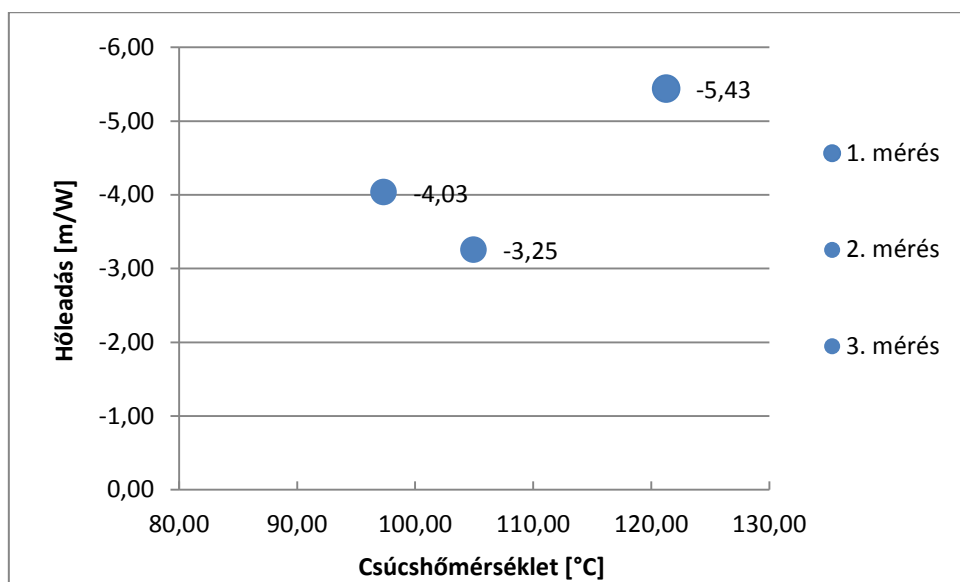
5. ábra: A Kraftliner 300 típusú alappapír mérési eredményei
