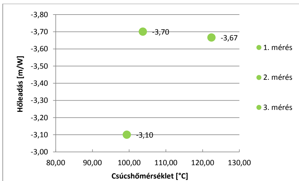
3. ábra: A Kraftliner 135 típusú alappapír mérési eredményei
