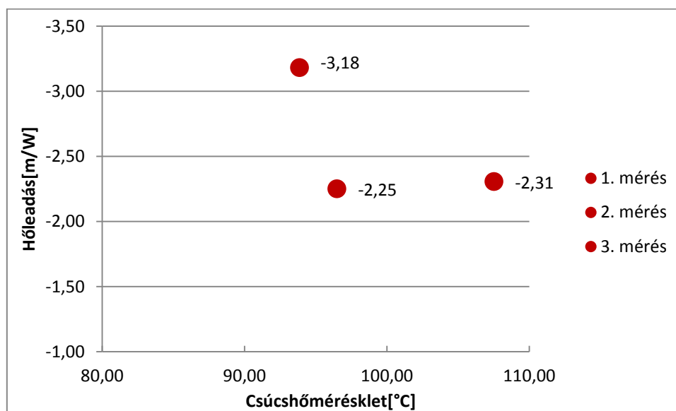
8. ábra: A Testliner II. típusú alappapír mérési eredményei
