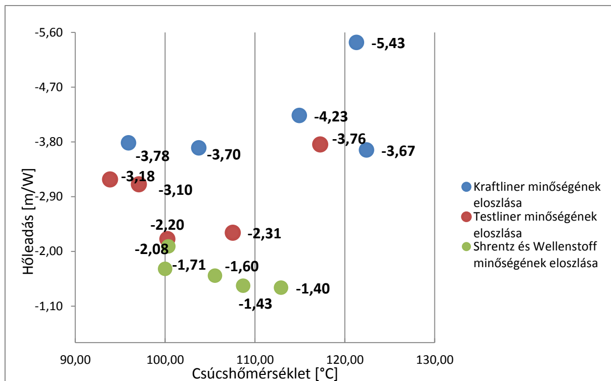
15. ábra: Az egyes alappapír típusok vizsgálati eredményei a csúcs hőmérséklet és a hőáramlás függvényében
