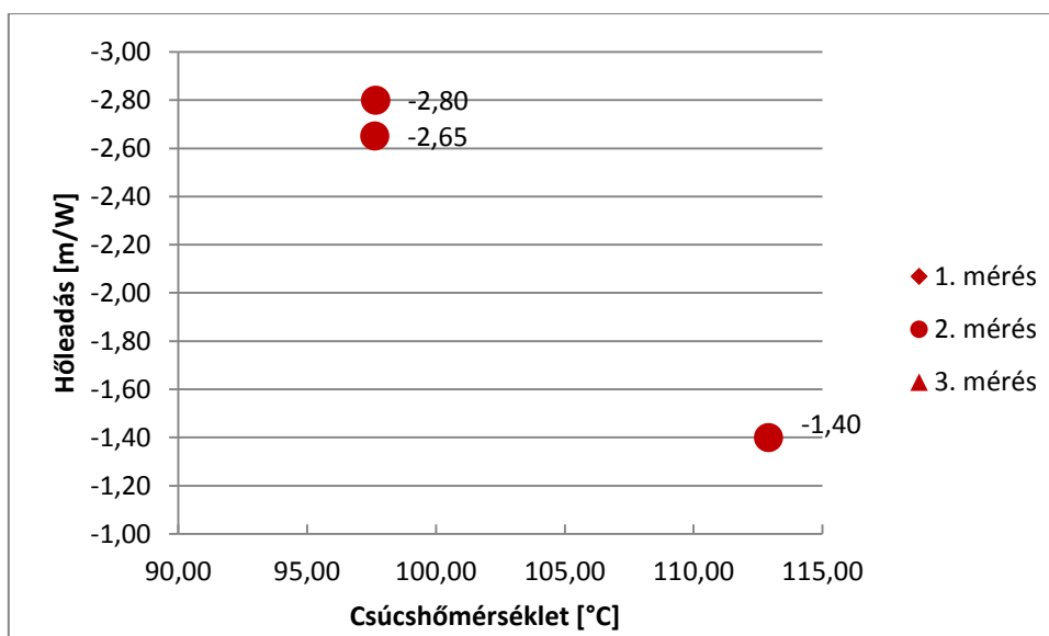
13. ábra: A Wellenstoff 150 típusú alappapír mérési eredményei
