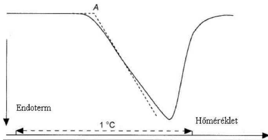
2. ábra: Jellegzetes differenciális termo analitikai görbe
