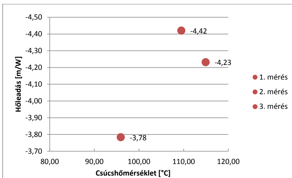
4. ábra: A Kraftliner 186 típusú alappapír mérési eredményei
