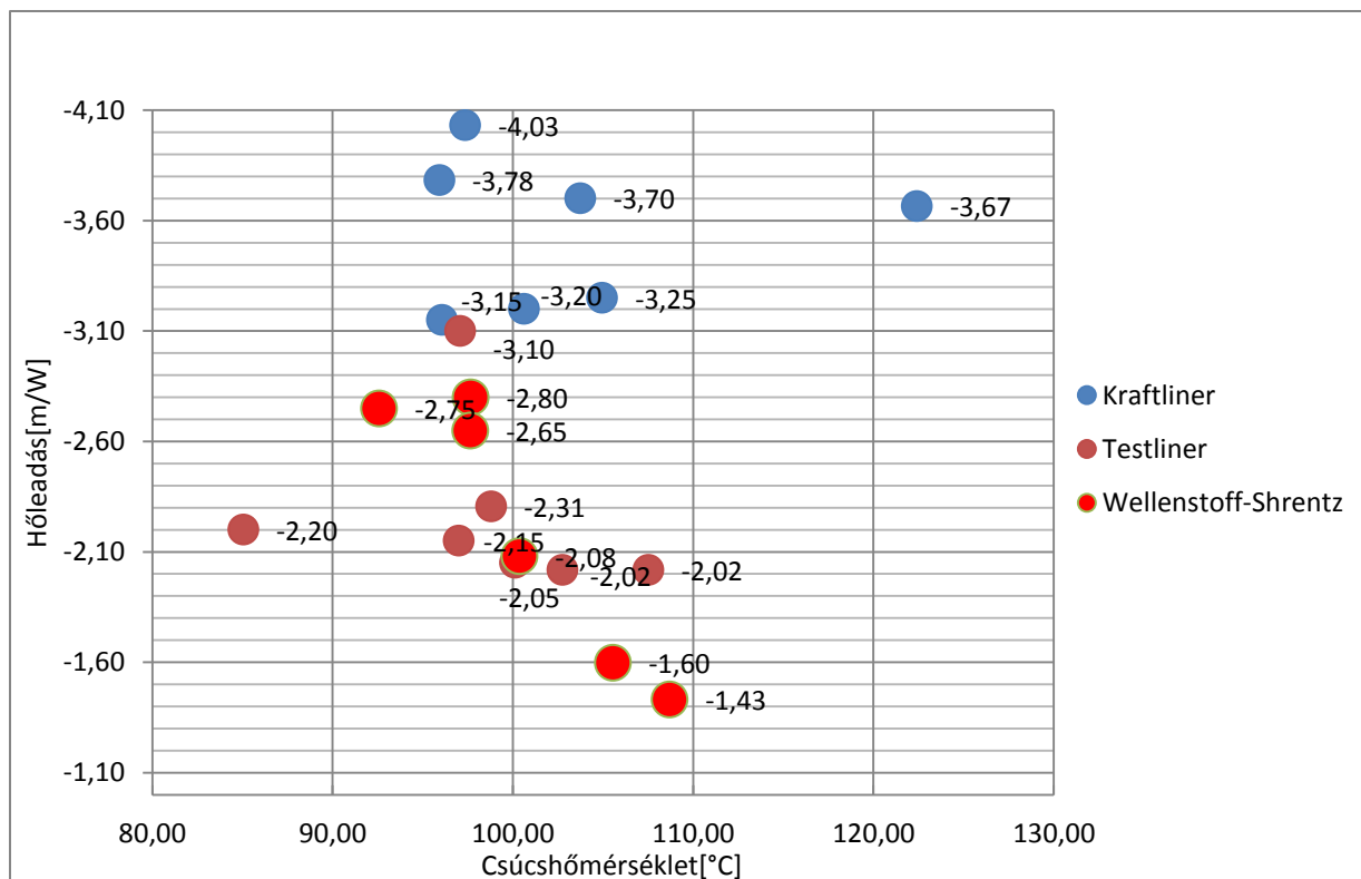
16. ábra: Az egyes alappapír típusok vizsgálati eredményei a csúcs hőmérséklet függvényében
