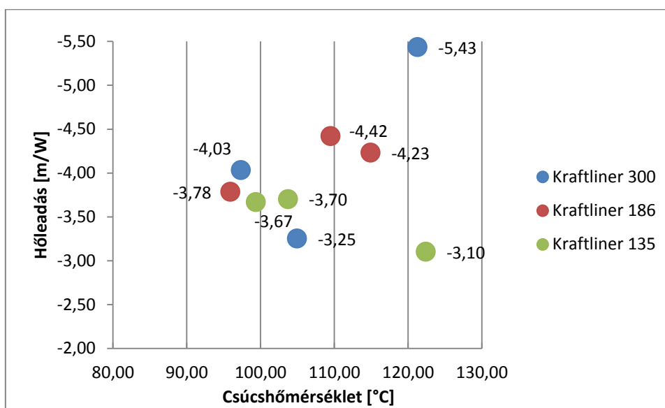
6. ábra: A Kraftliner típusú alappapírok összesített mérési eredményei
