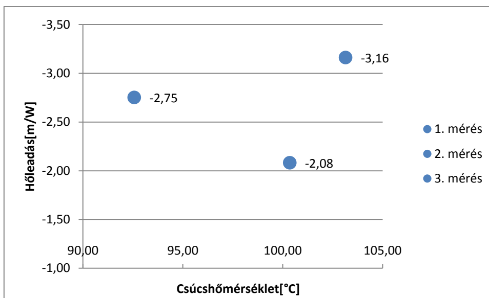
11. ábra: A Schrentz 100 típusú alappapír mérési eredményei
