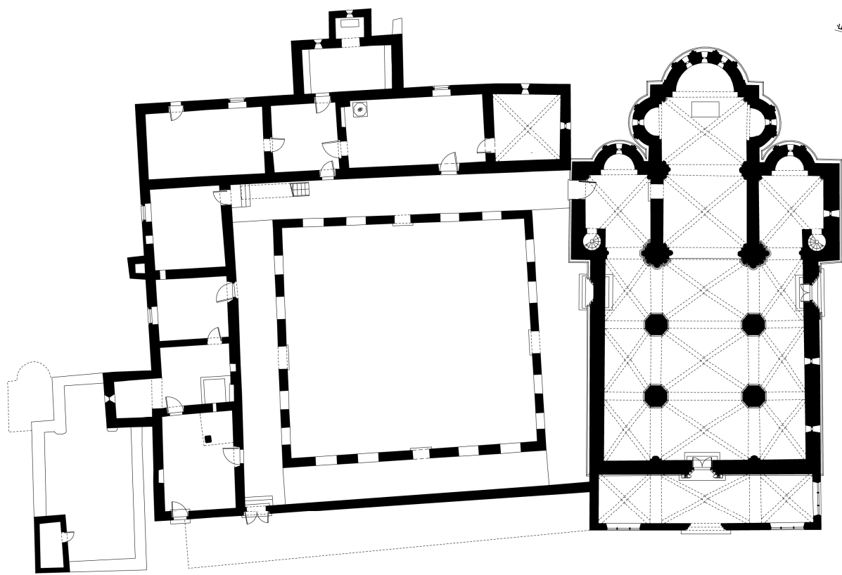
földszinti alaprajz
