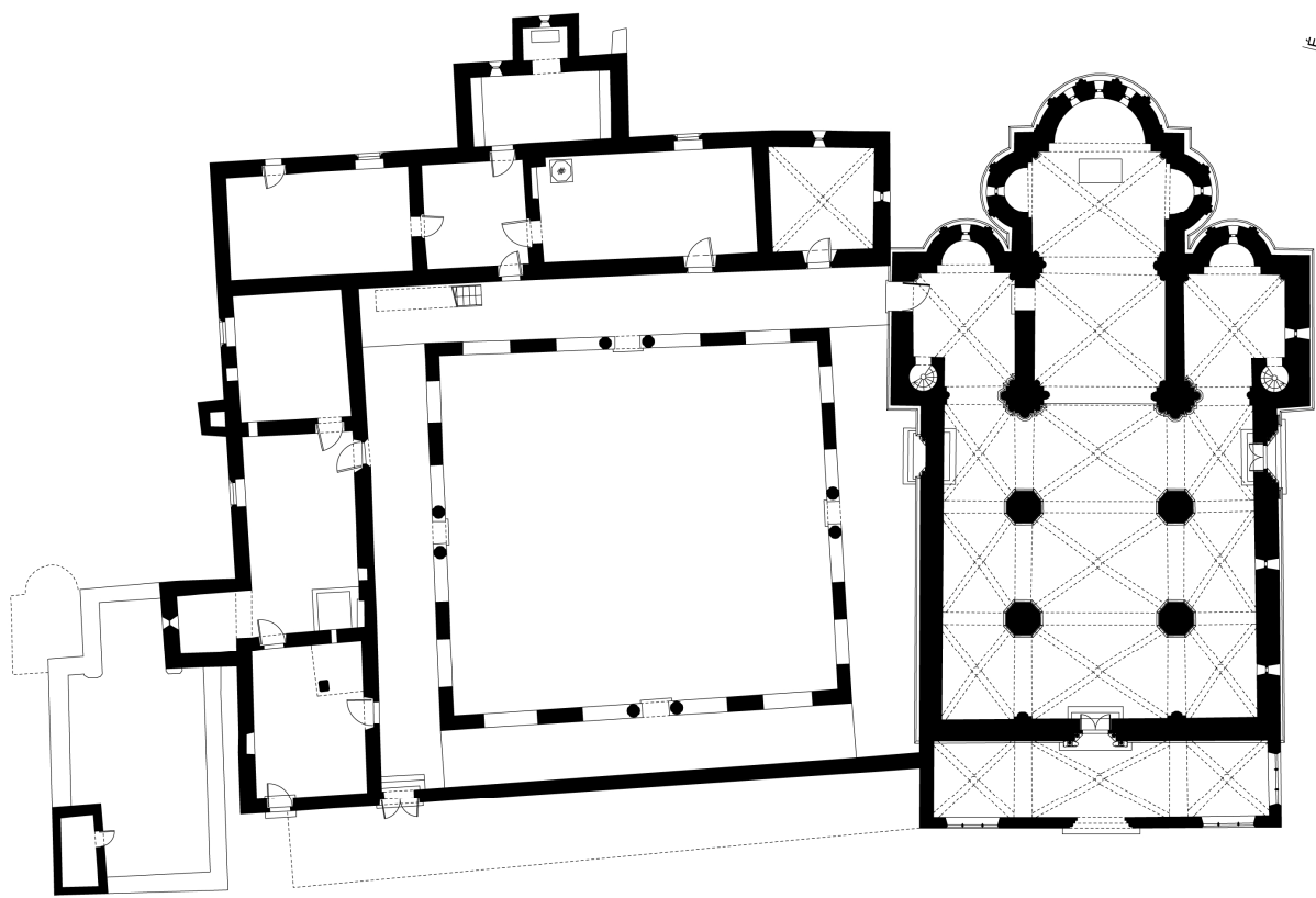
földszinti alaprajz
