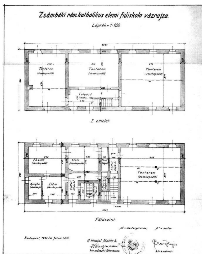
20. kép: A zsámbéki iskola bővítési terve
