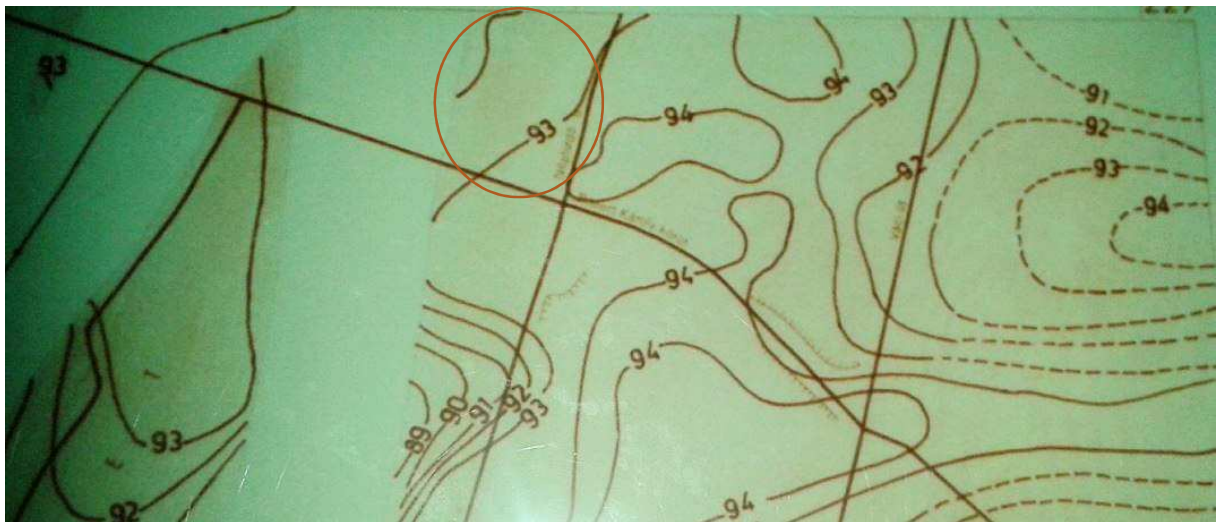
5. ábra: Agyagfekü izometrikus vonalai (mBf.) (BUDAPEST ÉPÍTÉSFÖLDTANI TÉRKÉPSOROZATA)
