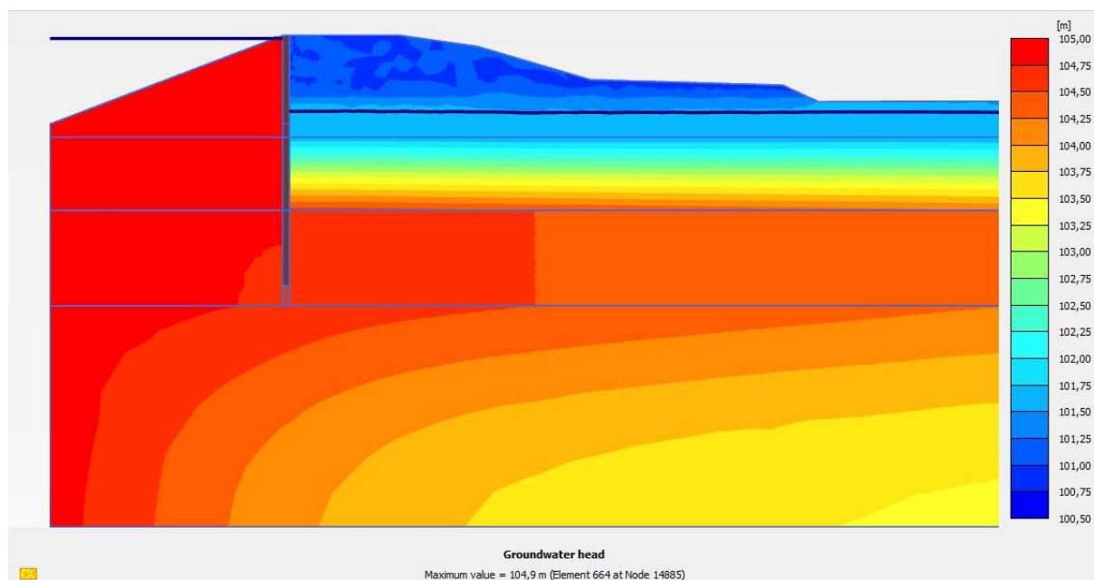
28. ábra: Kialakuló nyomásmagasságok – 3. eset (legsekélyebb résfal)
