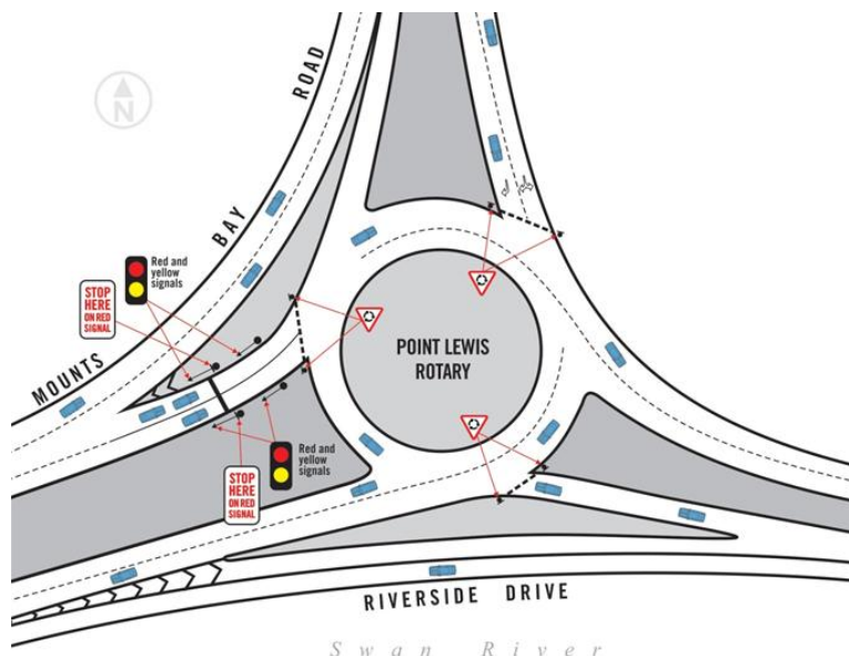
18. ábra Indirekt irányítású jelzőlámpával szabályozott körforgalom 1. 33
