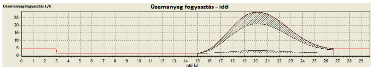
50. ábra Üzemanyag fogyasztás alakulása a sebességgel, gyorsulással összefüggésében 2. 92
