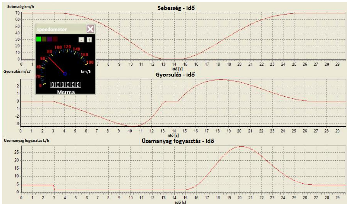
49. ábra Üzemanyag fogyasztás alakulása a sebességgel, gyorsulással összefüggésében 1. 91
