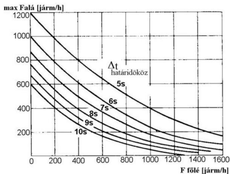
9. ábra Összefüggés az elsőbbséggel rendelkező úton haladó forgalom, a határidőköz és a mellékirányból átbocsátható max. forgalomnagyság között 19
