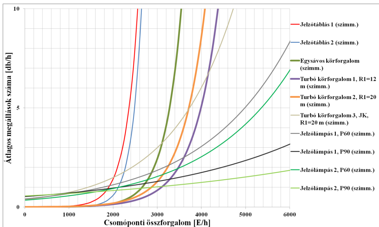
52. ábra A csomópont összforgalma és a járművenkénti átlagos megállások száma közötti összefüggés különböző csomópont típusoknál, szimmetrikus forgalomterhelés mellett
