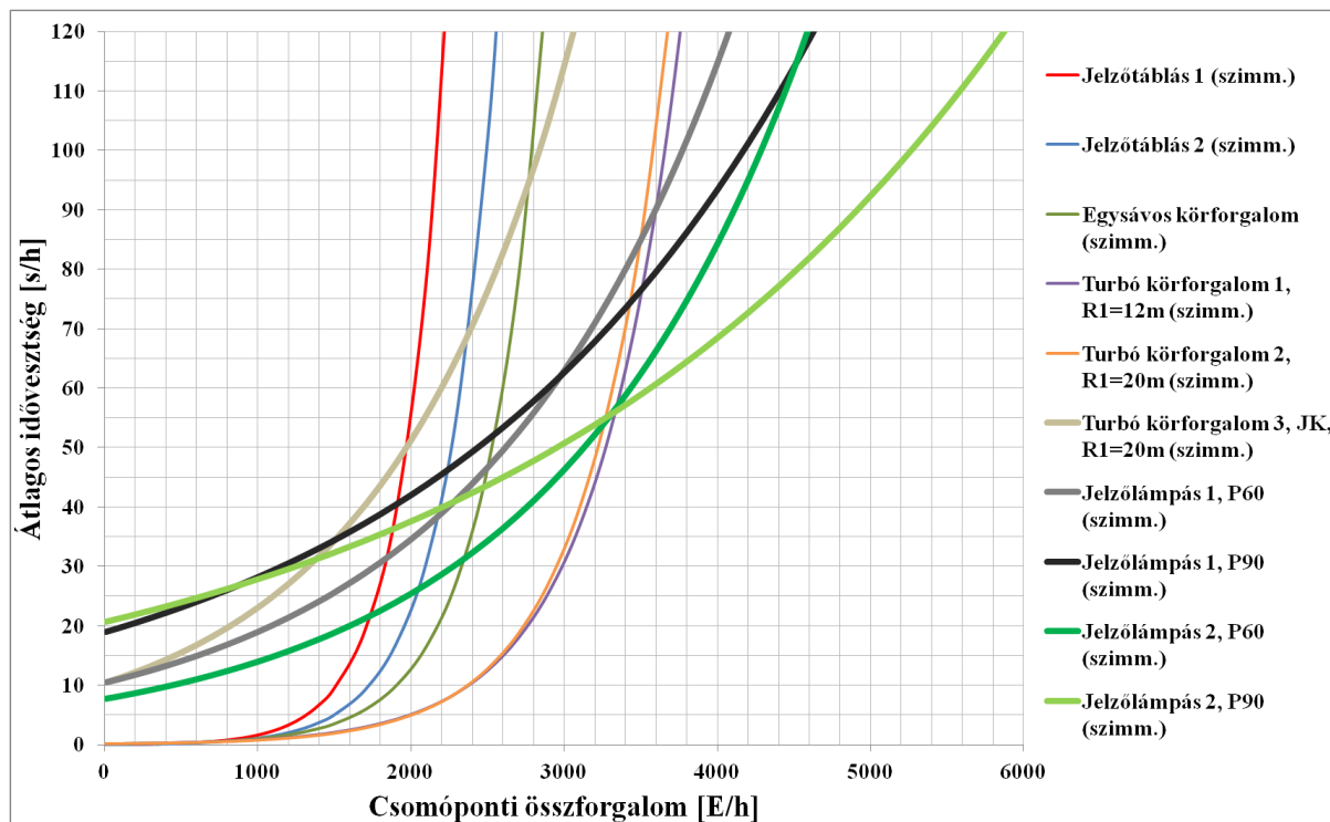
47. ábra A csomópont összforgalma és járművenkénti átlagos idővesztés összefüggése különböző csomópont típusoknál, szimmetrikus forgalomterhelés mellett
