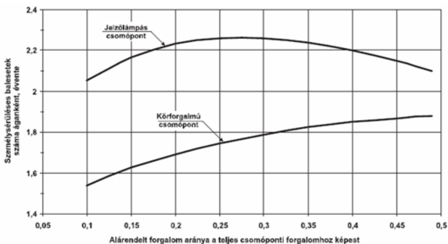
F.4. ábra – Balesetek a jelzőlámpás és körforgalmú csomópontok esetében, teljes csomóponti forgalom: 30 000 jármű/nap
