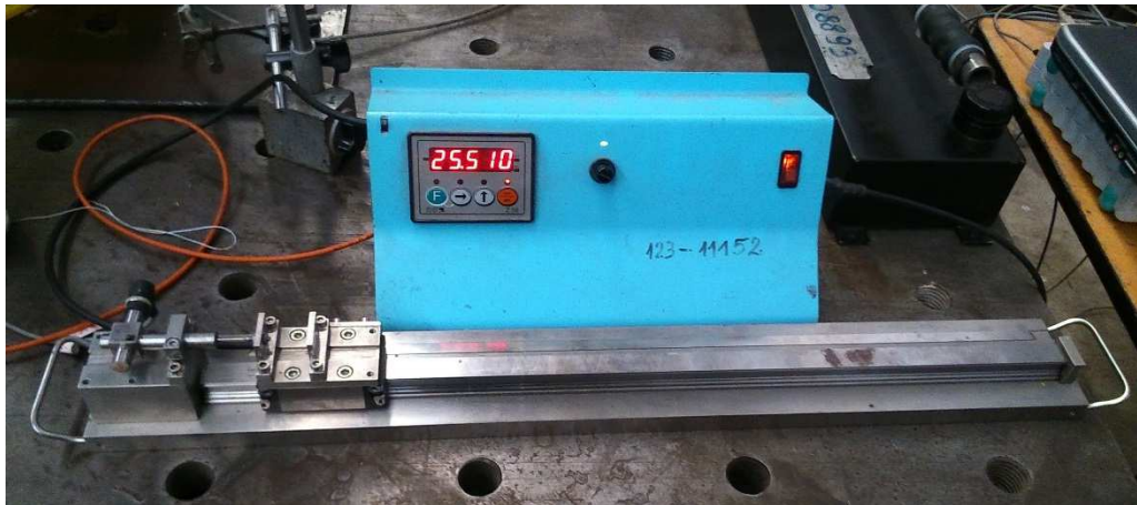
M5-1. kép Az induktív úradók kalibrálásához használt mérőasztal
