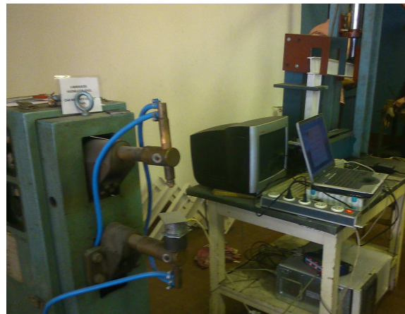
5.3 kép Elektroda összeszorító erő mérése - mérési összeállítás
