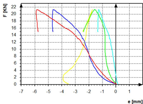
4.6 ábra B200-...-01 tesztelem F-e grafikonja (kN-mm)
