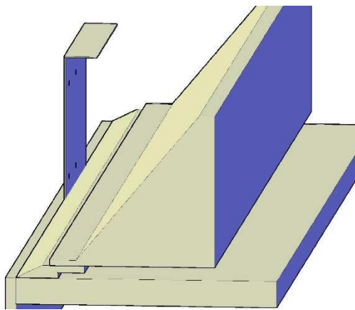
3.5 ábra Élhajlítás ellenőrzése: gerinc alkotóelem kialakításánál
