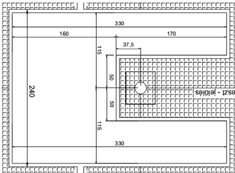
6.1 ábra A gépasztal munkalapjának fontosabb méretei
