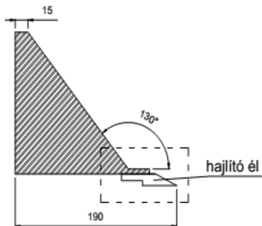
3.1 ábra Lemzhajlító gép sematikus ábrája
