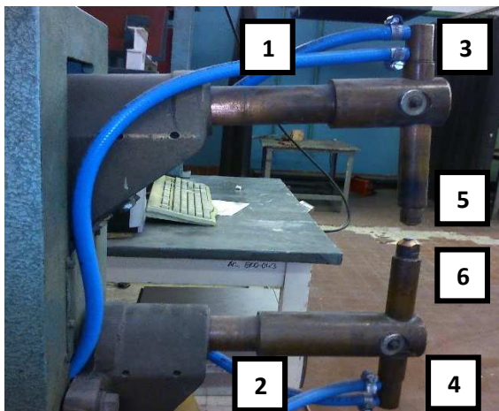
2.2 kép A hegesztő ablak részei – a gépasztal szempontjából lényegesebb gépalkatrészek elnevezése
