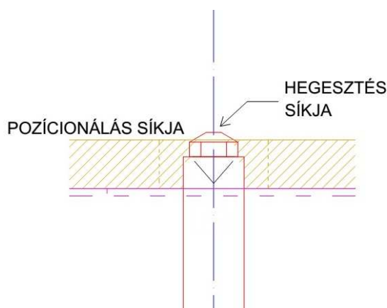
2.4 ábra Munkalap megfelelő állása síklemezek hegesztése esetén
