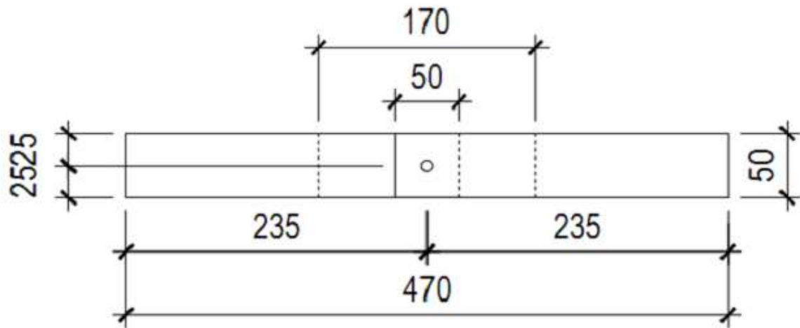
5.3 ábra Szabványos egy pontvarratos próbatest (MSZ EN ISO 14270:2002)
