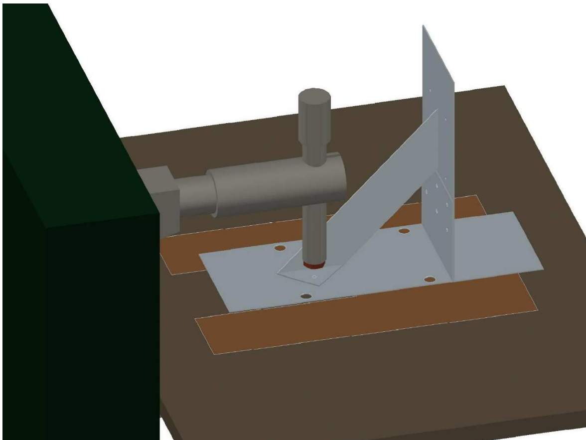
3.3 ábra Hegesztett kapcsolat ellenőrzése: Borda alsó fül + alaplemez
