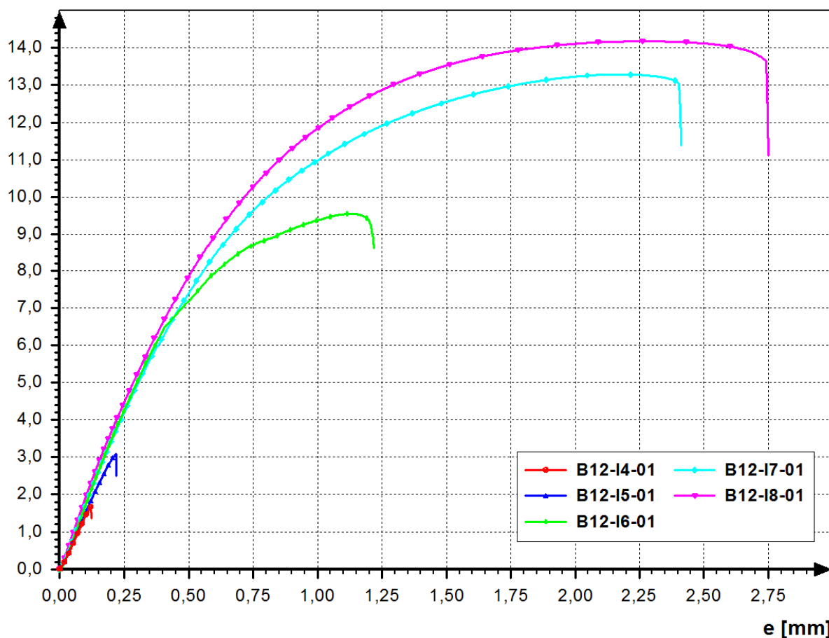
5.5 ábra Egy pontvarratos kapcsolatok nyíró-szakító jelleggörbéi
