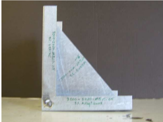
3.3 kép B200-2U10-1AB10 baktípus egyik gyártmánya
