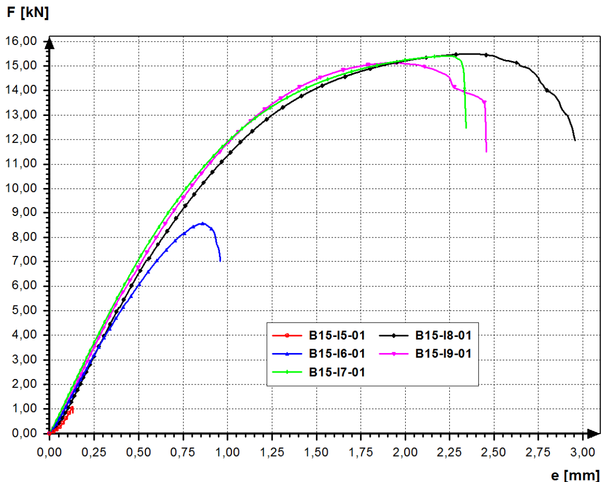
5.6 ábra Egy pontvarratos kapcsolatok nyíró-szakító jelleggörbéi (1,5 mm x 1,5 mm)
