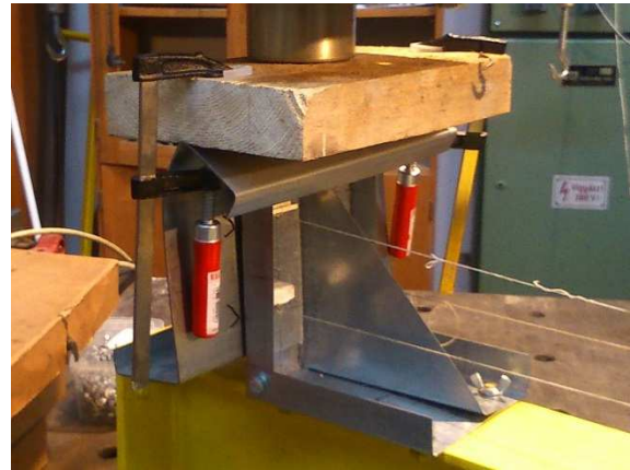
2.6 kép Z-szelemen alakváltozása terhelés után
