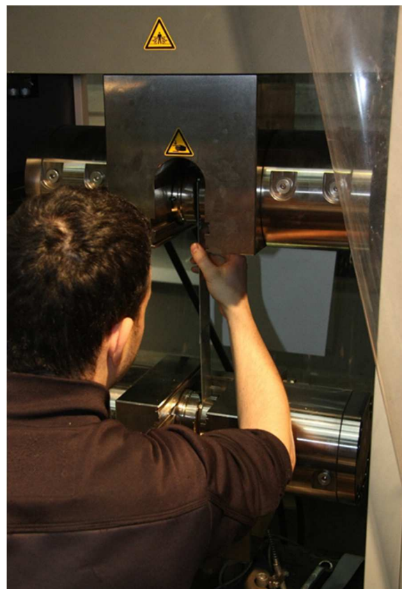
5.17 kép Próbatest befogása egy ZWICK ROLL Z400 szakítógépbe
