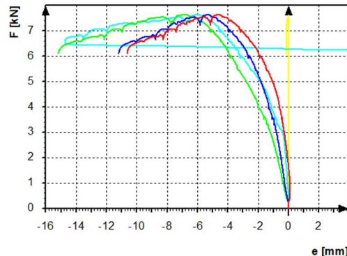
4.7 ábra B200-...-02 tesztelem F-e grafikonja (kN-mm)
