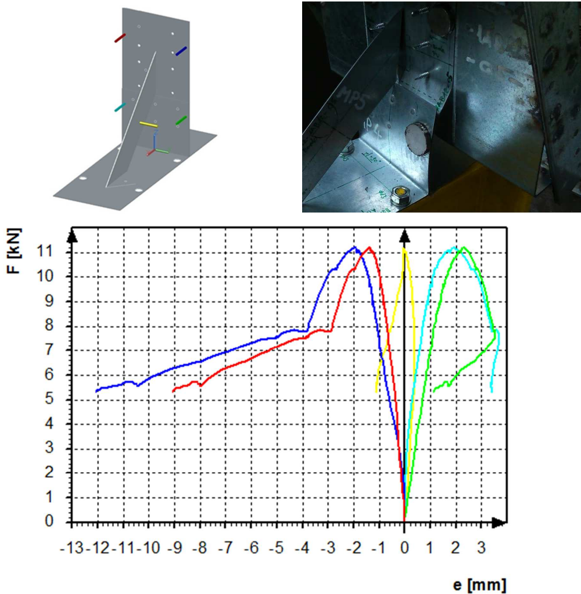
4.3 ábra B200-2L12-1AB12-05 tesztelem sematikus ábrája a tönkremenetel pillanatát és F-e grafikonja (kN-mm)
