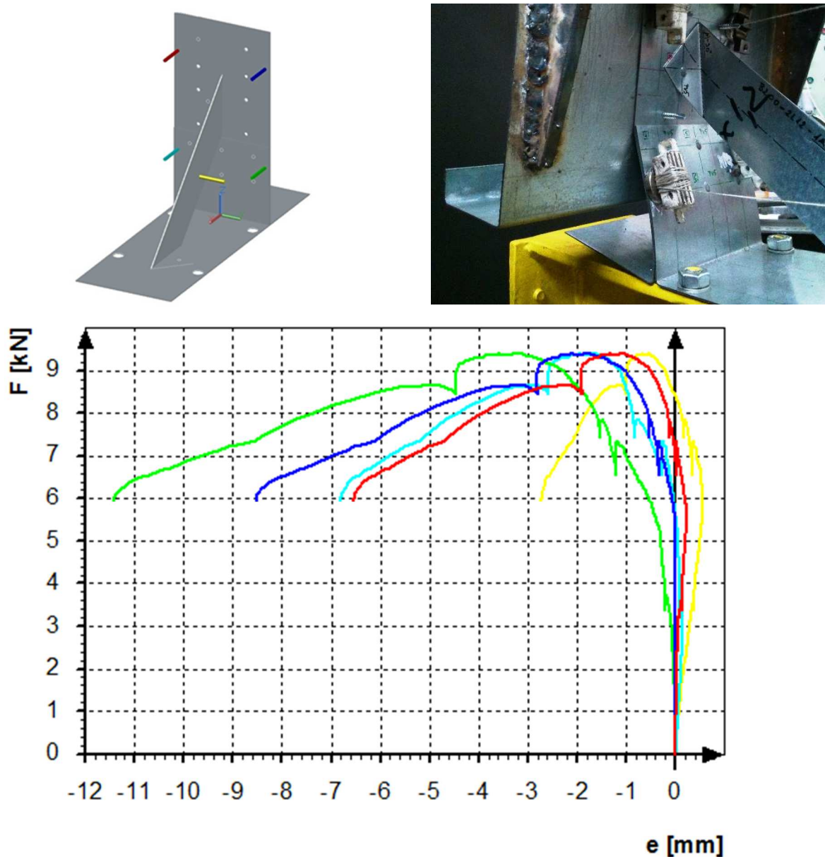
3.1 ábra B200-2L12-1AB12-02 tesztelem sematikus ábrája a tönkremenetel pillanatát és F-e grafikonja (kN-mm)
