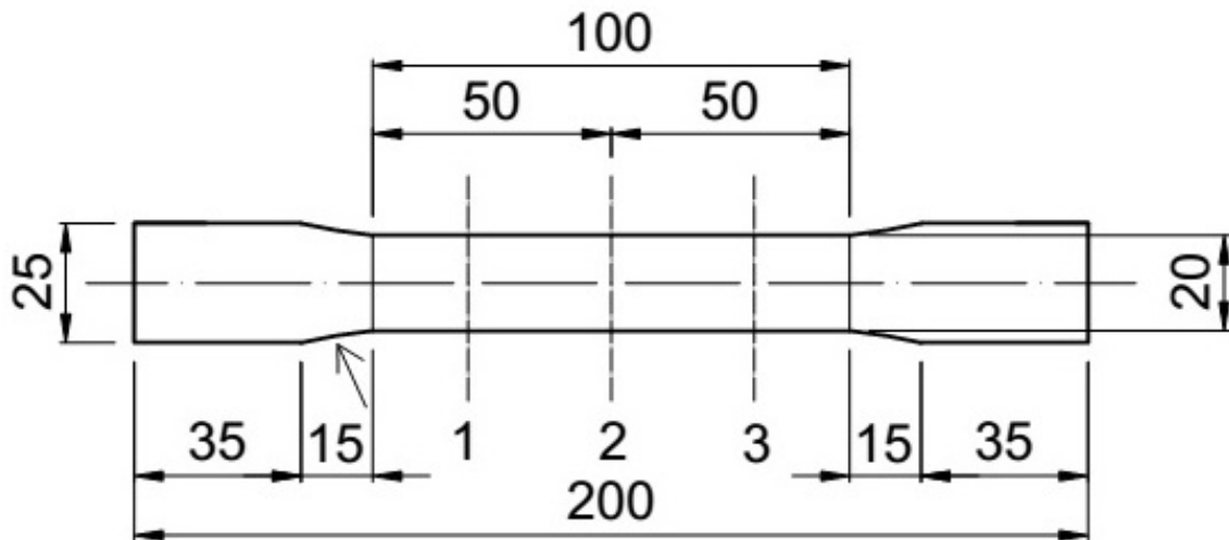
3.1 ábra A szakítóvizsgálathoz alkalmazott próbatest kialakítása
