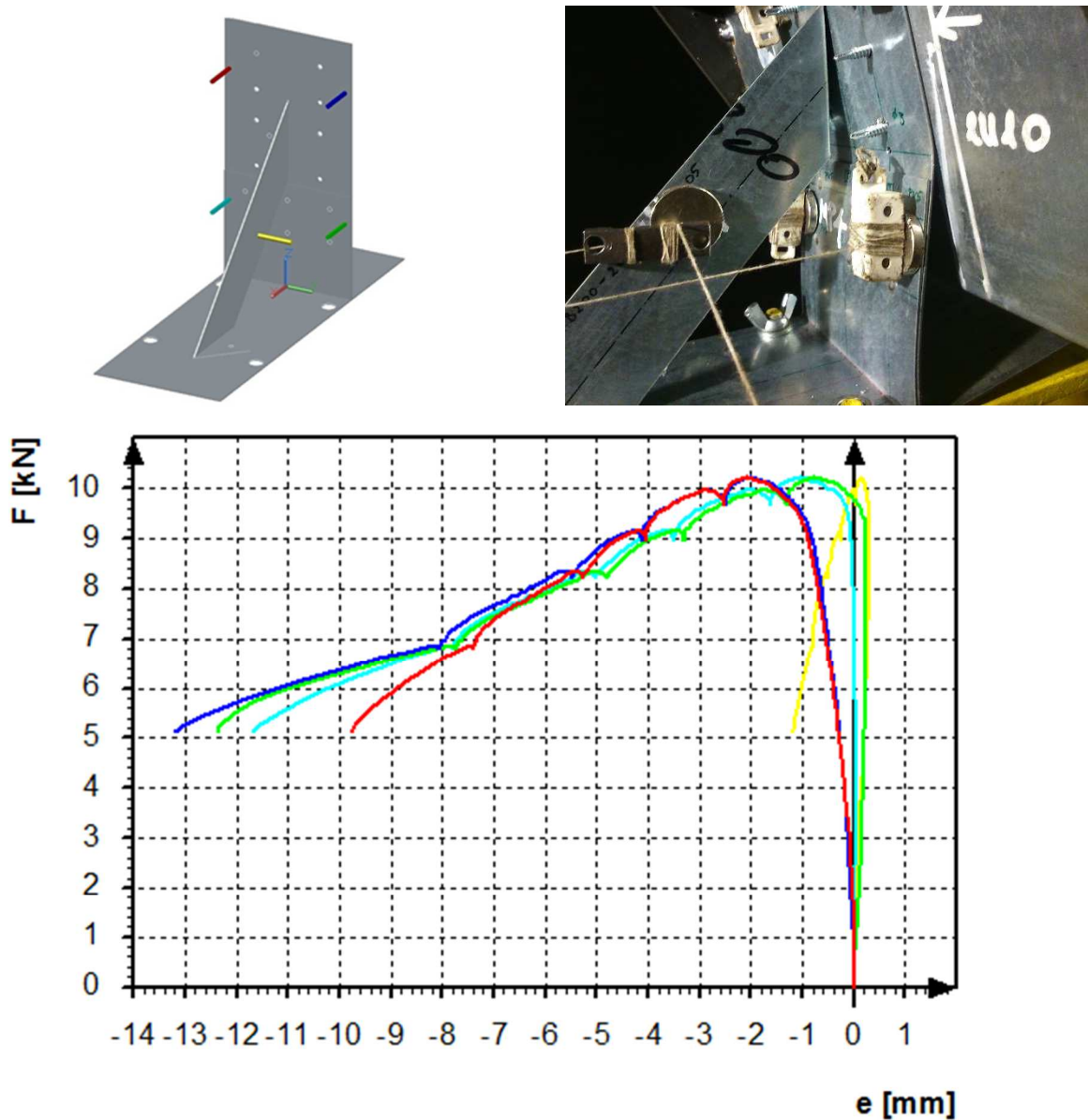
4.1 ábra B200-2L12-1AB12-03 tesztelem sematikus ábrája a tönkremenetel pillanatát és F-e grafikonja (kN-mm)
