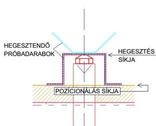
2.5 ábra Munkalap pozíciója a hegesztési síkhoz képest bonyolultabb elemek esetén
