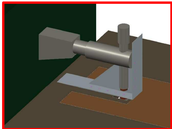
3.11 ábra I. SZE hegesztése: Belső pontvarrat elkészíthetőségének vizsgálata
