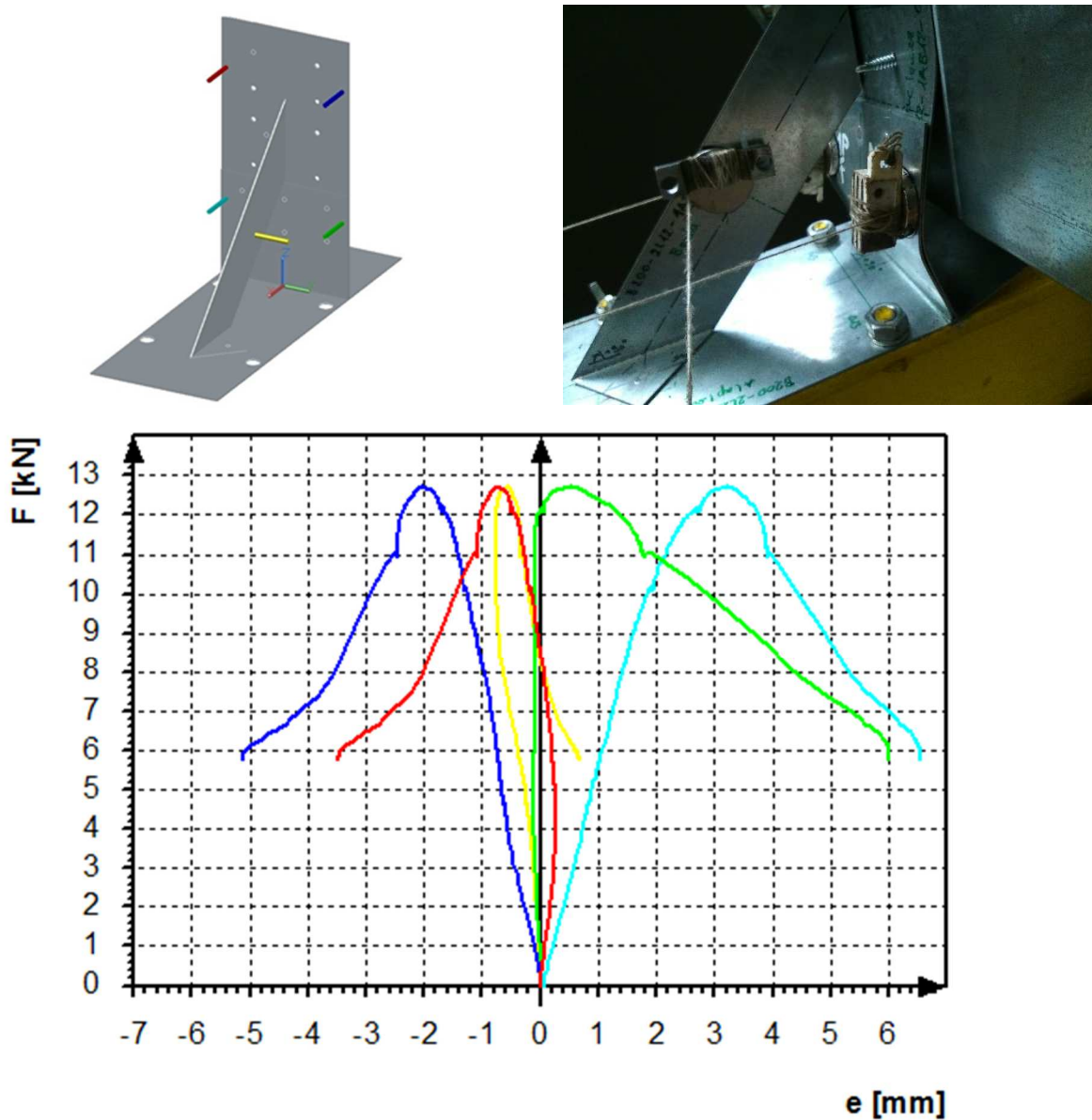
4.2 ábra B200-2L12-1AB12-04 tesztelem sematikus ábrája a tönkremenetel pillanatát és F-e grafikonja (kN-mm)
