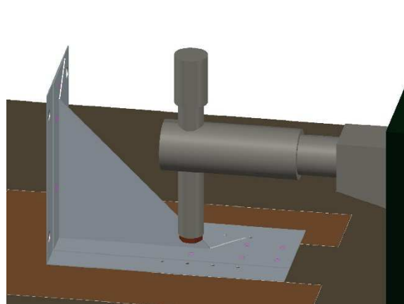
3.13 ábra A felső elektródatartó elfér a gerincborda mellett
