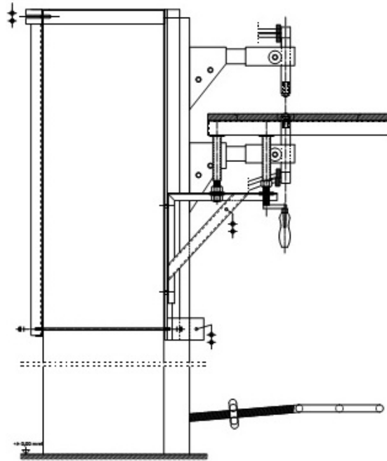
2.1 ábra A gépasztal sematikus ábrája
