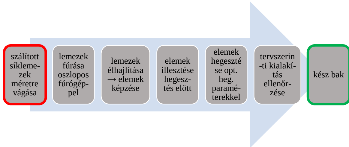
2.1 ábra A bak gyártásának folyamatábrája
