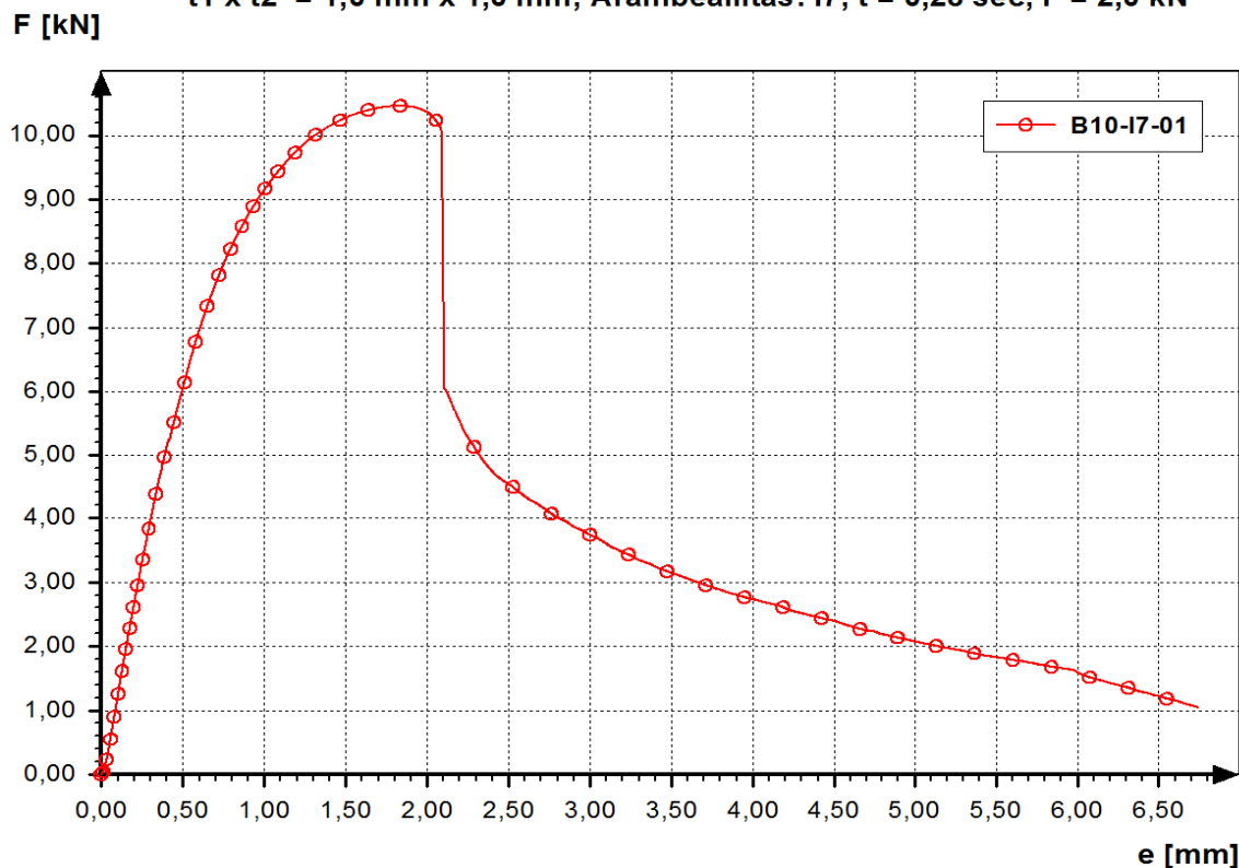
Egy pontvarratos kapcsolat nyíró-szakító vizsgálata t_1 \times t_2 = 1,0 \text{ mm} \times 1,0 \text{ mm} ; Árambeállítás: I7, t = 0,28 \text{ sec} , F = 2,0 \text{ kN}
