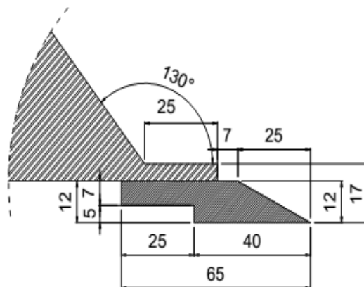
3.2 ábra Hajlítóél méretei
