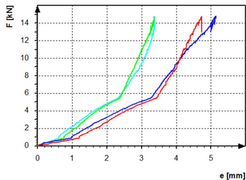
1.3 ábra B200-2U10-1AB10-02 tesztelem F-e grafikonja (kN-mm)
