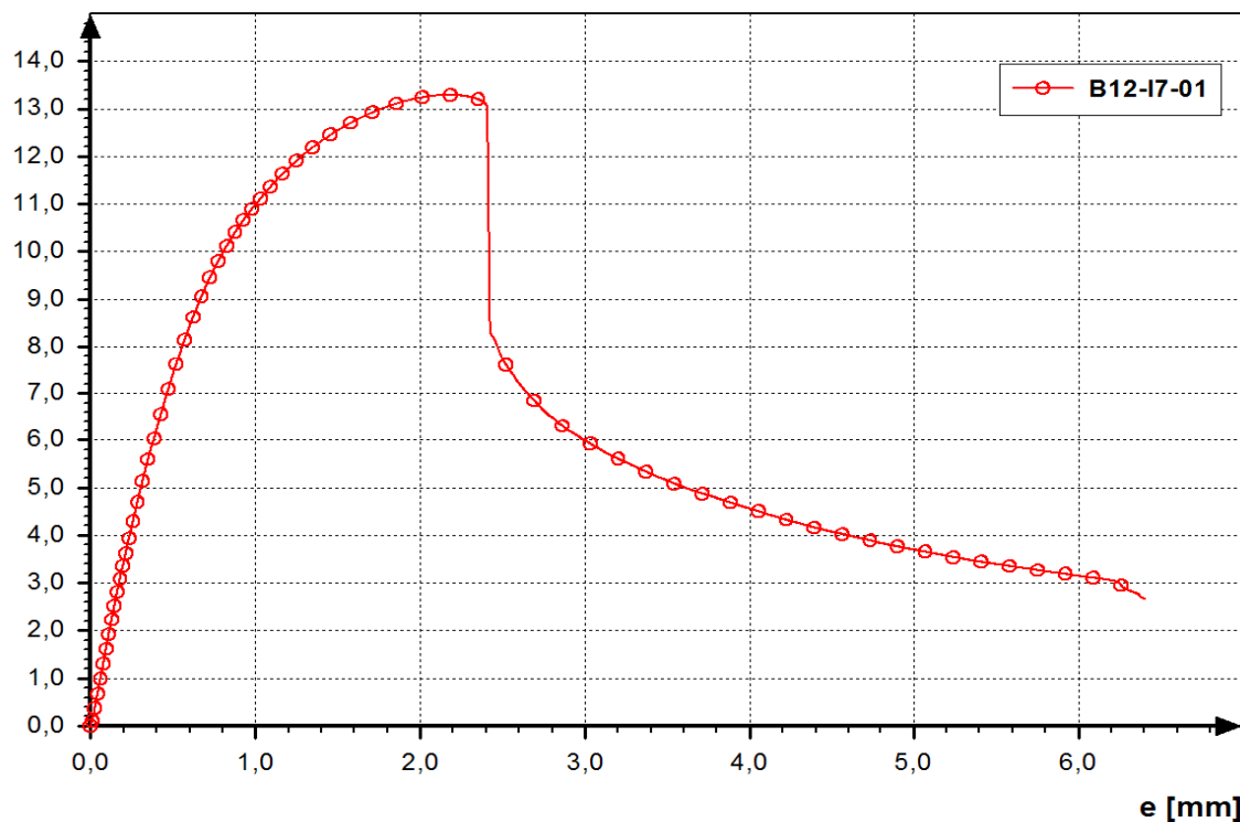
Egy pontvarratos kapcsolat nyíró-szakító vizsgálata t_1 \times t_2 = 1,2 \text{ mm} \times 1,2 \text{ mm} ; Árambeállítás: I7, t = 0,28 \text{ sec} , F = 2,0 \text{ kN}
