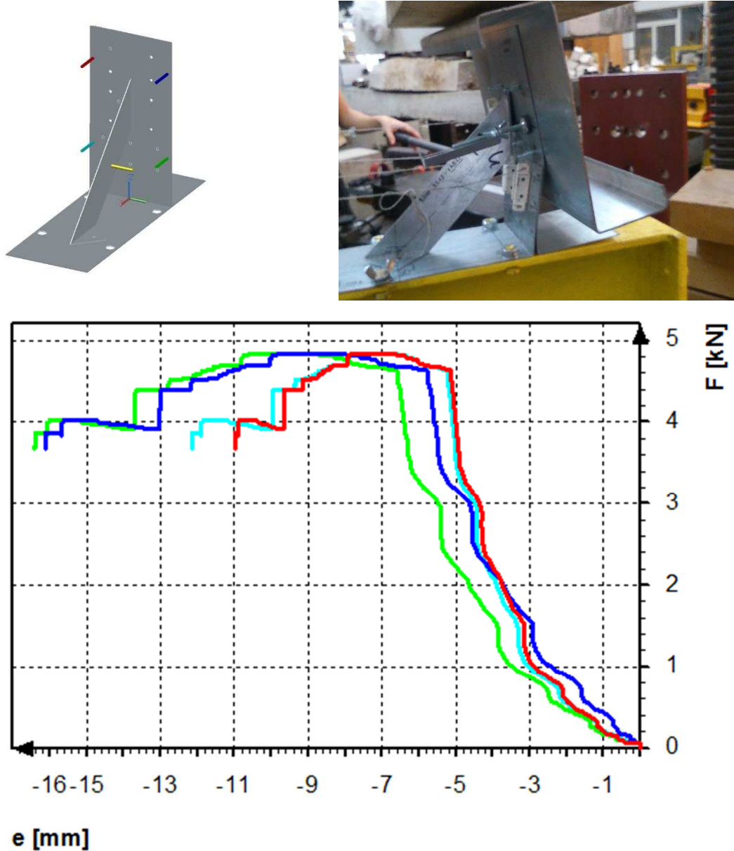
1.1 ábra B200-2L12-1AB12-01 tesztelem sematikus ábrája és F-e grafikonja (kN-mm)
