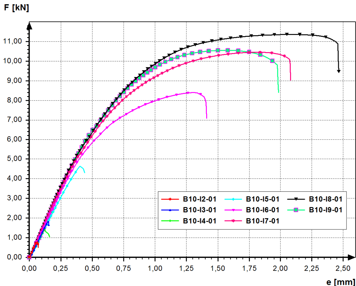
5.4 ábra Különböző áramerősségek mellett, 1,0 mm vastag lemezekből ellenállás-ponthegesztés technológiával kialakított egy pontvarratos kapcsolatok nyíró-szakító jelleggörbéi
