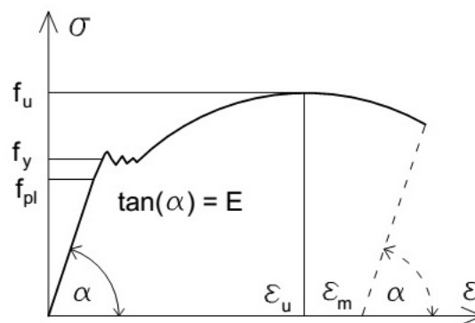
2.2 ábra Természetes folyáshatárral rendelkező anyag húzódiagramja
