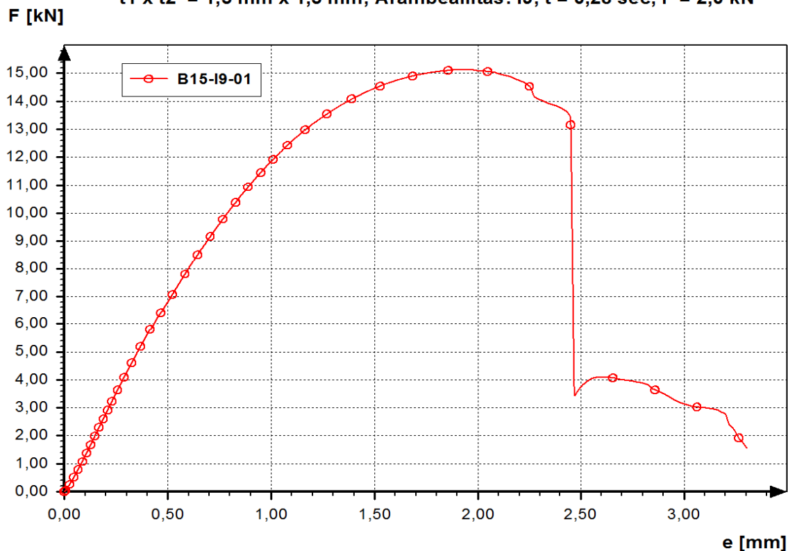
Egy pontvarratos kapcsolat nyíró-szakító vizsgálata t_1 \times t_2 = 1,5 \text{ mm} \times 1,5 \text{ mm} ; Árambeállítás: I9, t = 0,28 \text{ sec} , F = 2,0 \text{ kN}
