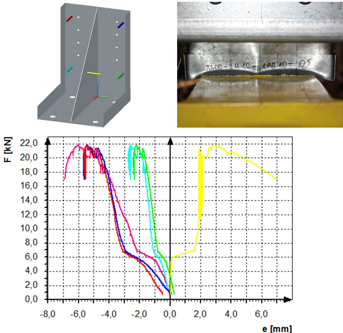
5.1 ábra B200-2U10-1AB10-05 tesztelem sematikus ábrája a tönkremenetel pillanatát és F-e grafikonja (kN-mm)
