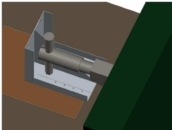
3.7 ábra Hegesztett kapcsolat ellenőrzése: Borda felső fül + gerinc
