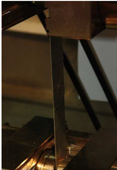
5.08 kép Próbatest a terhelés elején
