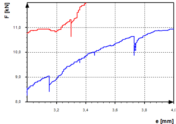
1.4 ábra Csavarkihúzódnás jelensége az F-e grafikonon (B200-2U10-...-01)
