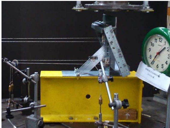
4.1 kép Negyedik tesztsorozat kísérleti összeállítása
