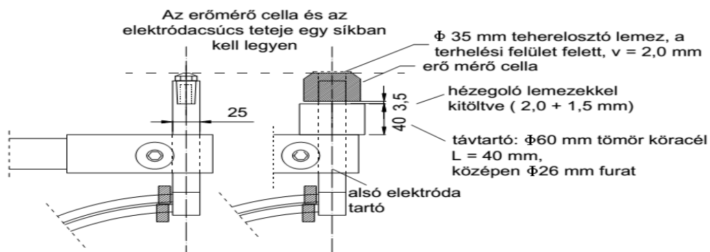
5.2 ábra A mérési összeállítás vázlatrajza
