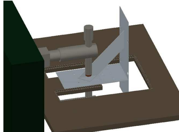
3.2 ábra Hegesztett kapcsolat ellenőrzése: Borda felső fül + gerinc
