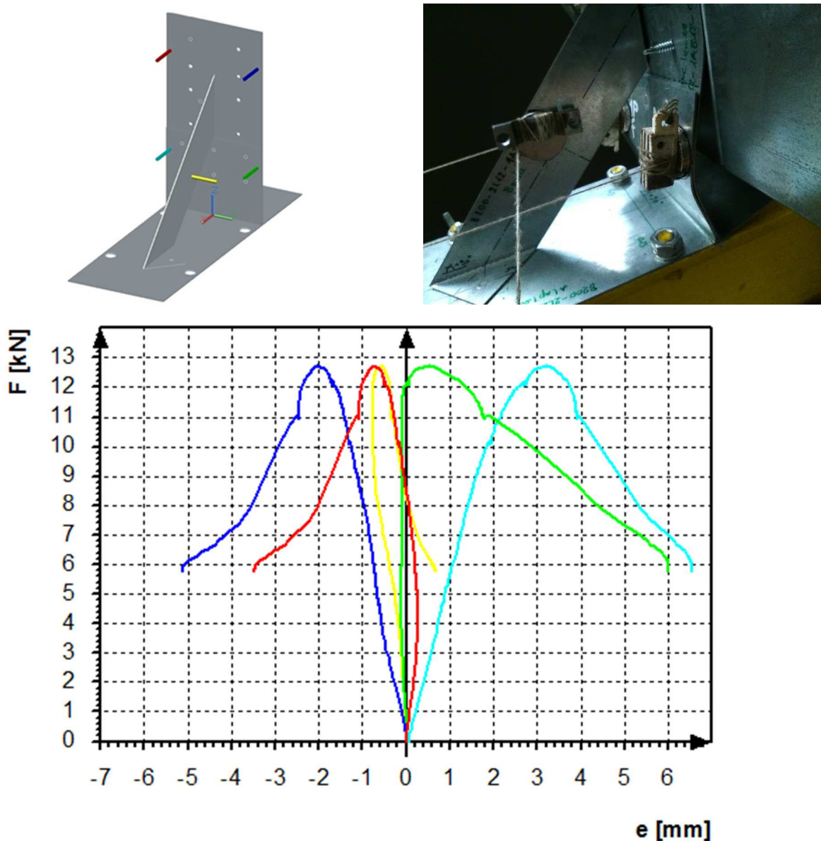
4.2 ábra B200-2L12-1AB12-04 tesztelem sematikus ábrája a tönkremenetel pillanatát és F-e grafikonja (kN-mm)
