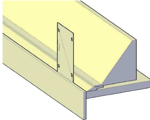
3.10 ábra élhajlítás ellenőrzése a gerinc alkotóelem kialakításánál
