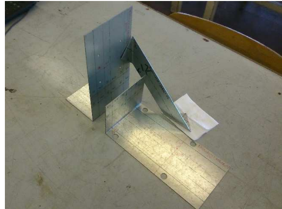
3.2 kép Egymásnak támasztott alkotóelemek
