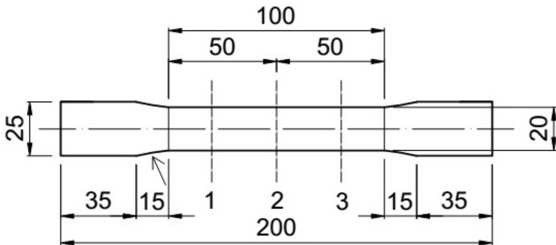
3.1 ábra A szakítóvizsgálathoz alkalmazott próbatest kialakítása
