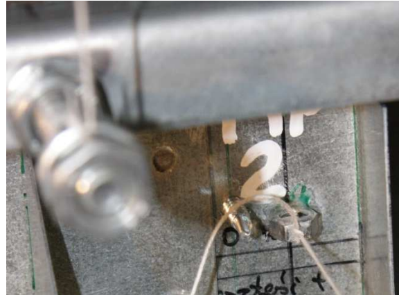
5.2 kép Mérőműszerek kialakítása: induktív adók + anyacsavarok
