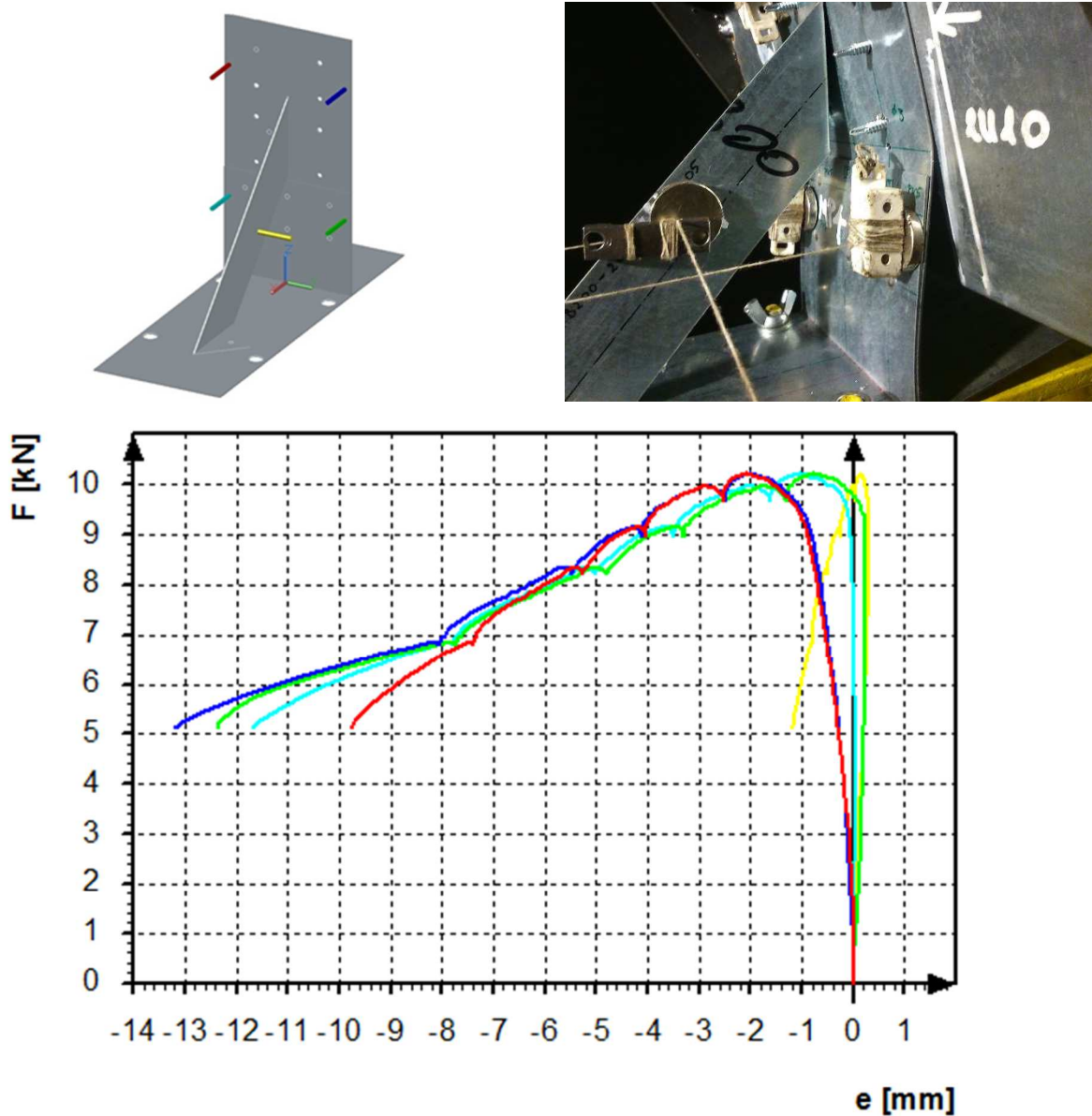
4.1 ábra B200-2L12-1AB12-03 tesztelem sematikus ábrája a tönkremenetel pillanatát és F-e grafikonja (kN-mm)
