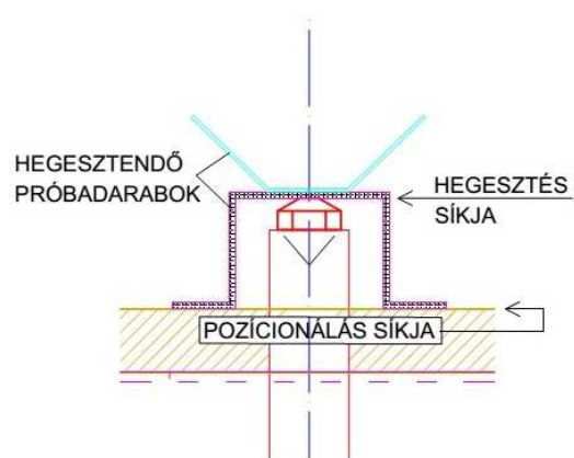
2.5 ábra Munkalap pozíciója a hegesztési síkhoz képest bonyolultabb elemek esetén
