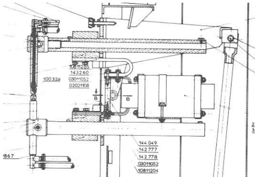
5.1 ábra Ellenállás hegesztő berendezés tervdísz részlete
