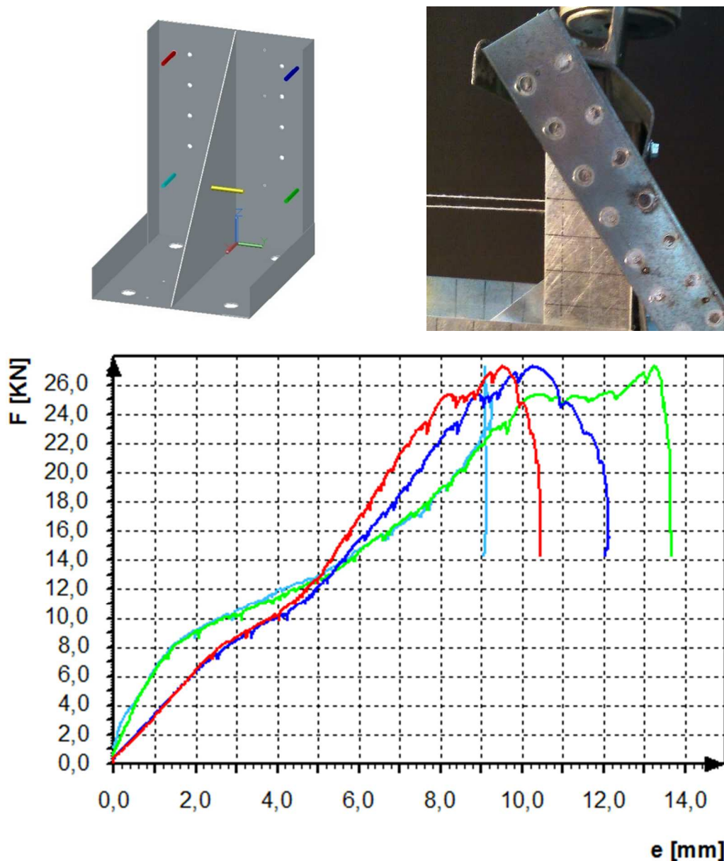
4.8 ábra B200-1U10-1AB10-01 tesztelem sematikus ábrája a tönkremenetel pillanatát és F-e grafikonja (kN-mm)
