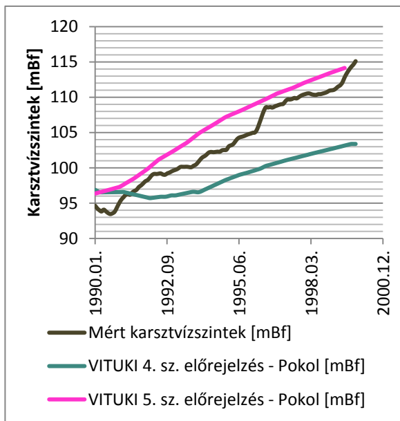
5.11.-5.12. ábra A mért és a VITUKI által előrejelzett karsztvízszintek alakulása a Pokol észlelőkút esetében
