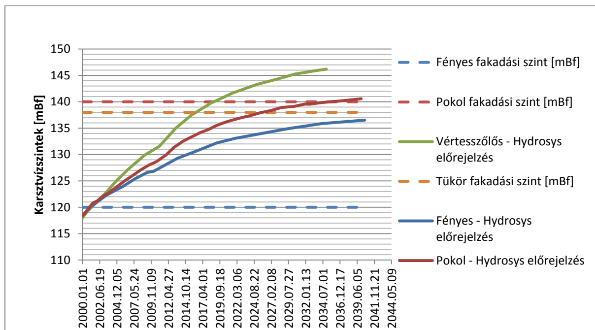
5.1. ábra A Hydrosys Kft. által készített előrejelzés
