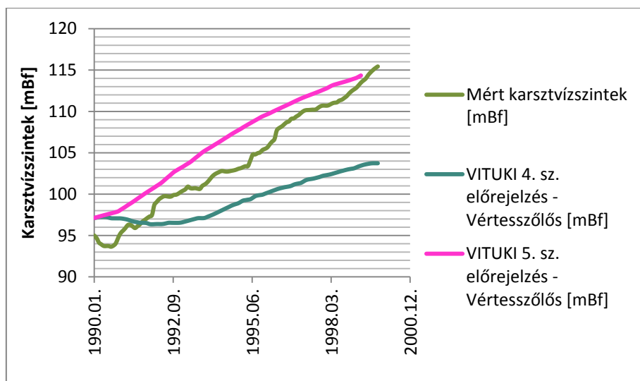
5.24. ábra A mért és a VITUKI által előrejelzett karsztvízszintek alakulása a vértesszőlői észlelőkút esetében
