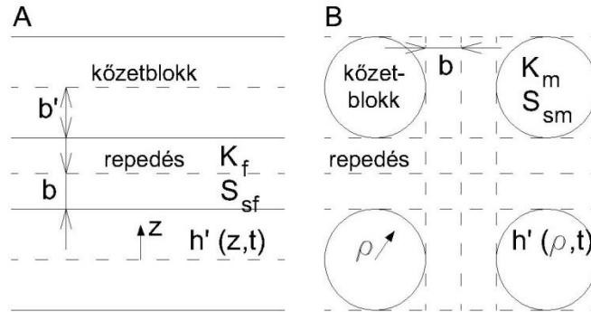
6.4. ábra A Moench módszer lapszerű illetve gömbszerű kőzetblokkjának sematikus ábrája /Moench (1984) nyomán Karay (2012)/
