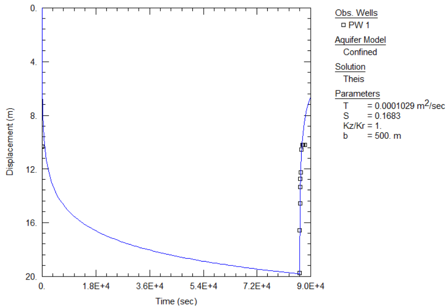
6.8. ábra A TÉ-2 kút szivárgásának meghatározása hagyományos Theis módszerrel
