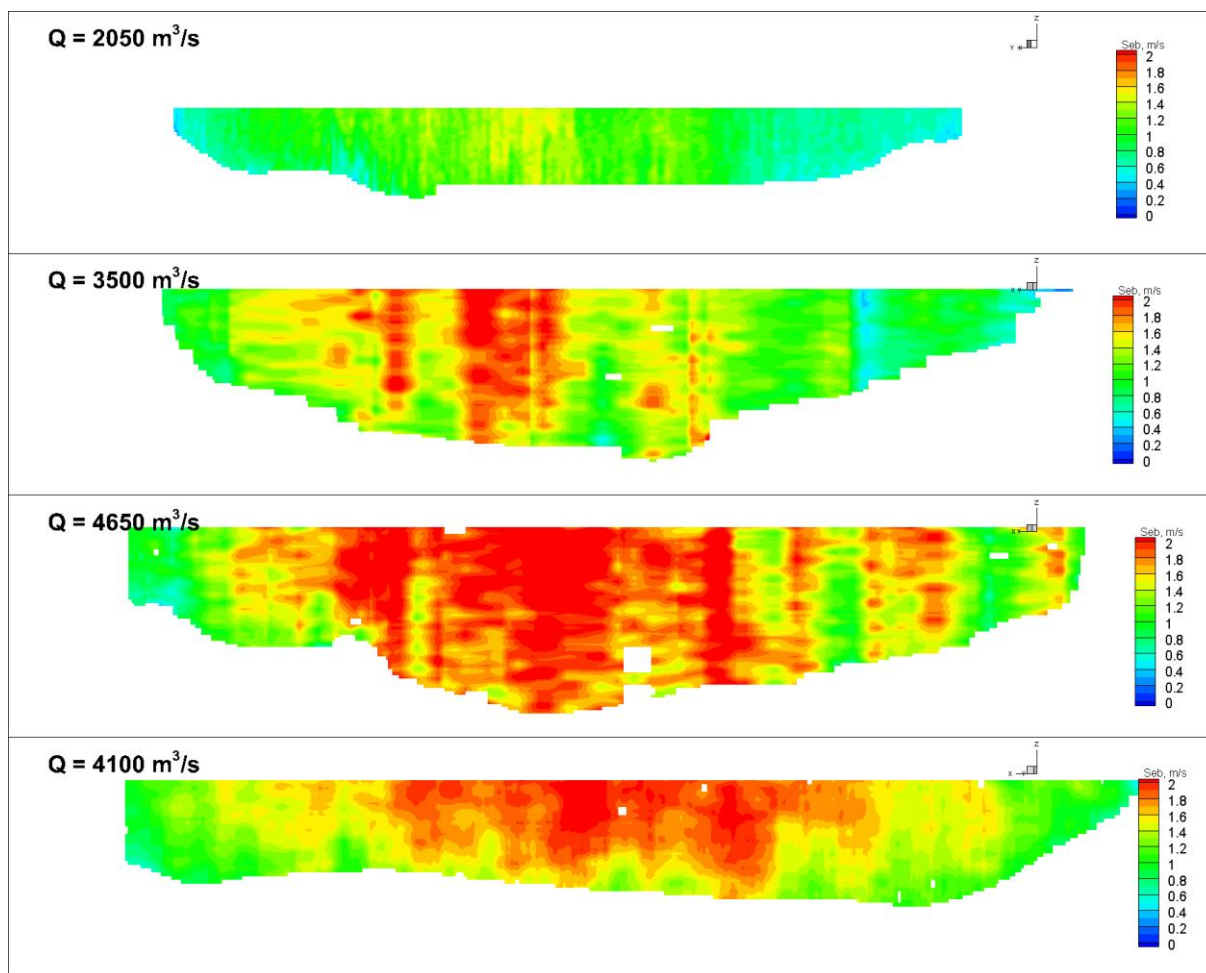
34. ábra: Sebesség eloszlása a keresztaszelvénymentén a négy expedíció során
