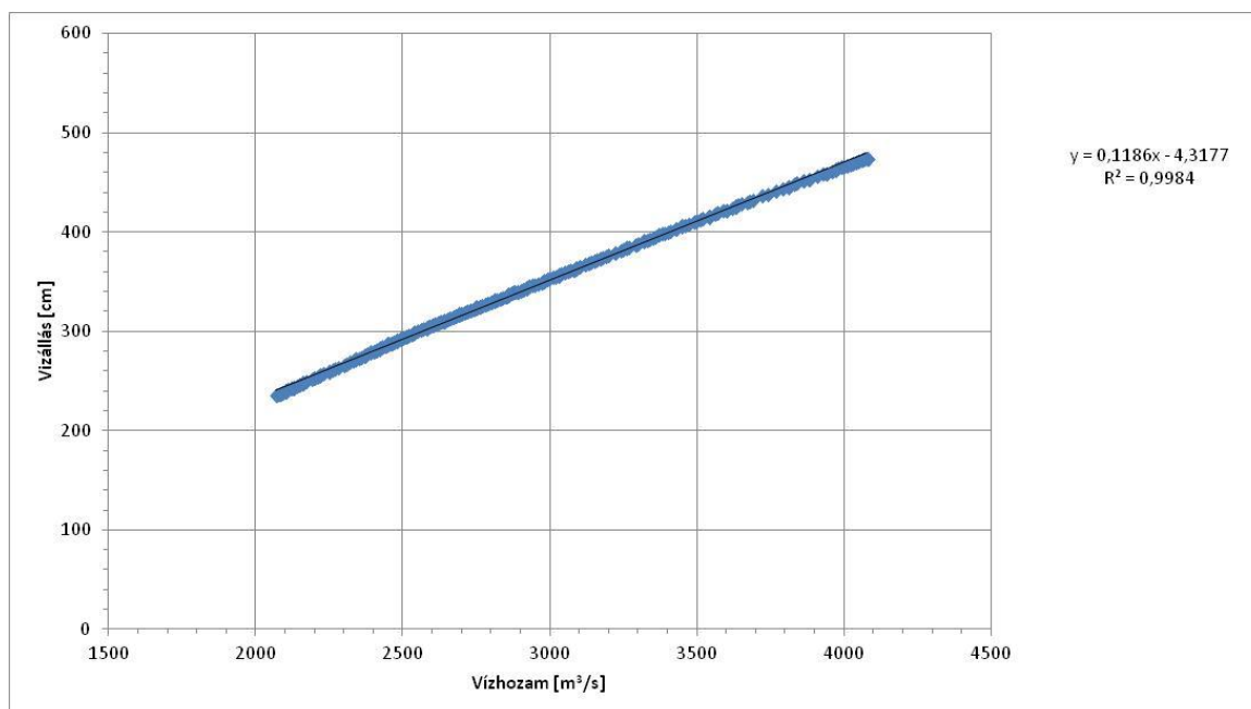
23. ábra: Q-H görbe (Budapest, Duna 1646,5 fkm)
