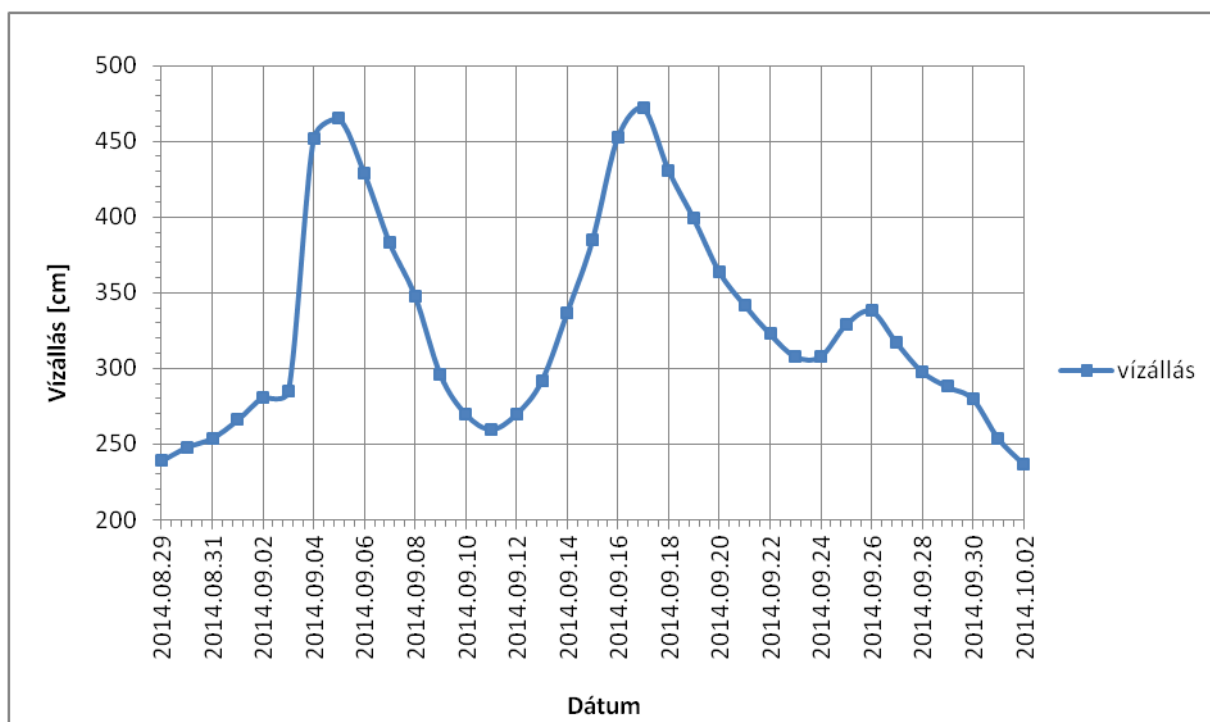
22. ábra: Vízállás idősor a mérési időszakra
