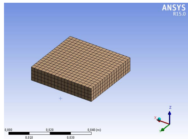
2.10. ábra: Akkumulátoron alkalmazott háló
