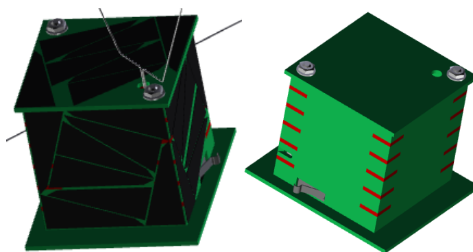
1.4. ábra: Műhold menetes száakkal erősítve, bal oldali a teljes, a jobb oldali a szimulációk során használt, napelemektől és antennáktól egyszerűsített szerkezet
