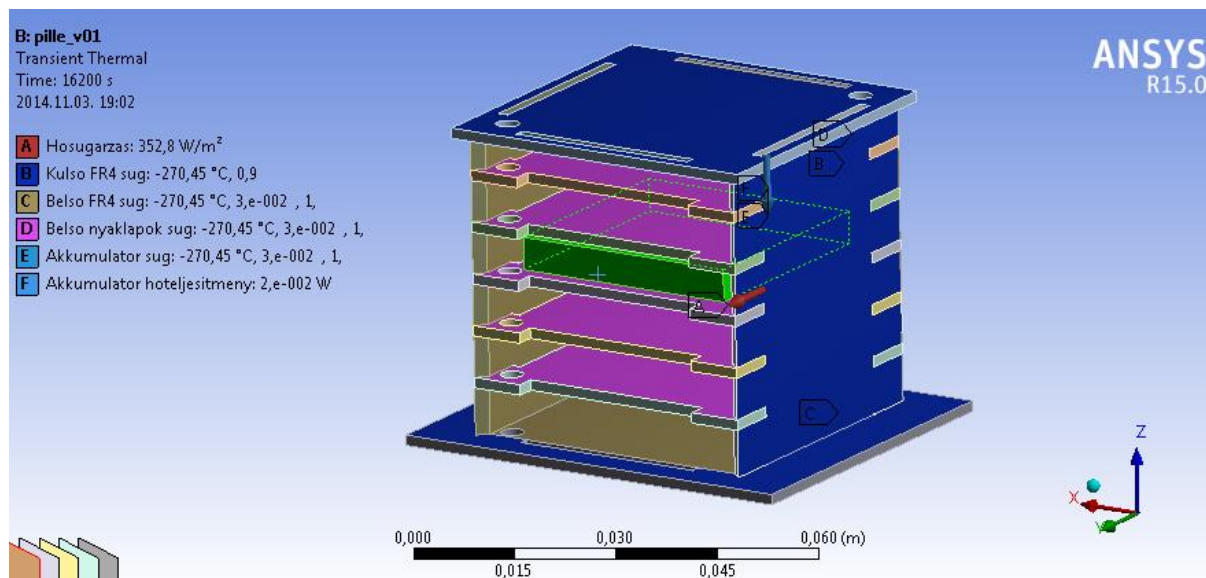
3.9. ábra: Vázszerkezetes konstrukció peremfeltételei
