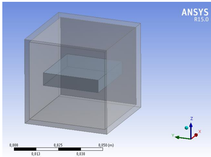
2.8. ábra: Kockahéj és akkumulátor geometriája
