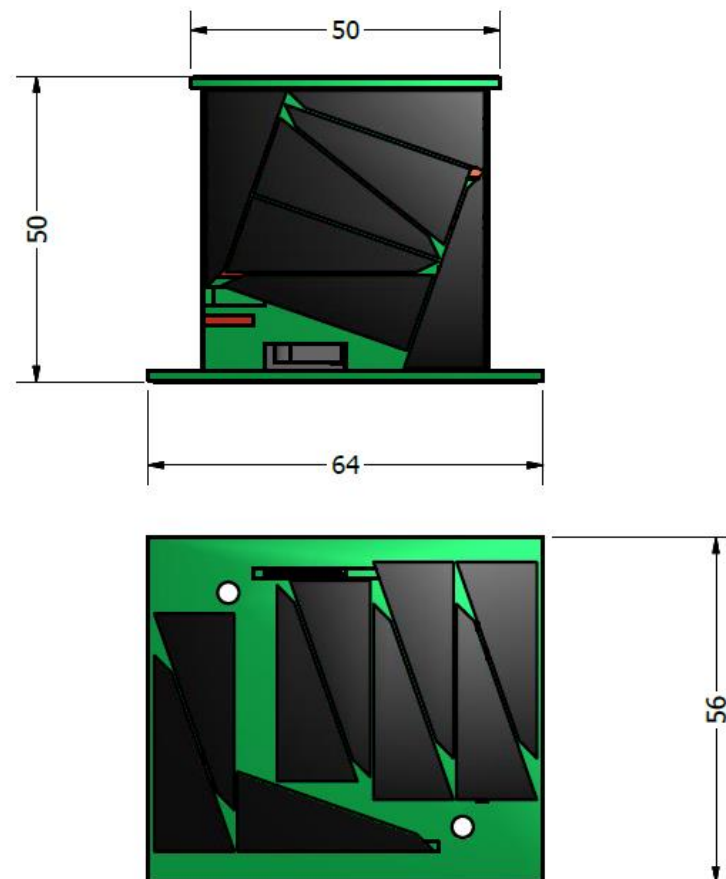
1.2. ábra: Műhold szükséges befoglaló méretei
