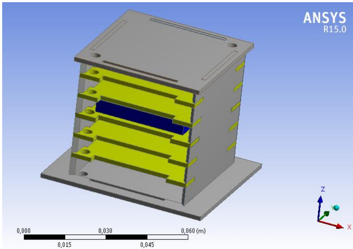
3.7. ábra: Menetes száakkal erősített konstrukció belső elrendezése
