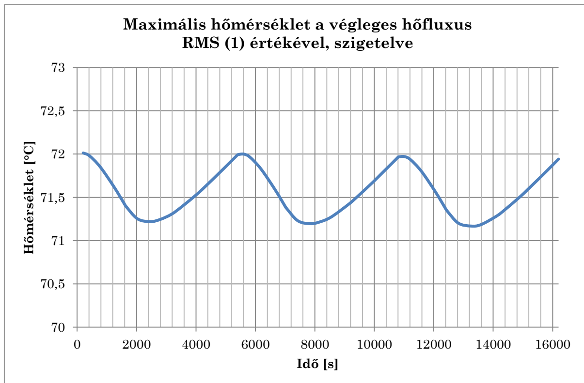
2.14. ábra: A szigetelt, hasznosított hőteljesítmény nélküli hőfluxussal számolt maximális hőmérsékletek az akkumulátoron.
