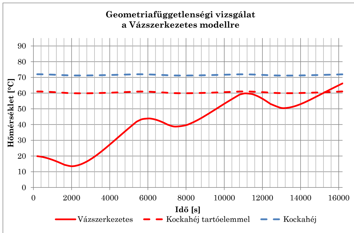
4.2. ábra: Geometriafüggetlenségi vizsgálat
