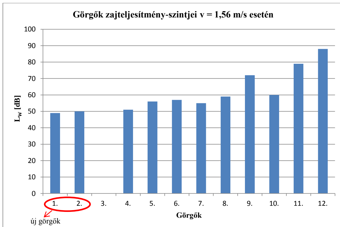
20. ábra: Görgők zajteljesítmény-szintjei 1,56 \frac{m}{s} heveder sebesség esetén
