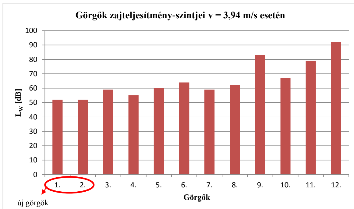
21. ábra: Görgők zajteljesítmény-szintjei 3,94 \frac{\text{m}}{\text{s}} heveder sebesség esetén
