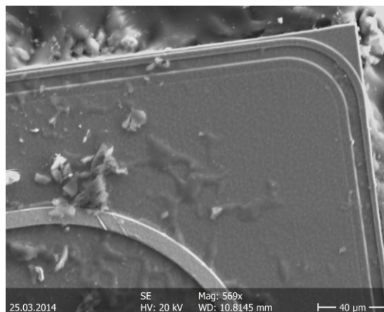
40. ábra: LG LED chip sarok kialakítása (569x-es nagyítás)
