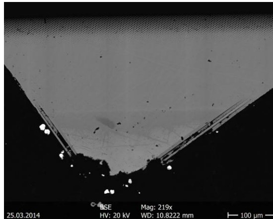
37. ábra: LG Matrix LED, LED chip rétegzettsége (219x-es nagyítás)
