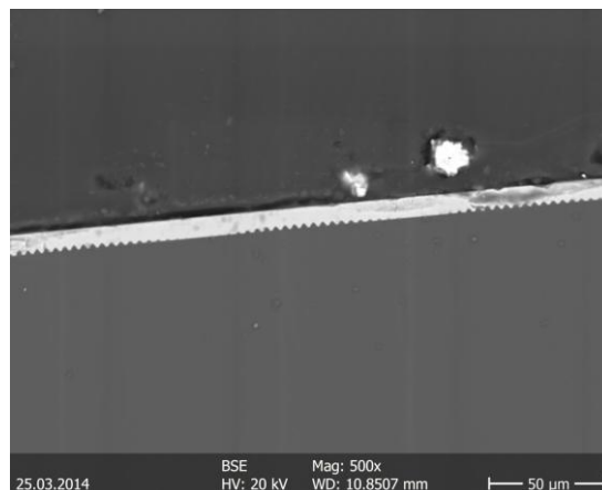
47. ábra: Samsung Mátrix LED Zafír-Gallium réteg csatlakozása (500×-es nagyítás)
