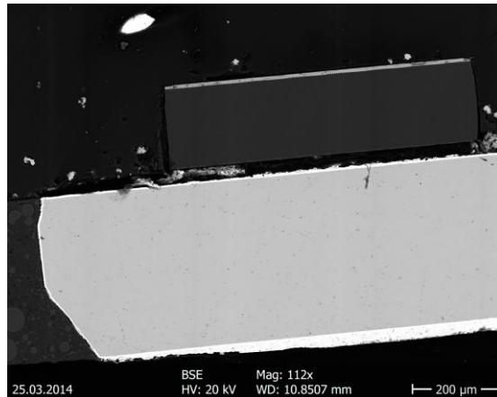
46. ábra: Oldalról csiszolt Samsung Mátrix LED közepén a LED chip alatta a zafír tömb (112x-es nagyítás)
