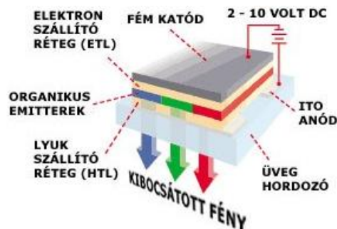
8. ábra: OLED chip szerkezeti felépítése [www.hazi-mozi.hu]
