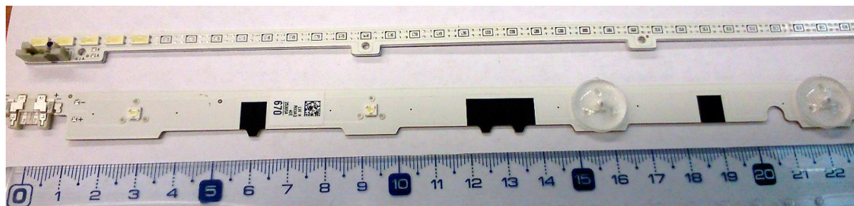
23. ábra: Edge (felső) és Matrix (alsó) típusú LED panel
