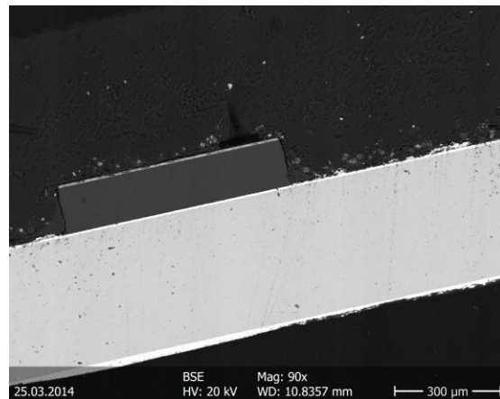
54. ábra: Sony EDGE LED keresztmetszeti csiszolata (90x-es nagyítás)
