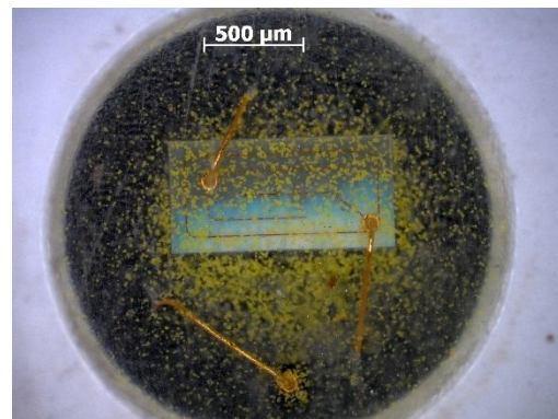
29. ábra: Alulról csiszolt Samsung Mátrix LED felülről fotózva 5x-ös nagyítás
