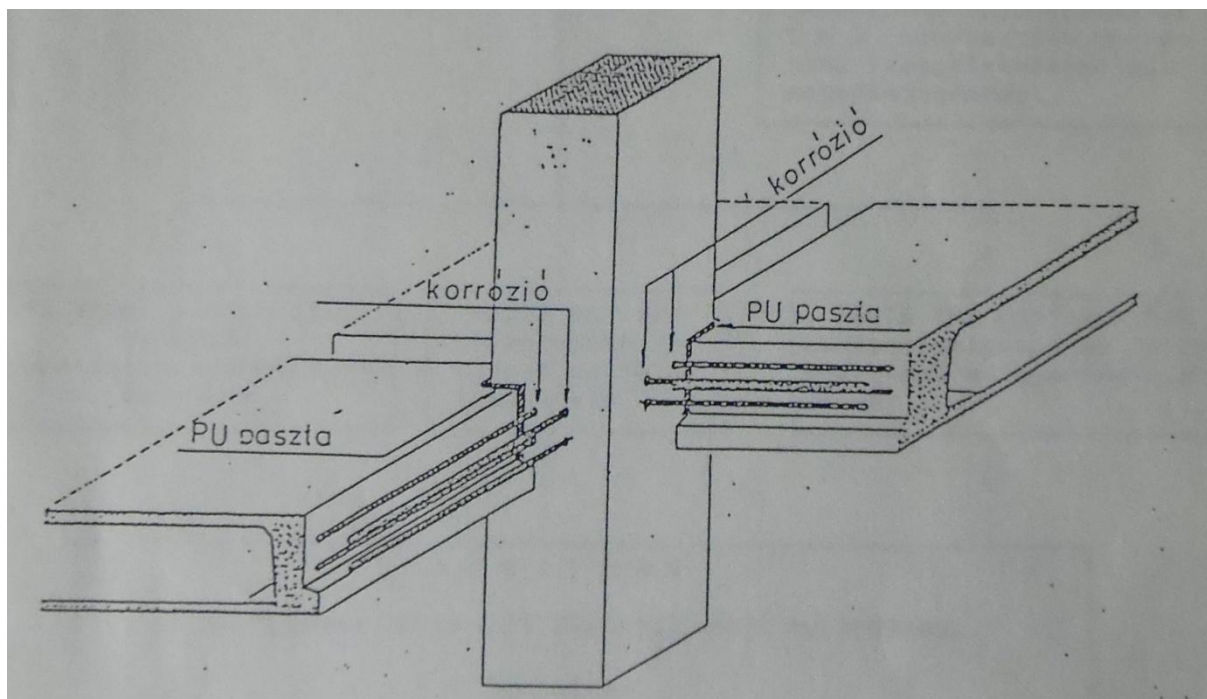
21. számú kép: PU- paszta által okozott korrózió
