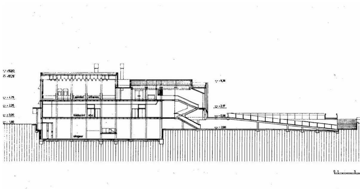
17. számú kép: ABC- áruház és étterem oldalrajz)
