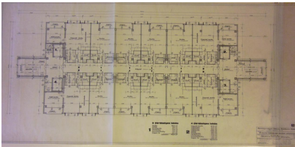
12. számú kép: 25 emeletes épület, általános emeleti rajz
