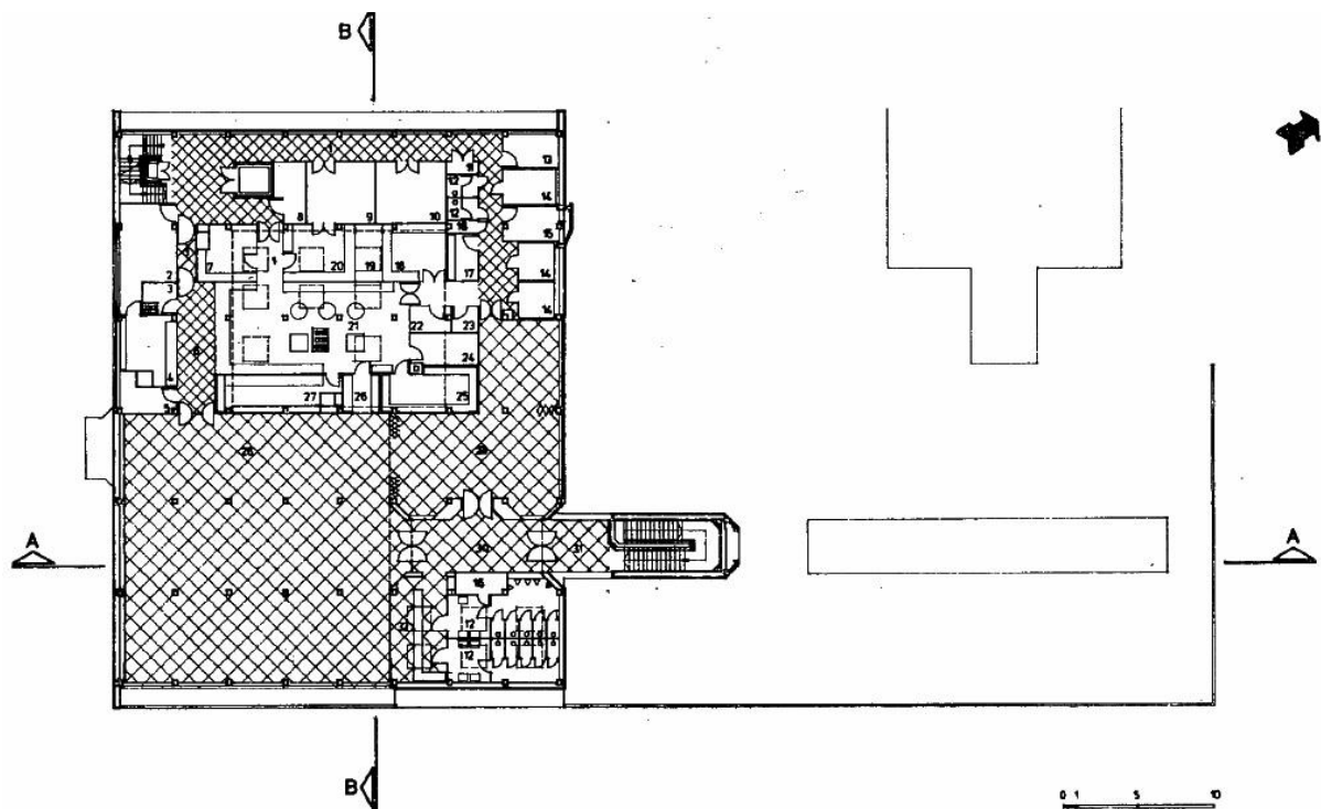
16. számú kép: étterem (első emeleti alaprajz)
