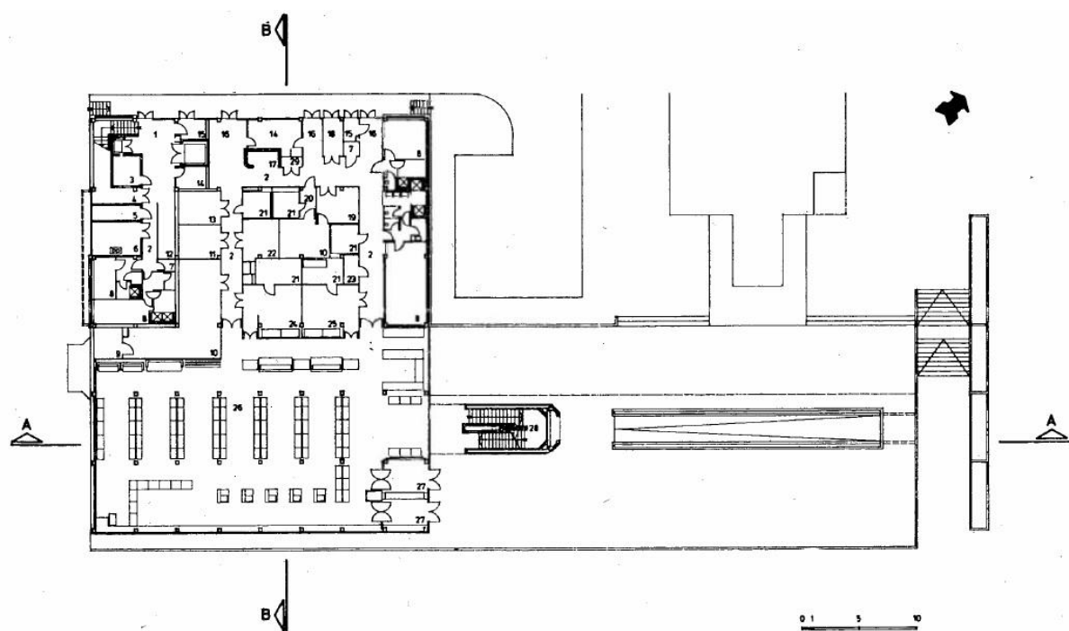
15. számú kép: ABC- áruház (földszinti alaprajz)
