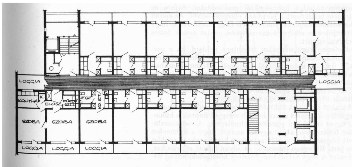
7. számú kép: Szigeti városrész 22 emeletes épület alaprajz
