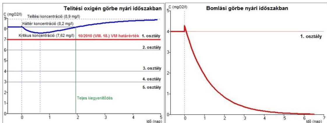
33. ábra Az oxigénvonal és a szerves anyag tartalom görbéjének alakulása nyáron [saját vizsgálat]
