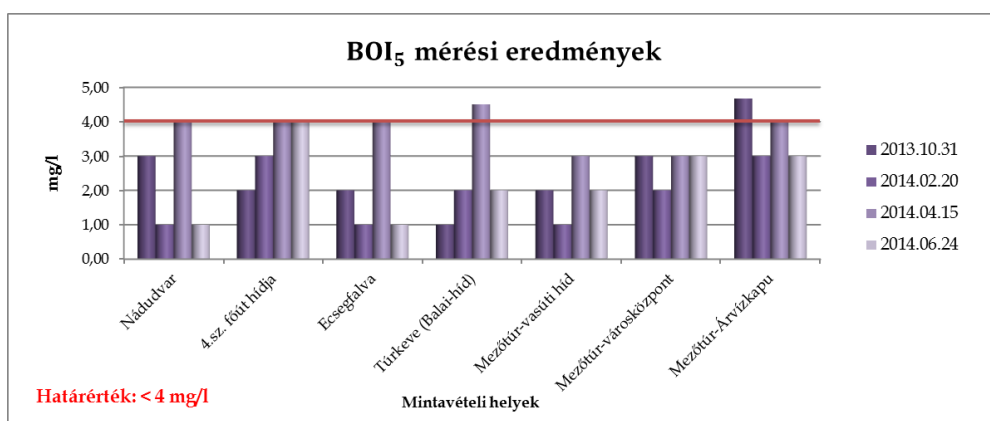
26. ábra Biológiai oxigénigény ( BOI_5 ) koncentráció értékek a mintavételi pontokon
