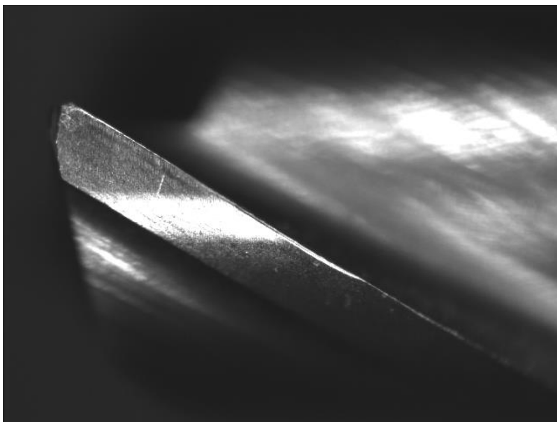
C45 acél -30%, palástél hátkopása
