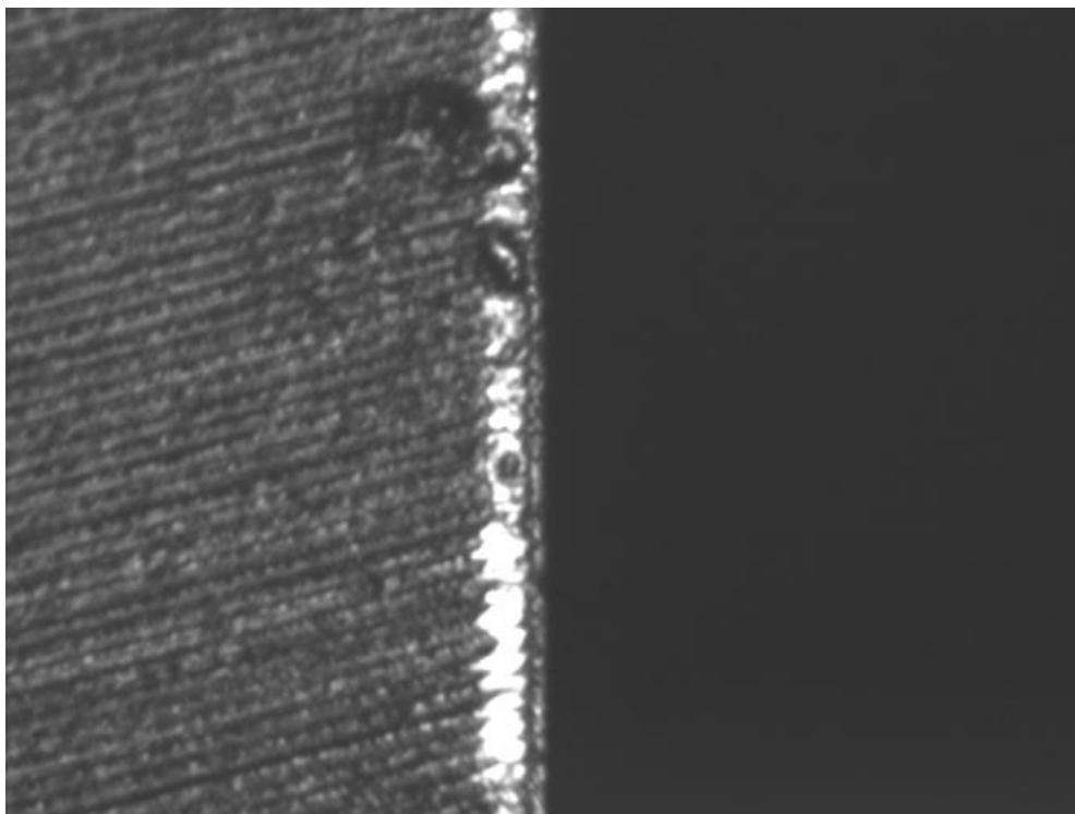
C45 acél +13%, homlokél hátkopása
