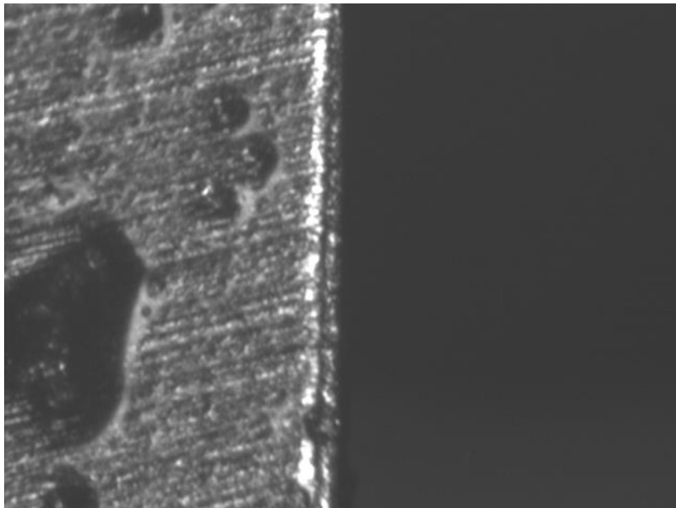
Automata acél -30%, homlokél hátkopása
