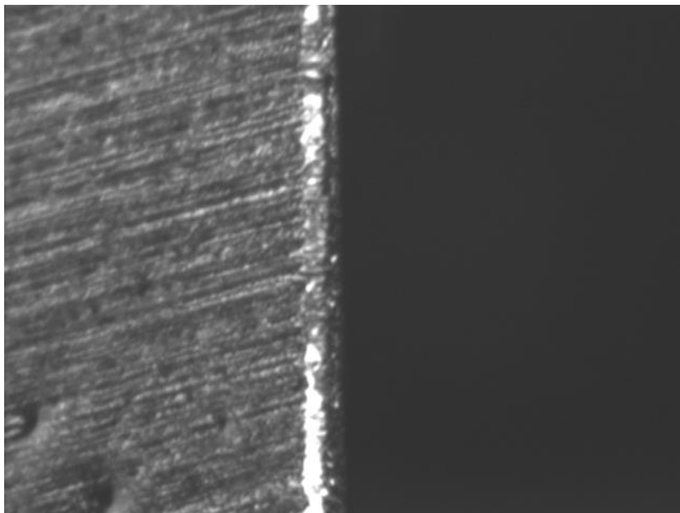
Automata acél +13%, homlokél hátkopása
