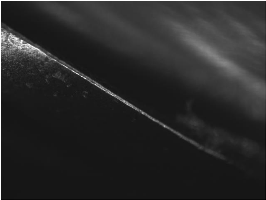
C45 acél optimális, palástél hátkopása
