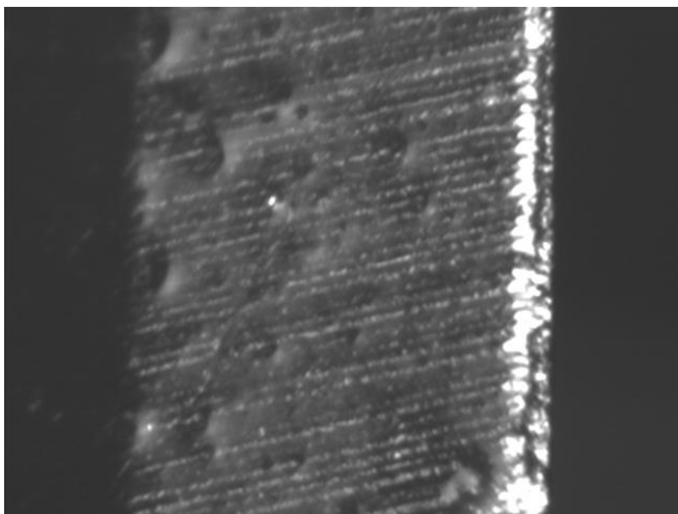
C45 acél -30%, homlokél hátkopása
