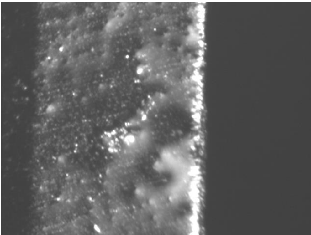
Automata optimális, homlokél hátkopása
