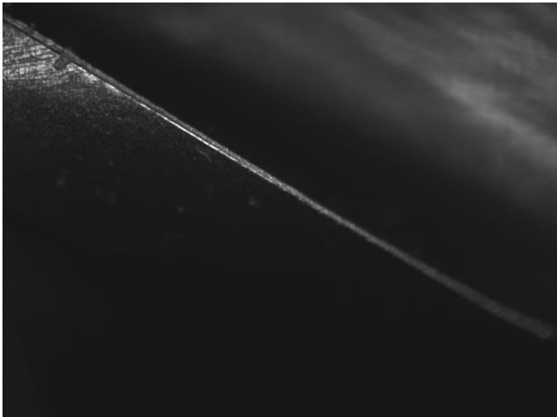
C45 acél +13%, palástél hátkopása
