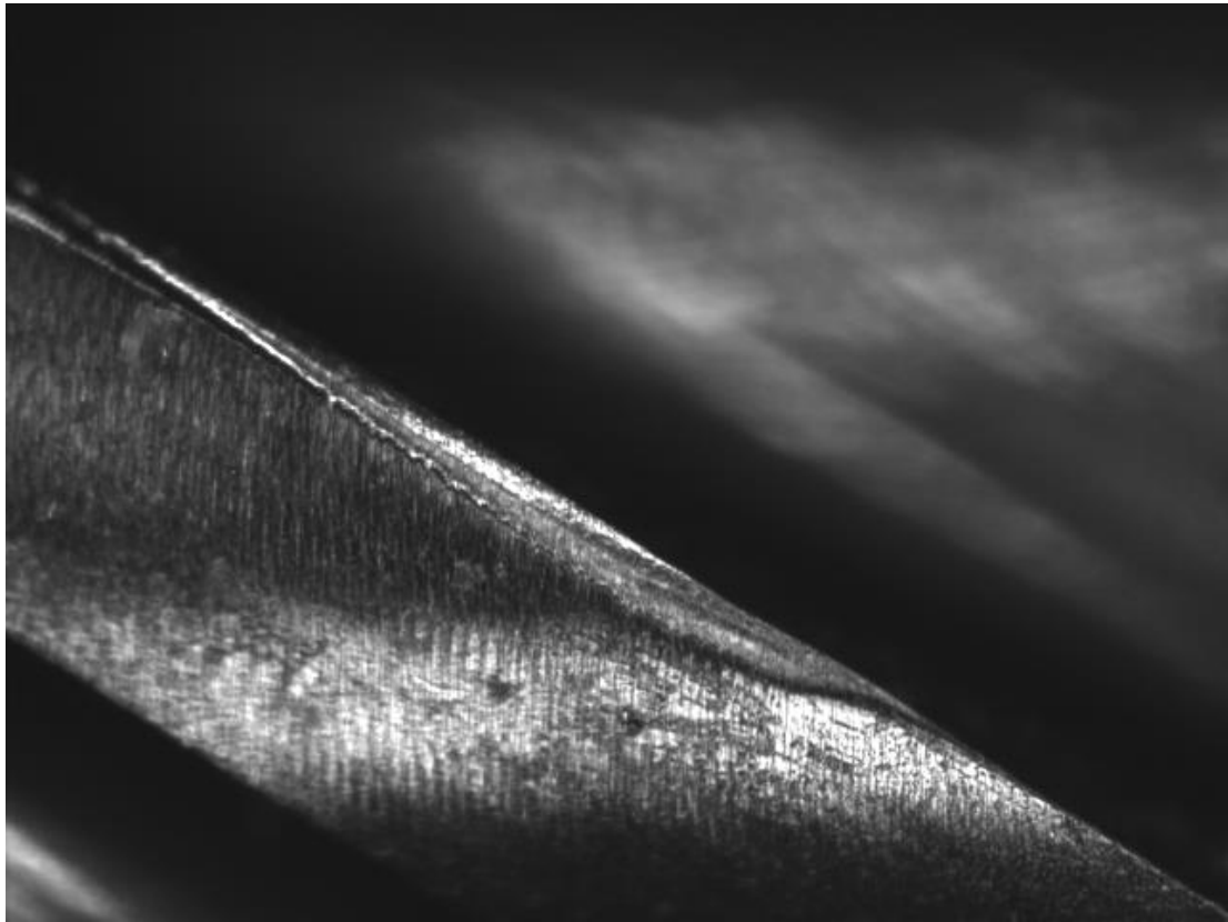
Régi technológia C45 acél esetén, palástél hátkopása
