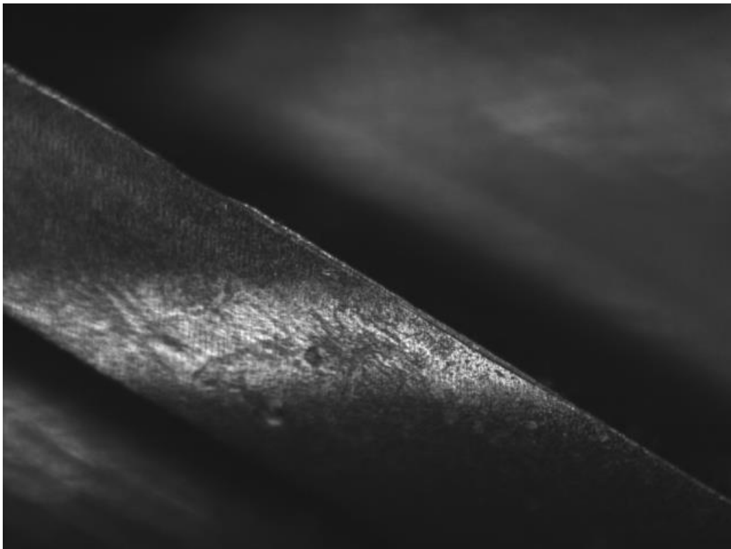
Automata optimális, palástél hátkopása
