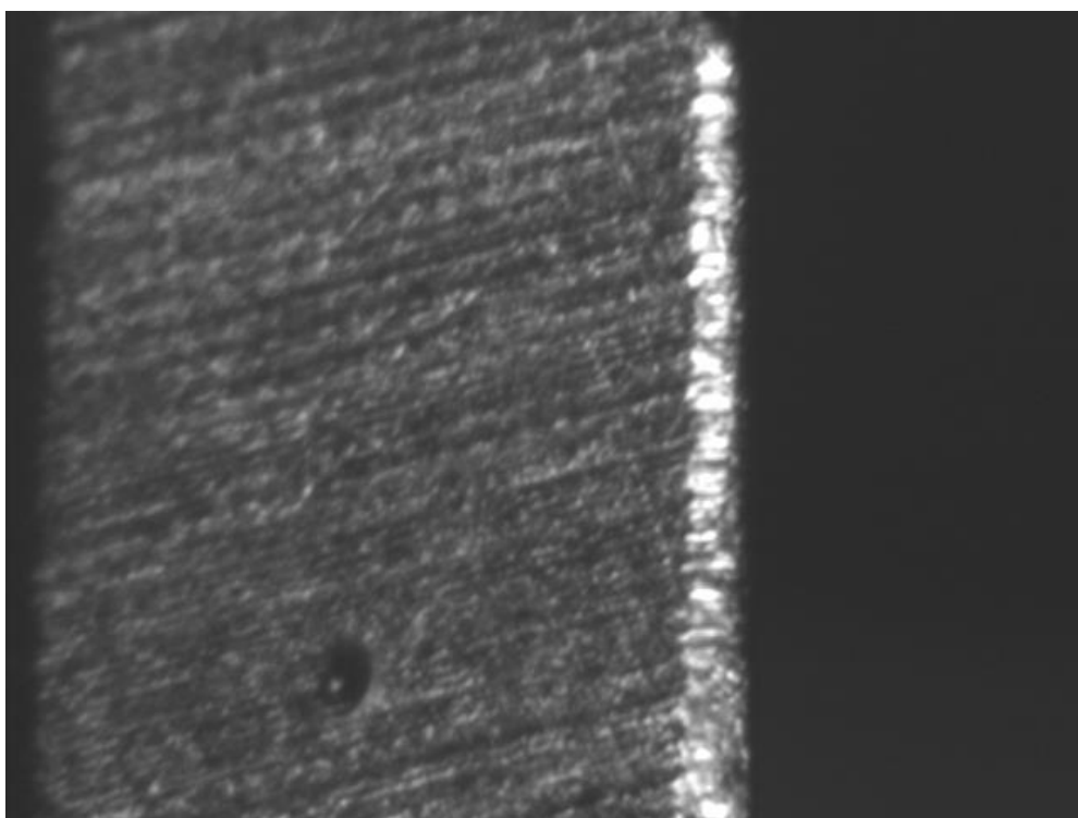
C45 acél optimális, homlokél hátkopása
