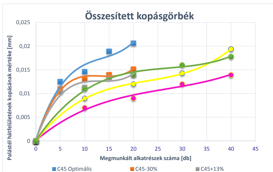
43. ábra. Palástél hátfelületének kopásgörbéi
