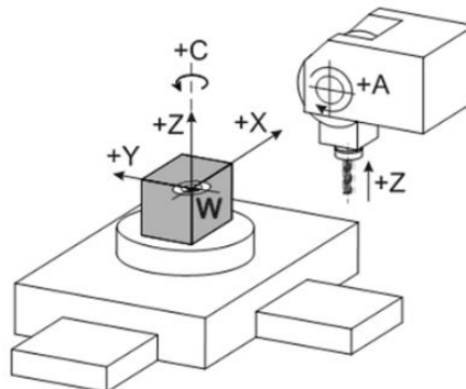
18. ábra. Megmunkáló központ tengelyeinek értelmezése (forrás: Dr. Boza Pál CNC-technológia és – programozás)
