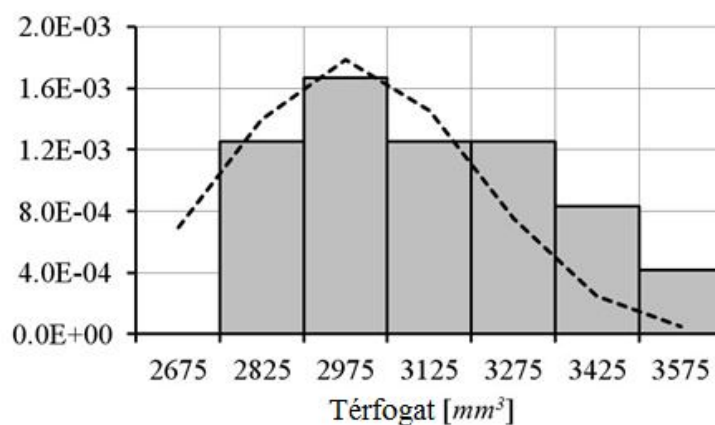
28. ábra A próbatestek térfogatainak, sűrűség histogramja [Forrás: saját készítés]
