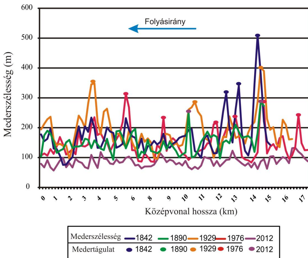
14. ábra: A folyószakasz szélességviszonyainak változása különböző időpontokban
