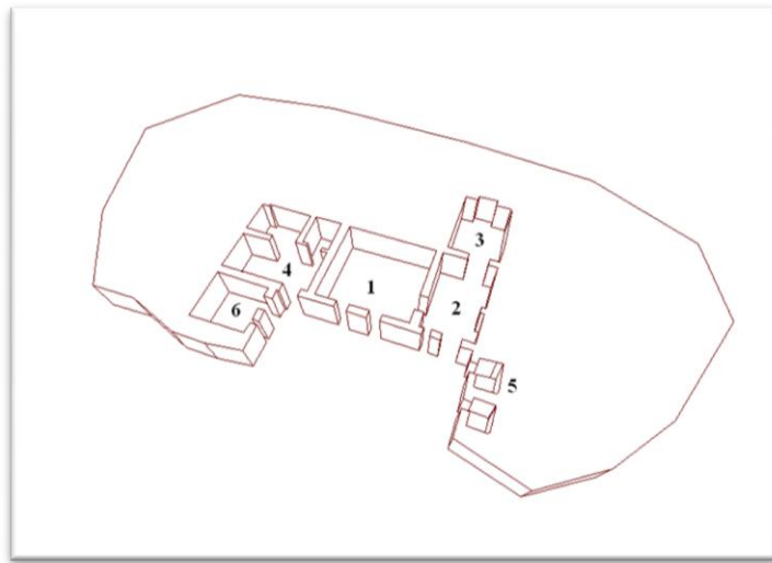
3. Barlanglakás alaprajz rekonstrukció Mednyánszky Miklós építészeti felméréséből (2009)
