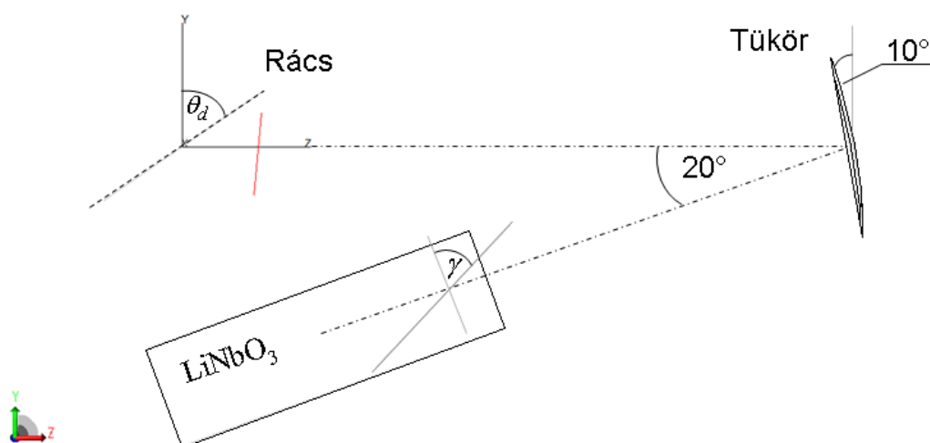
5. ábra: Az egy tükört tartalmazó elrendezés TracePro-ban
