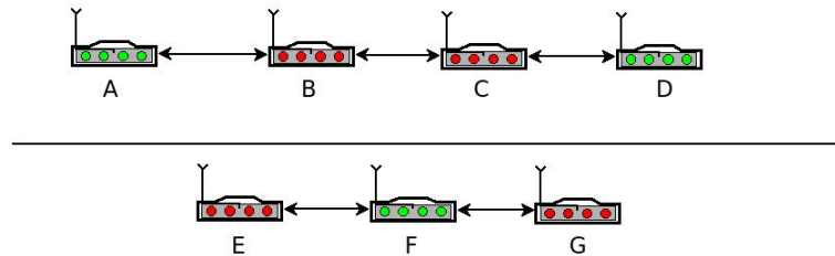
17. ábra: Rejtett csomópontok problémája.[31] A B csomópont A-nak, a C csomópont pedig D-nek akar küldeni. Bár B és C szomszédok, egymás akadályoztatása nélkül képesek küldeni. E és G csomópontok egyaránt F-nek akarnak üzenni. Bár nem szomszédok, interferenciát okoznak egymásnak.
