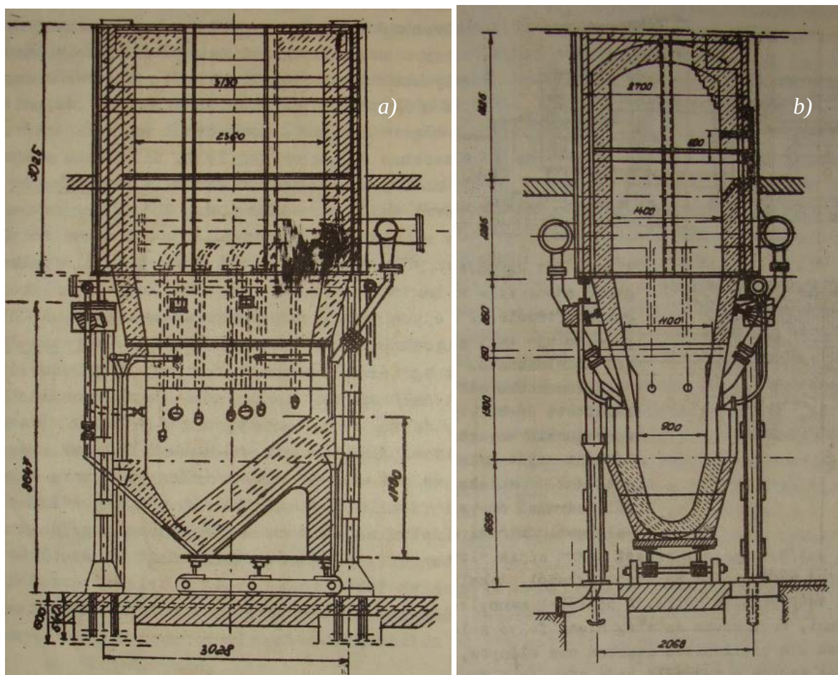
9. ábra Rachette típusú aknákemence (a), és a hagyományos körkeresztmetszetű aknákemence (b) [9].
