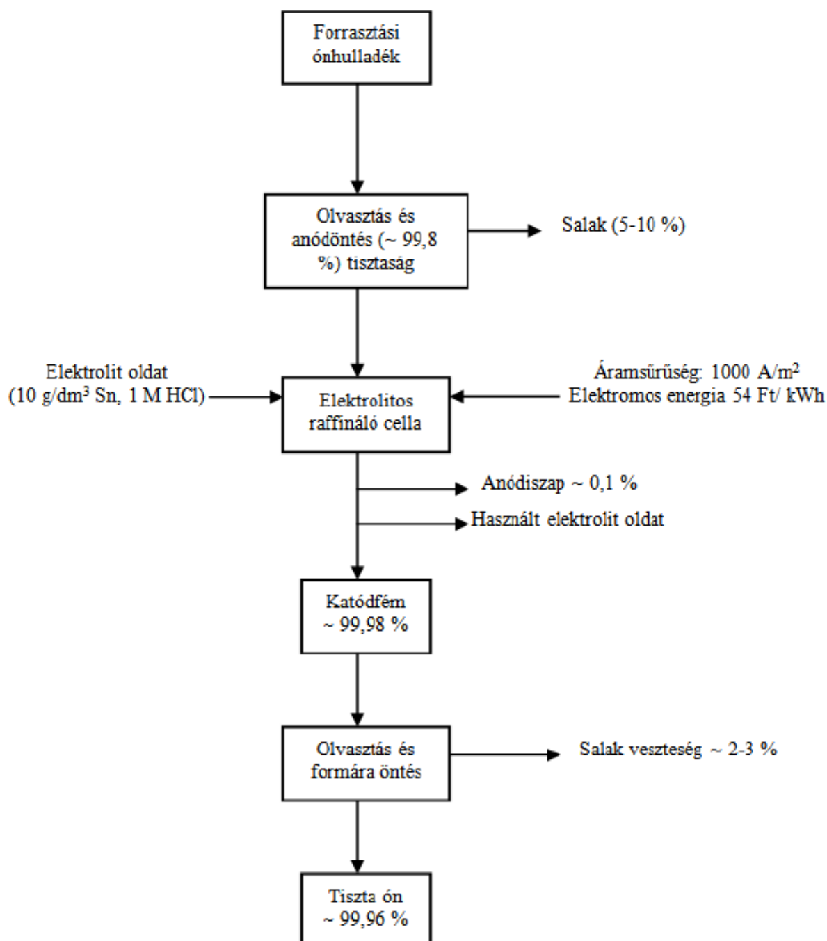
3. ábra Forrasztási ónhulladék feldolgozására kialakított eljárás [3].
