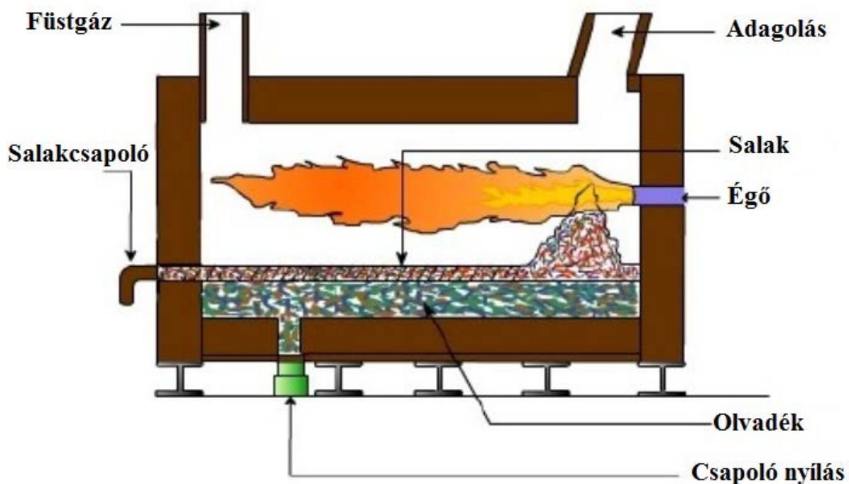
10. ábra Ón ércek redukálására használt lángkemence [10].
