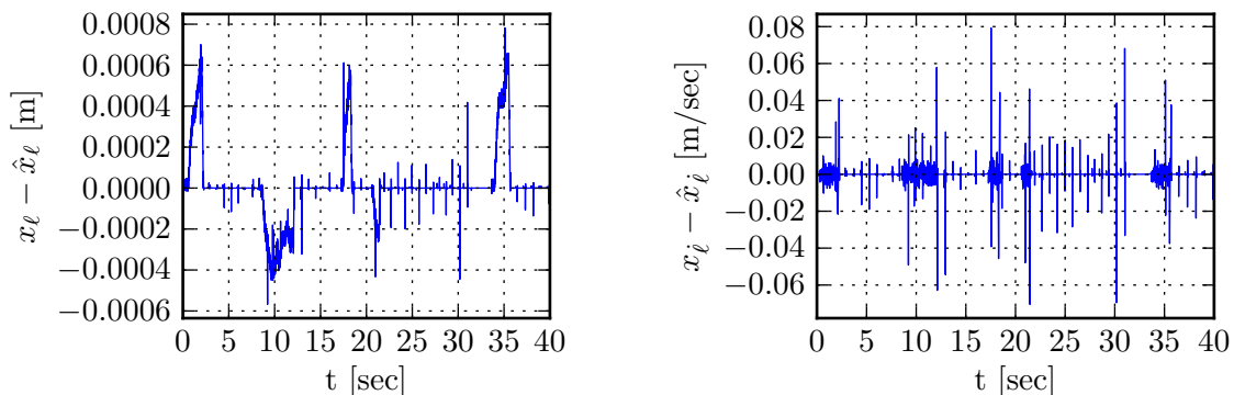
21. ábra. A kocsi pozíciójának és sebességének becslési hibája UKF alkalmazása esetén.
