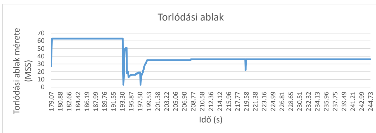
29. ábra: Torlódási ablak teljes törlés mellett
