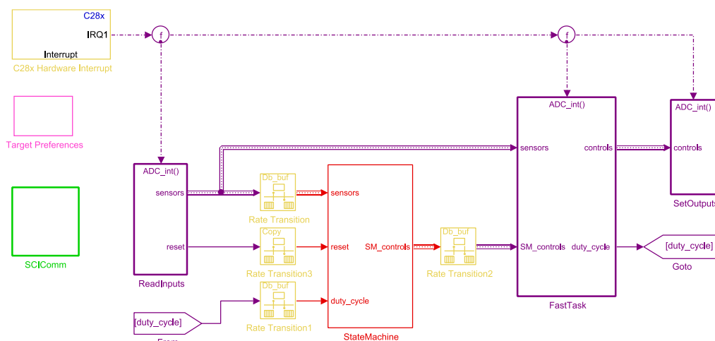
3.1.2 ábra: A vezérlőegység felső szintű Simulink modellje
