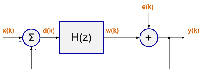
2.2.2 ábra: \Sigma/\Delta modulátor lineáris modellje
