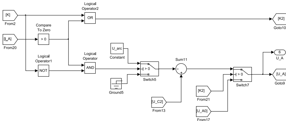
3.3.12 ábra: Az u_A változó számítása
