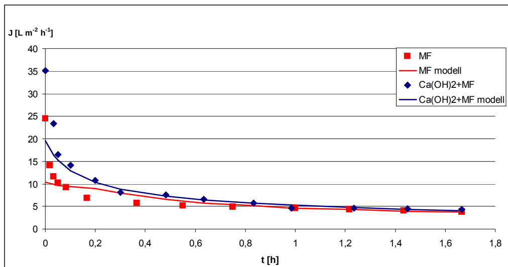
18. ábra: Kezeletlen és \text{Ca(OH)}_2 -dal kezelt szennyvíz szűrhetőségének összehasonlítása (MF – mikroszűrés)
