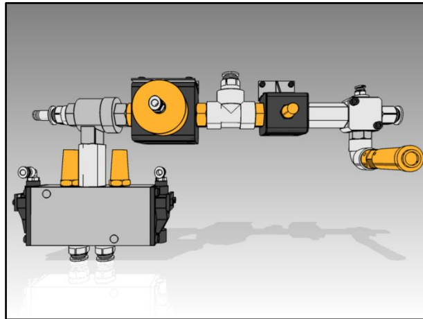
10. ábra A pneumatikus kapcsolás főága.
