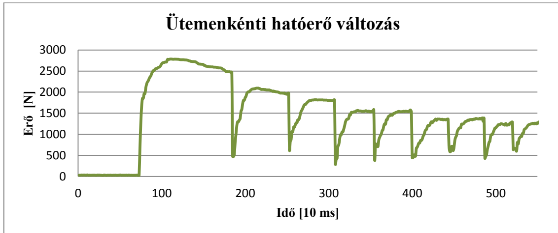
27. ábra Ütemenkénti hatóerő
