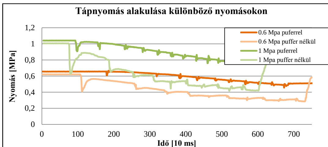
24. ábra Tápnymás alakulása különböző nyomásokon
