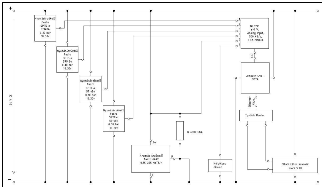
32. ábra Telemetria mérőkapcsolás
