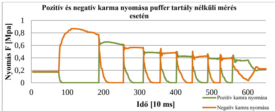
26. ábra Pozitív és negatív kamra nyomása puffer tartály nélküli mérés esetén
