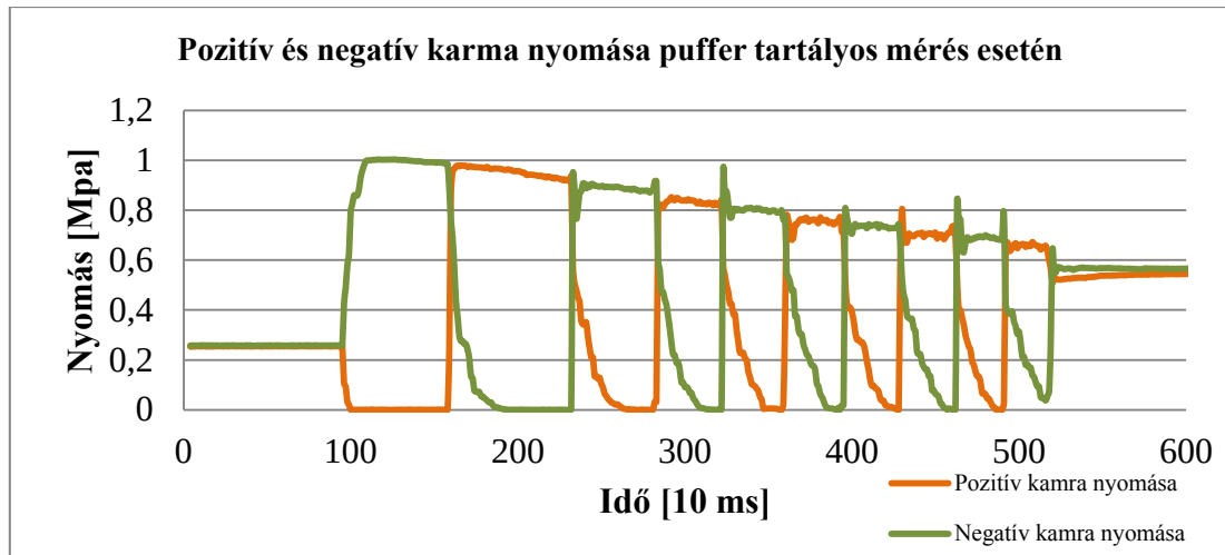
25. ábra Pozitív és negatív kamrák nyomása Puffer tartályos mérés esetén
