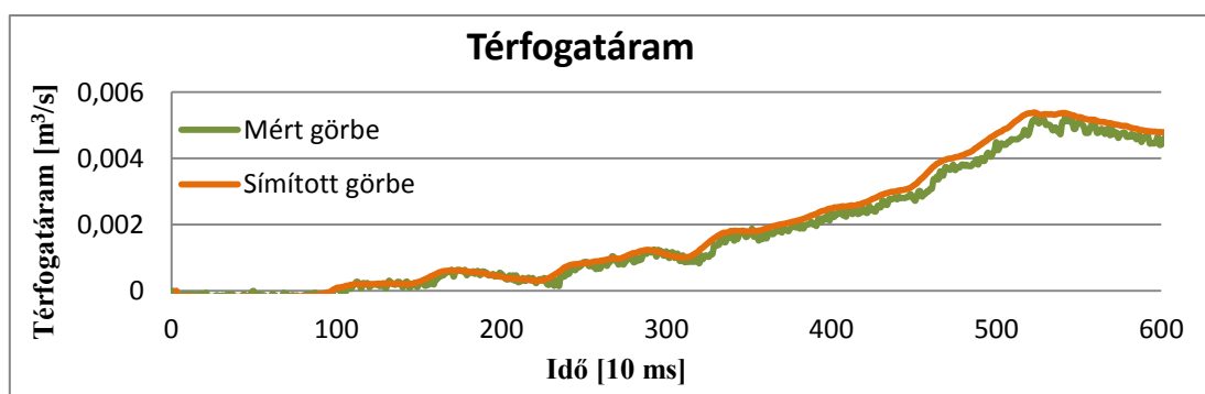
22. ábra Térfogatáram simítása
