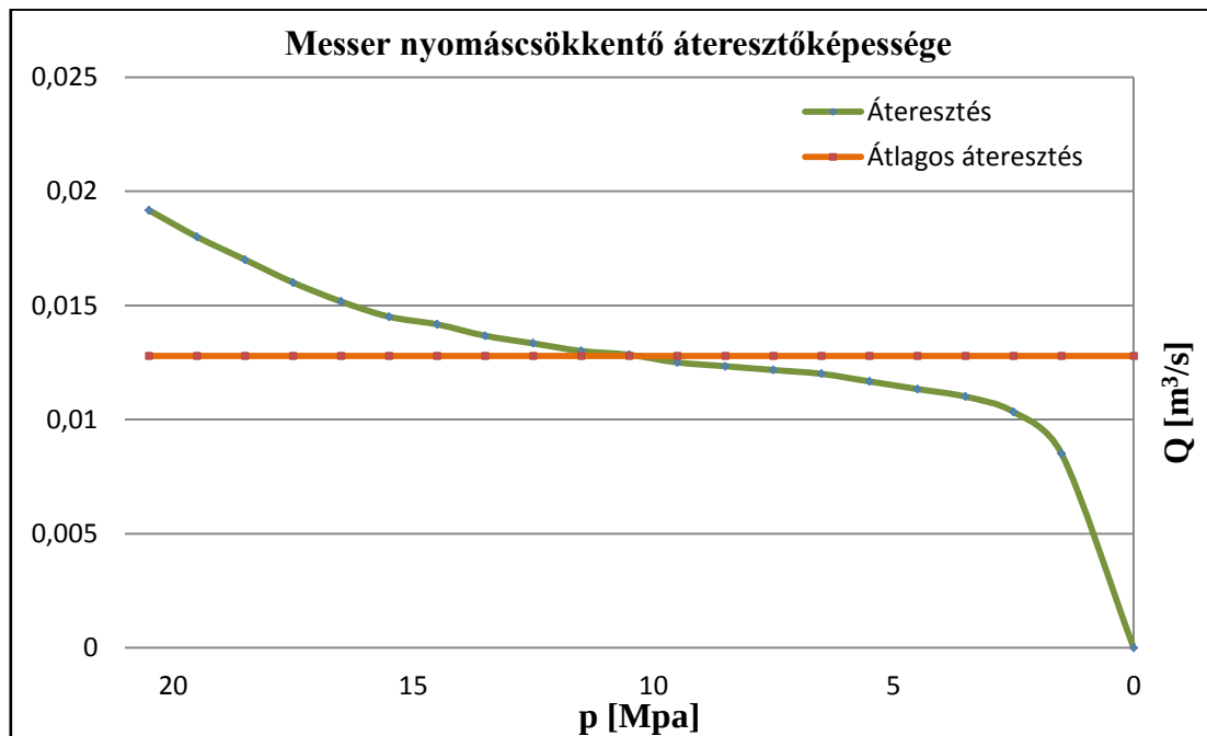
9. ábra Messer Constant 2000 nyomáscsökkentő áteresztési görbéje
