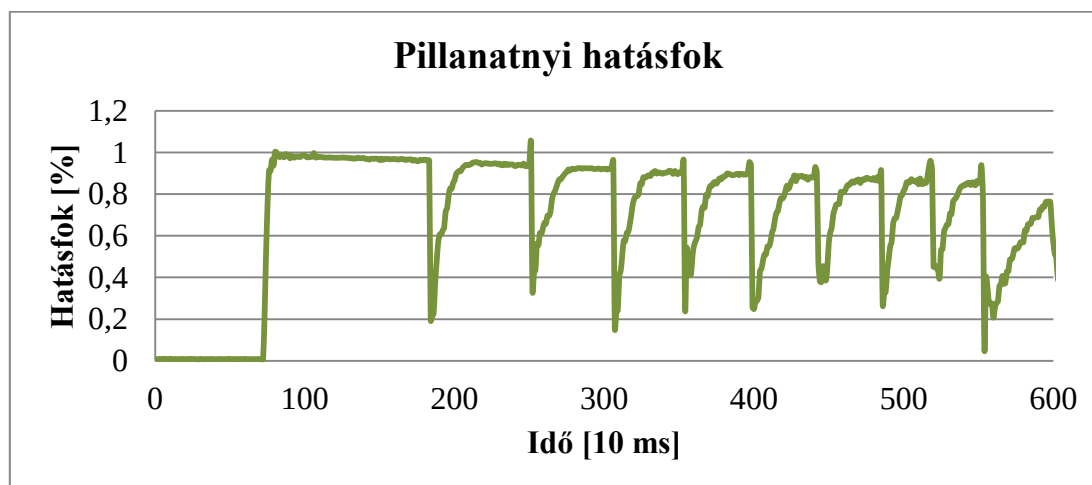
30. ábra 1 MPa-os mérés Pillanatnyi hatásfok görbéje
