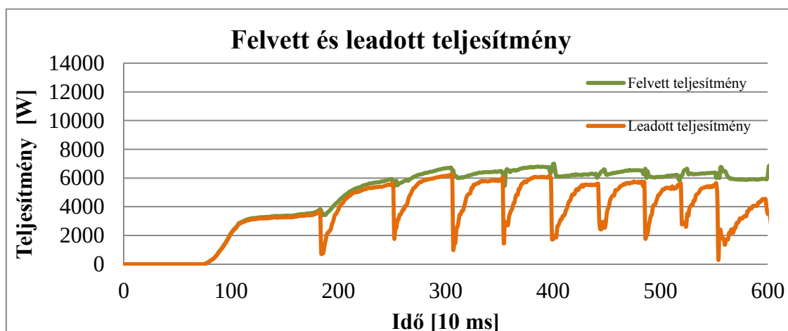
29. ábra 1 MPa-os mérés felvett és leadott teljesítménye
