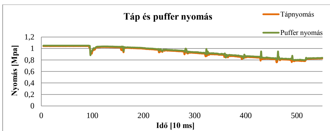
23. ábra 1 MPa értékű mérés táp és puffer nyomás görbéje
