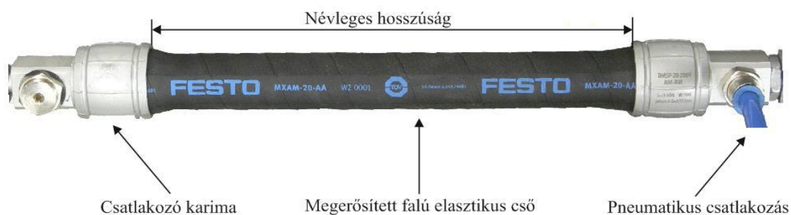
6. ábra A pneumatikus mesterséges izom felépítése (DMSP).
