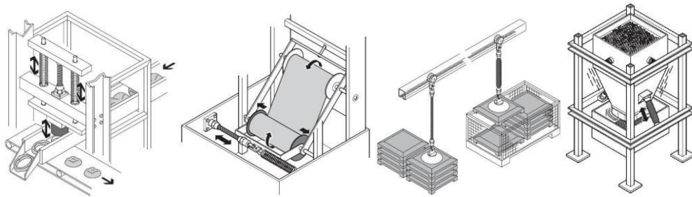
4. ábra Fluidic Muscle-ok ipari alkalmazása (balról): lyukasztógép, tekercselőgép, emelőszerkezet, vibrációs tölcser
