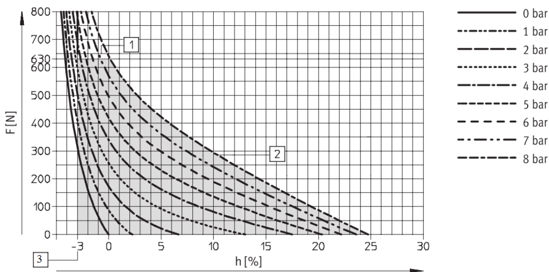
20. ábra MAS-10-100 jelölésű, Festo által gyártott Fluidic Muscle jelleggörbéje
