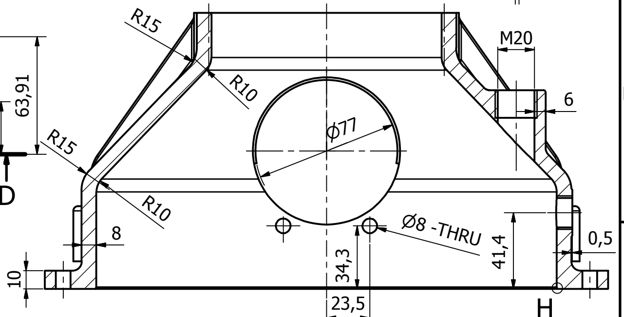
F-F (1 : 2)
