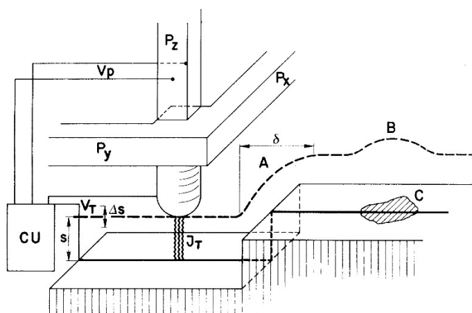
10. ábra. Az STM működésének alapjai[27]
